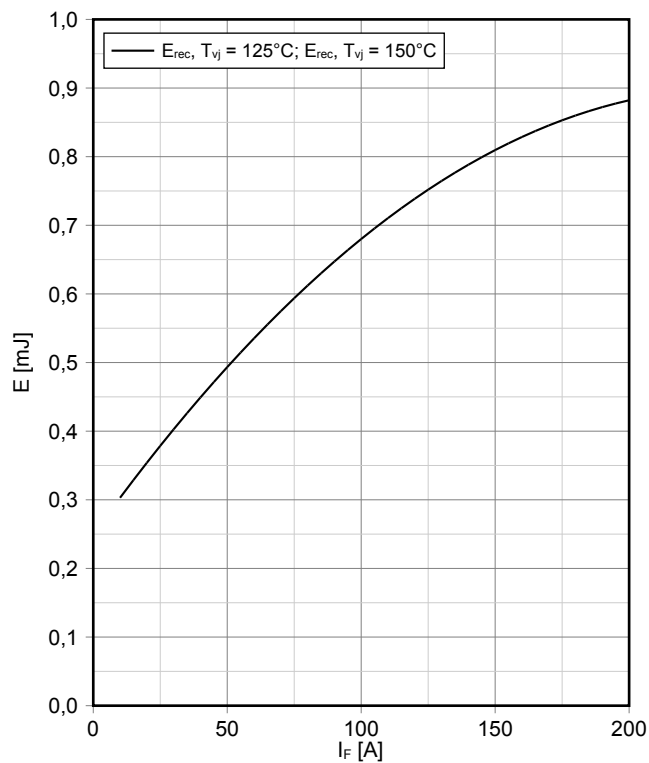
スイッチング損失 ダイオード, D5-D6 (Typical) switching losses Diode, D5-D6 (typical) E_{rec} = f(I_F) R_{Gon} = 5 \Omega , V_{CE} = 500 V
