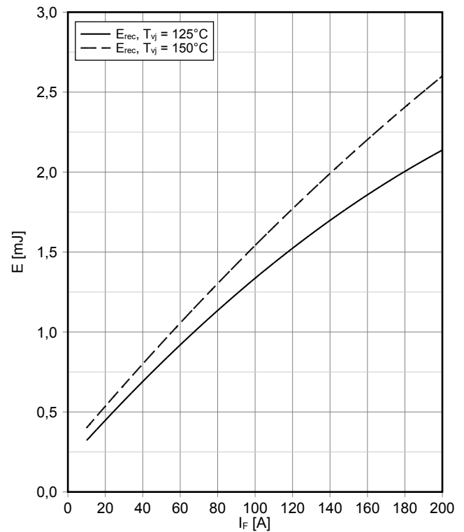
开关损耗 二极管, D1 / D4 (典型) switching losses Diode, D1 / D4 (typical)
