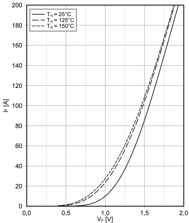
正向偏压特性 二极管, D1 / D4 (典型) forward characteristic of Diode, D1 / D4 (typical)
