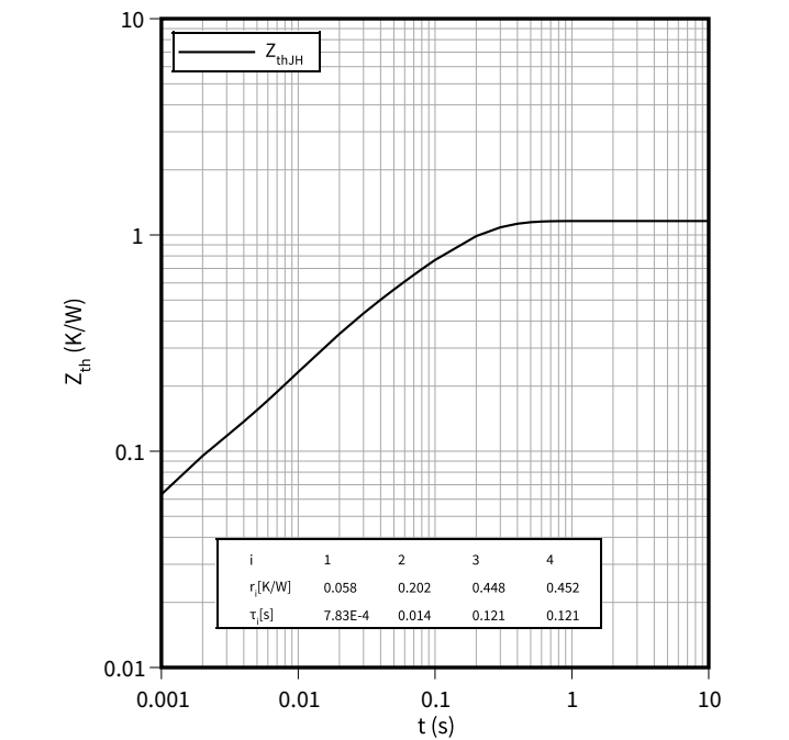
過渡熱インピーダンス, 逆極性保護 diode Z_{th} = f(t)
