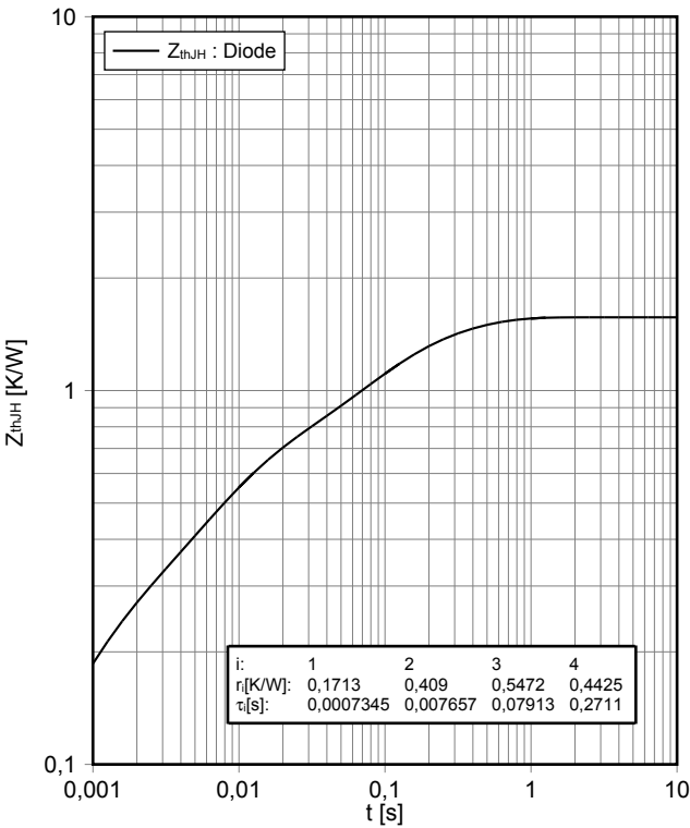
過渡熱インピーダンス Diode-、チョッパ transient thermal impedance Diode-Chopper Z_{thJH} = f(t)
