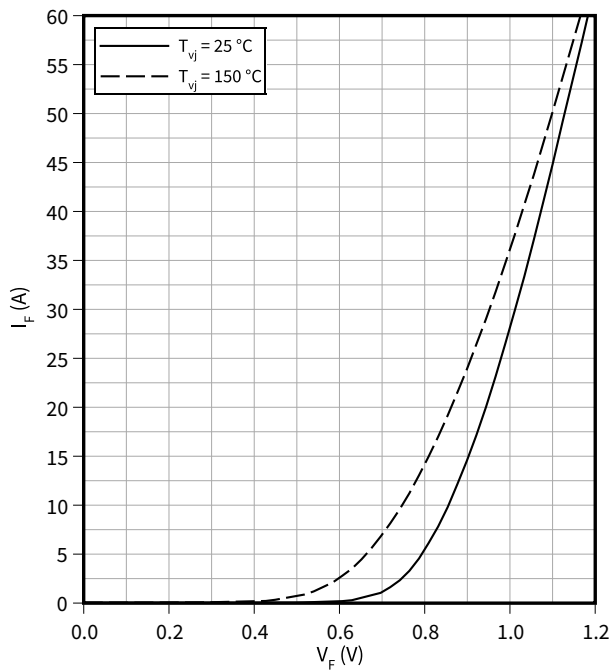
順電圧特性 (typical), 逆極性保護 diode
