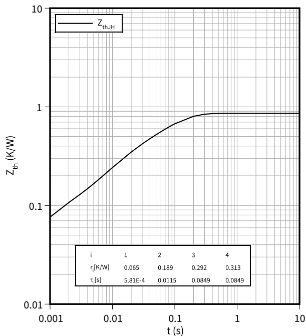
過渡熱インピーダンス, 逆極性保護 diode
