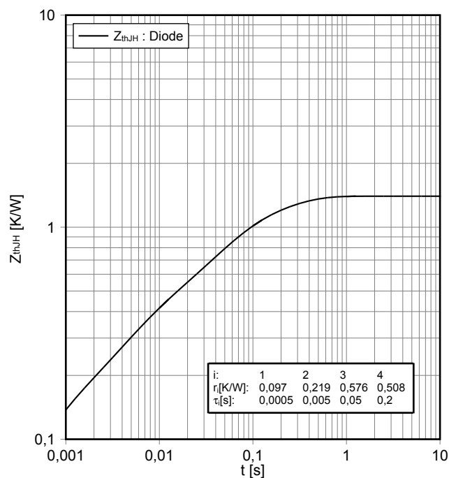
過渡熱インピーダンス Diode-、チョッパ transient thermal impedance Diode-Chopper Z_{thJH} = f(t)
