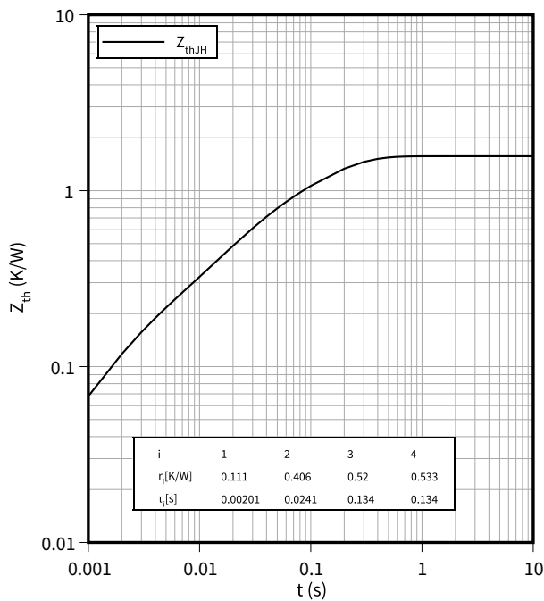
過渡熱インピーダンス, Diode、整流器 Zth = f(t)
