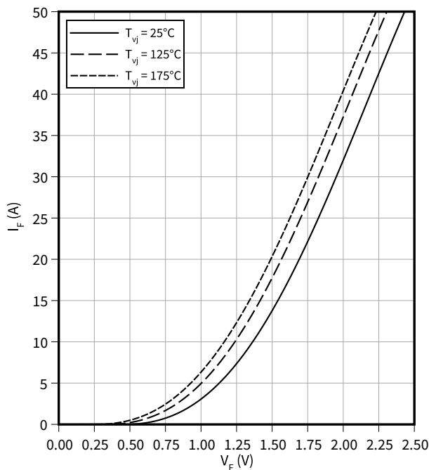
正向特性（典型）, Diode, D3 / D4
