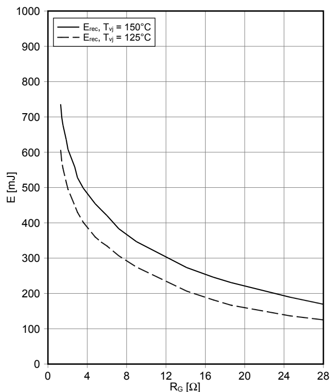
スイッチング損失 Diode、インバータ (Typical) switching losses Diode, Inverter (typical) E_{rec} = f(R_G) I_F = 500\text{ A} , V_{CE} = 1800\text{ V}
