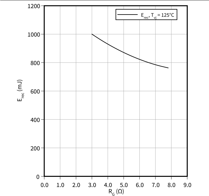
スイッチング損失 (typical), Diode、インバータ E_{rec} = f(R_G) V_{CE} = 3600\text{ V}, I_F = 250\text{ A}
