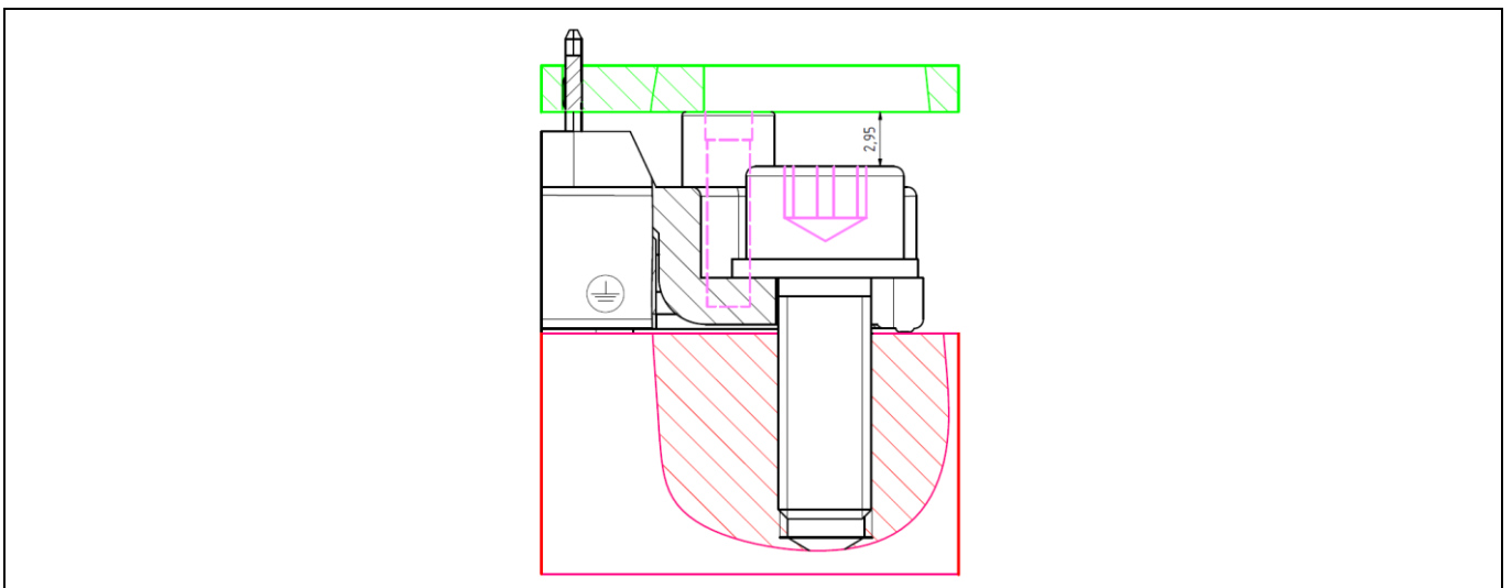
图 21 Easy3B 封装的夹具和 PCB 之间的空间距离
