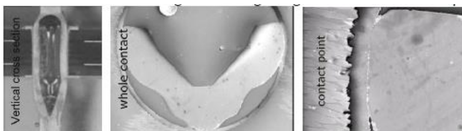
图 2 Easy PressFIT 管脚截面图
