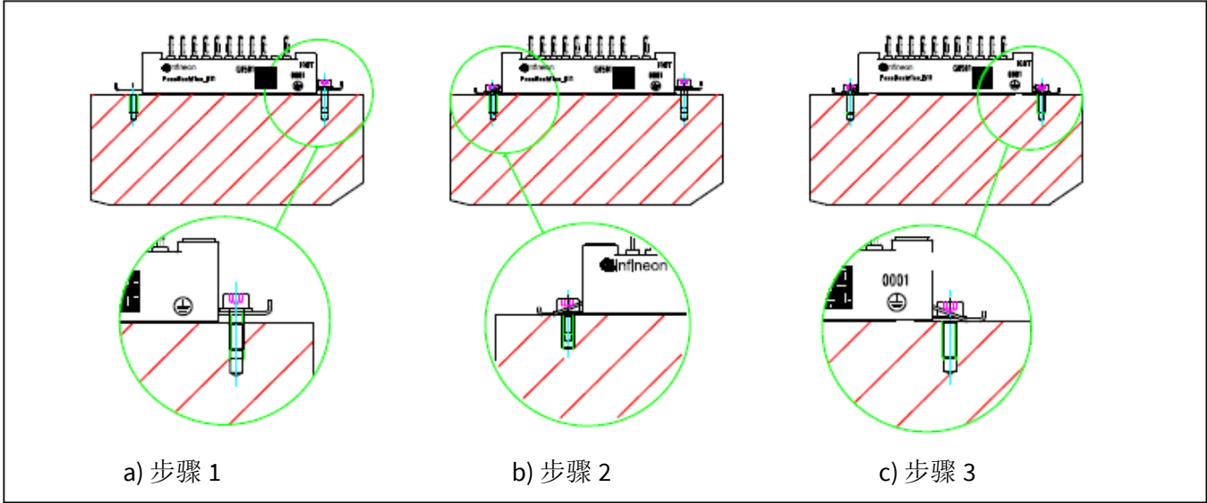
图 16 同时拧紧两个螺丝进行固定
