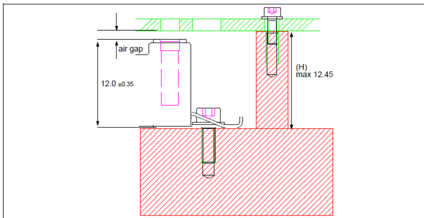
图 24 最终系统组装的放大图（图纸不符合比例）
