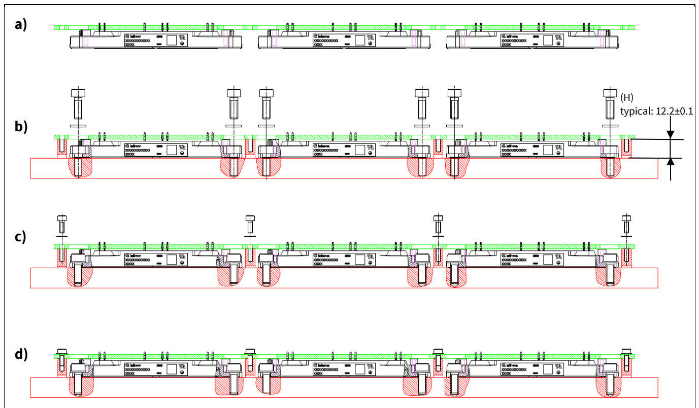
图 26 范例：PCB 和模块（仅 Easy3B 模块）安装到冷却系统上（图纸不符合比例）
