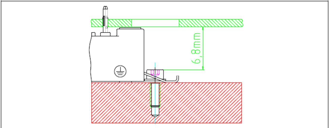
图 20 Easy1B 和 Easy2B 封装的夹具与 PCB 之间的空间距离
