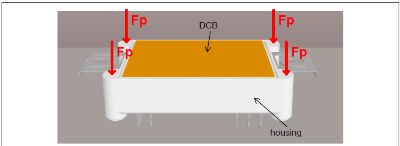
图 3 在模块处理过程中应避免外壳受力，防止 DCB 被推出
