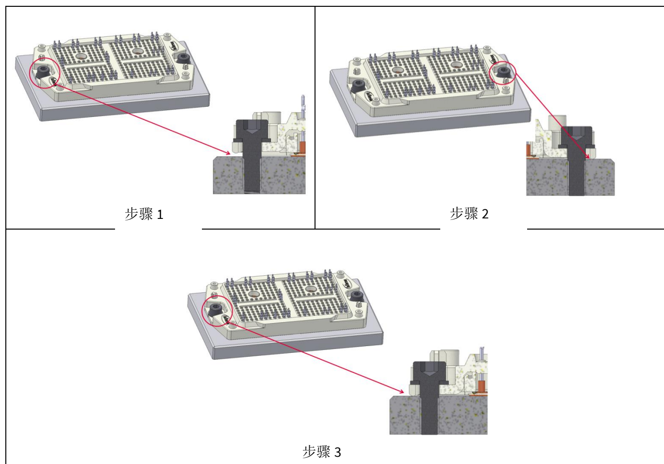
图 18 模块固定步骤
