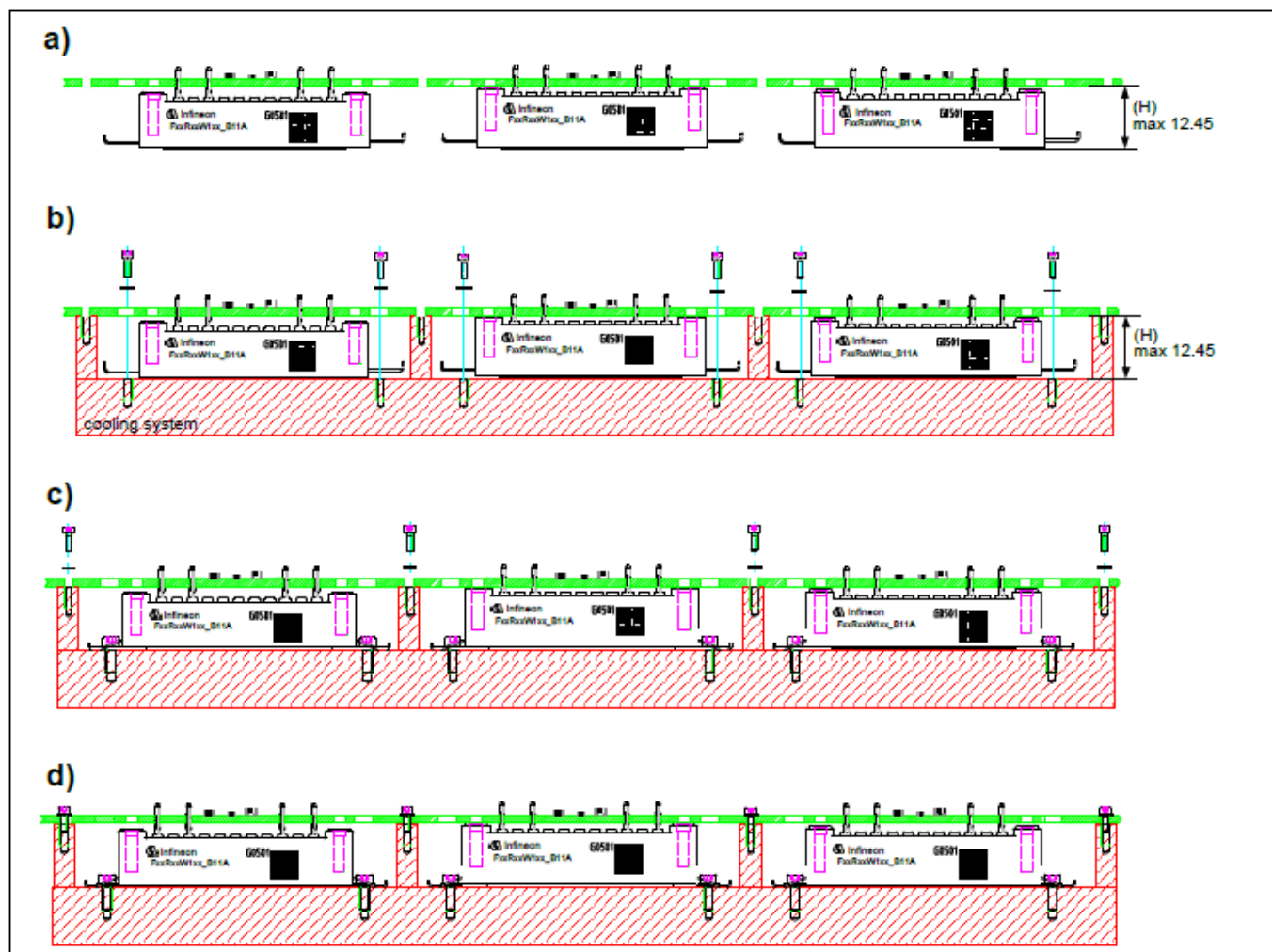
图 23 PCB 和模块安装到冷却系统 (图纸不符合比例)
