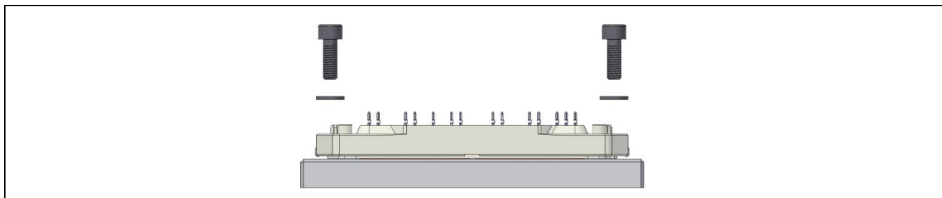
图 17 模块固定的步骤
