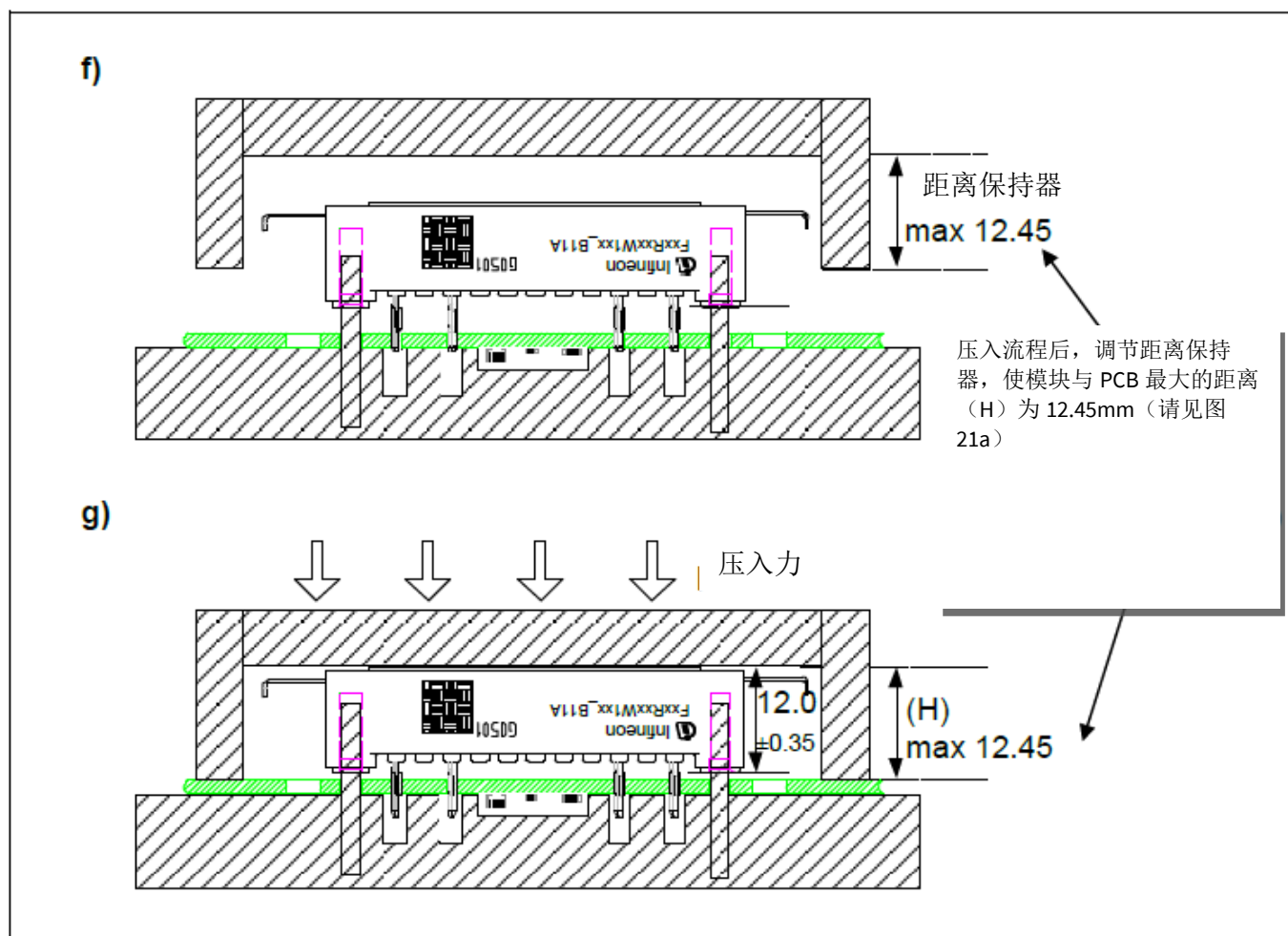
功率模块压入 (图纸不符合比例)
