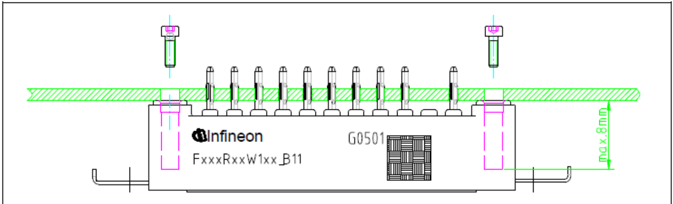
图 13 组装的详细视图
