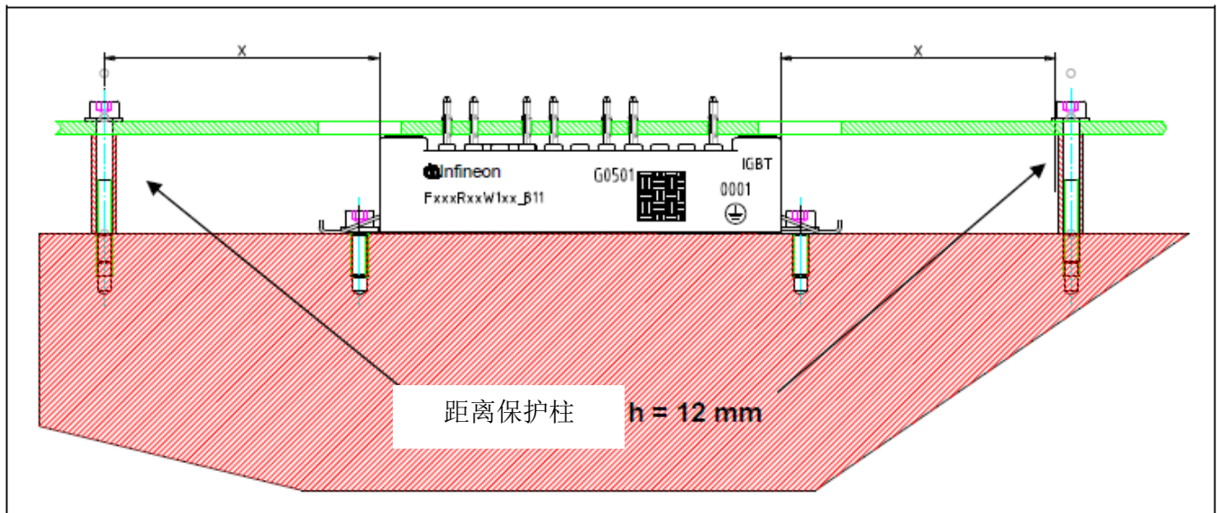
图 19 固定 PCB
