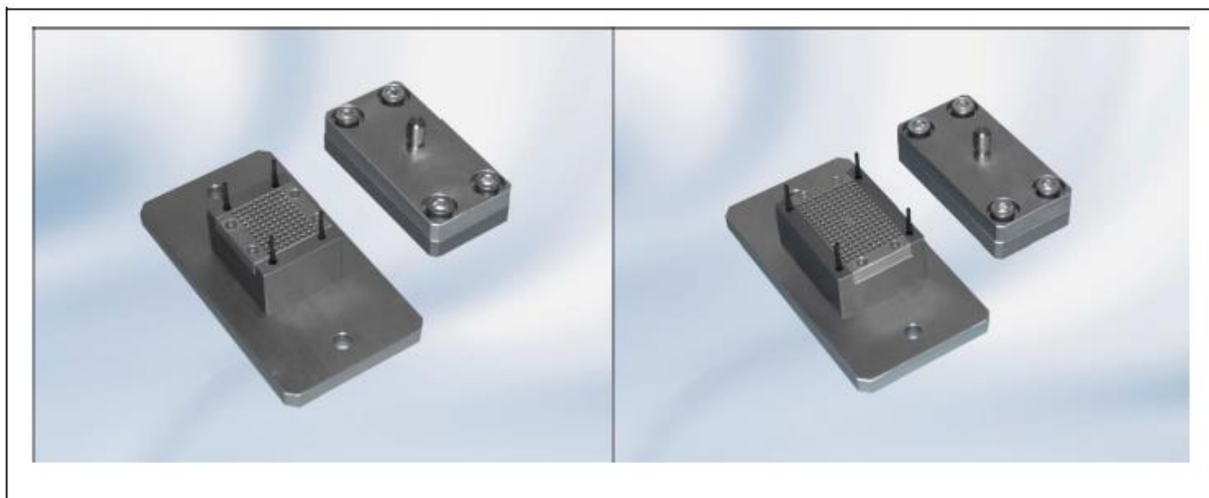
图 6 用于 Easy1B (左)、Easy2B (右) 的压接工具
