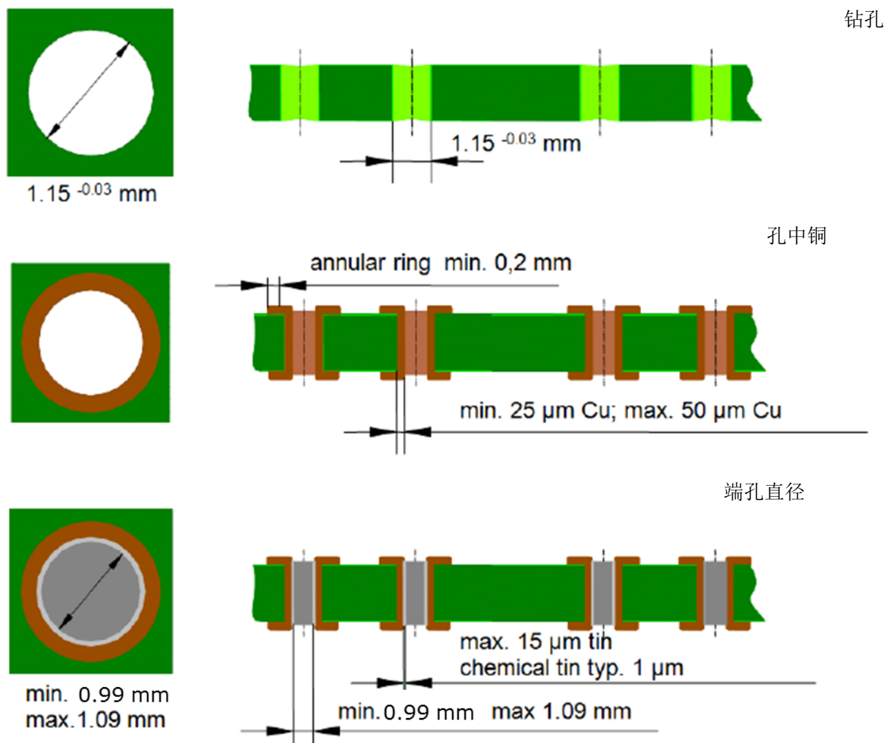
图 4 PCB 结构
