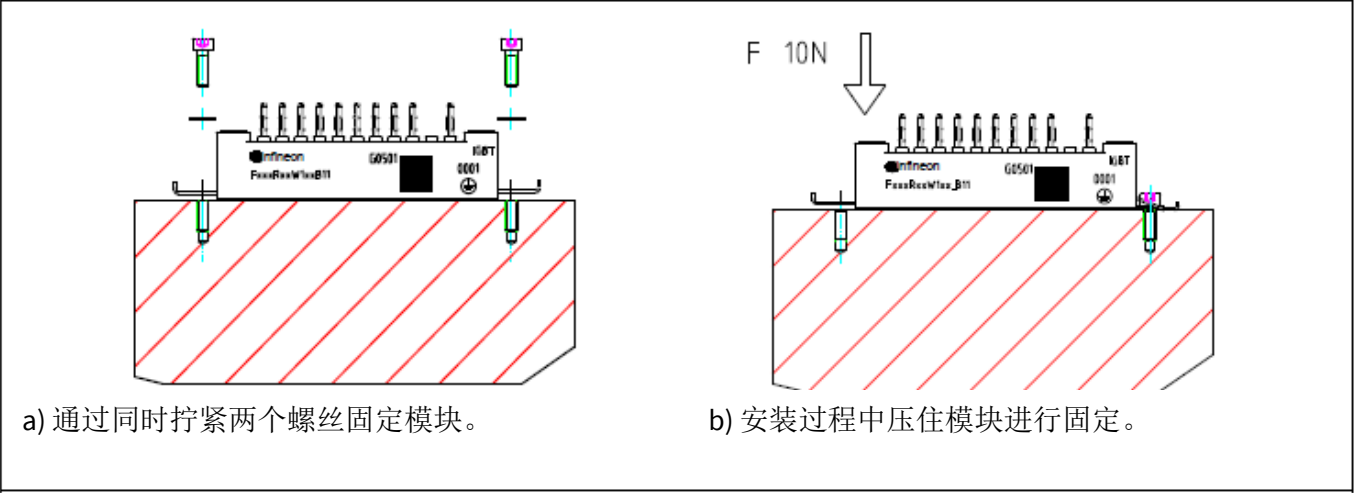
图 15 模块固定选项
