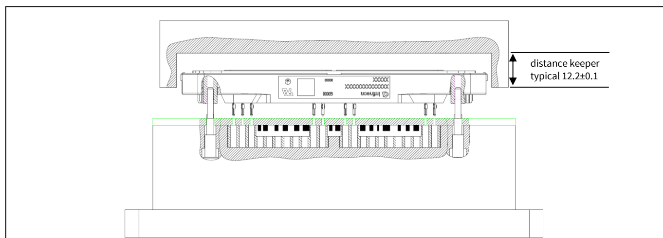
图 25 适用于 Easy3B 模块的典型距离保护柱
