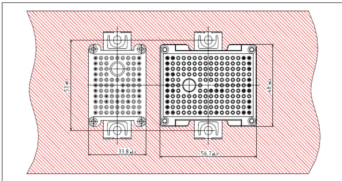
图 14 螺纹孔间距
