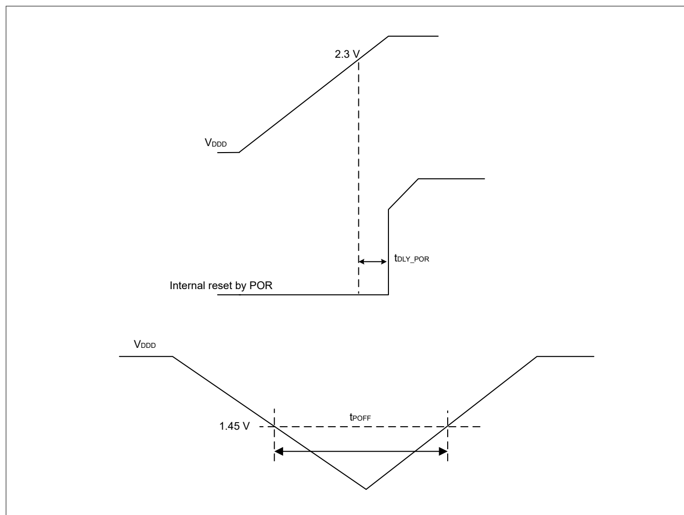
Figure 23 POR specifications
