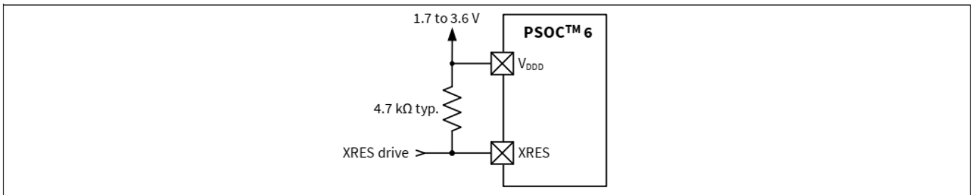
图 5 XRES 连接图
