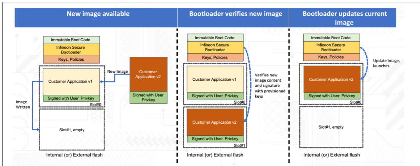
图 12 引导加载程序应用程序更新序列
