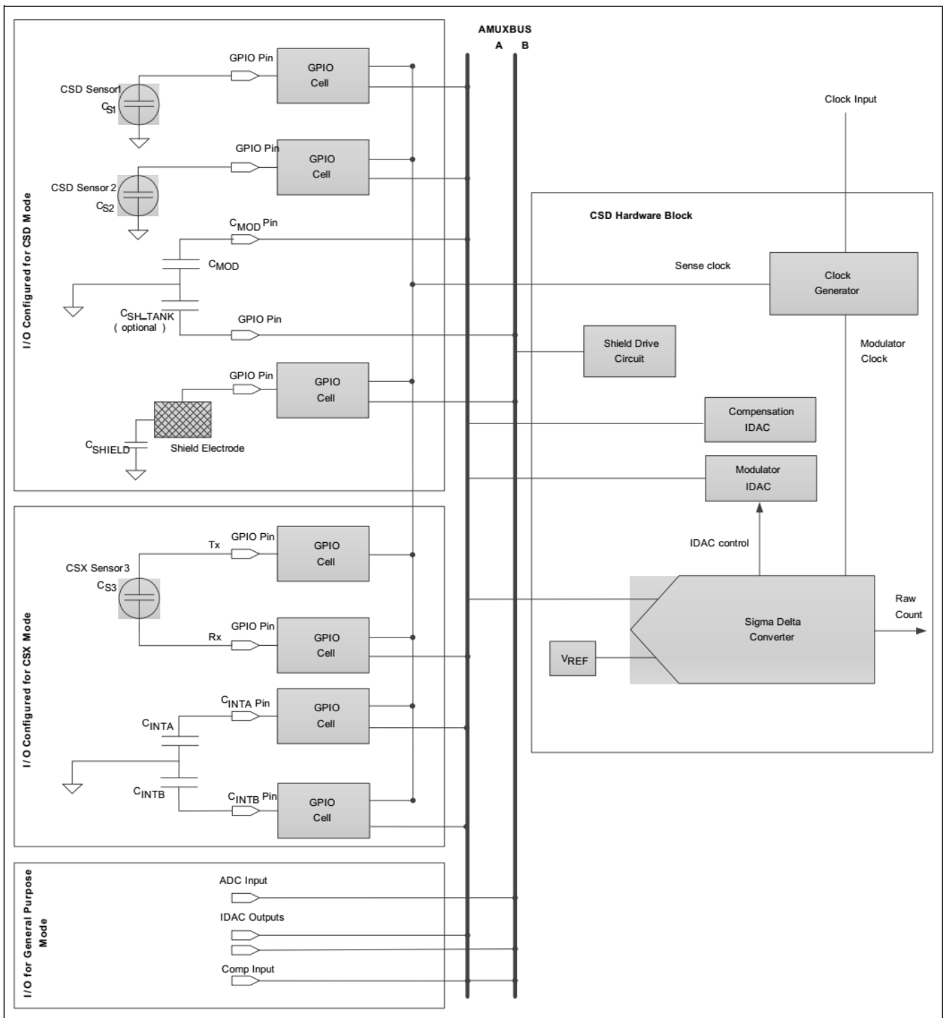
图 7 CAPSENSE™ 硬件子系统
