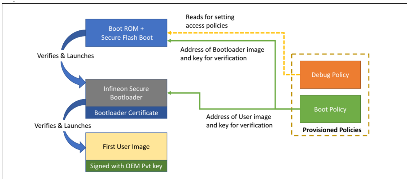
图 11 引导加载程序启动序列
