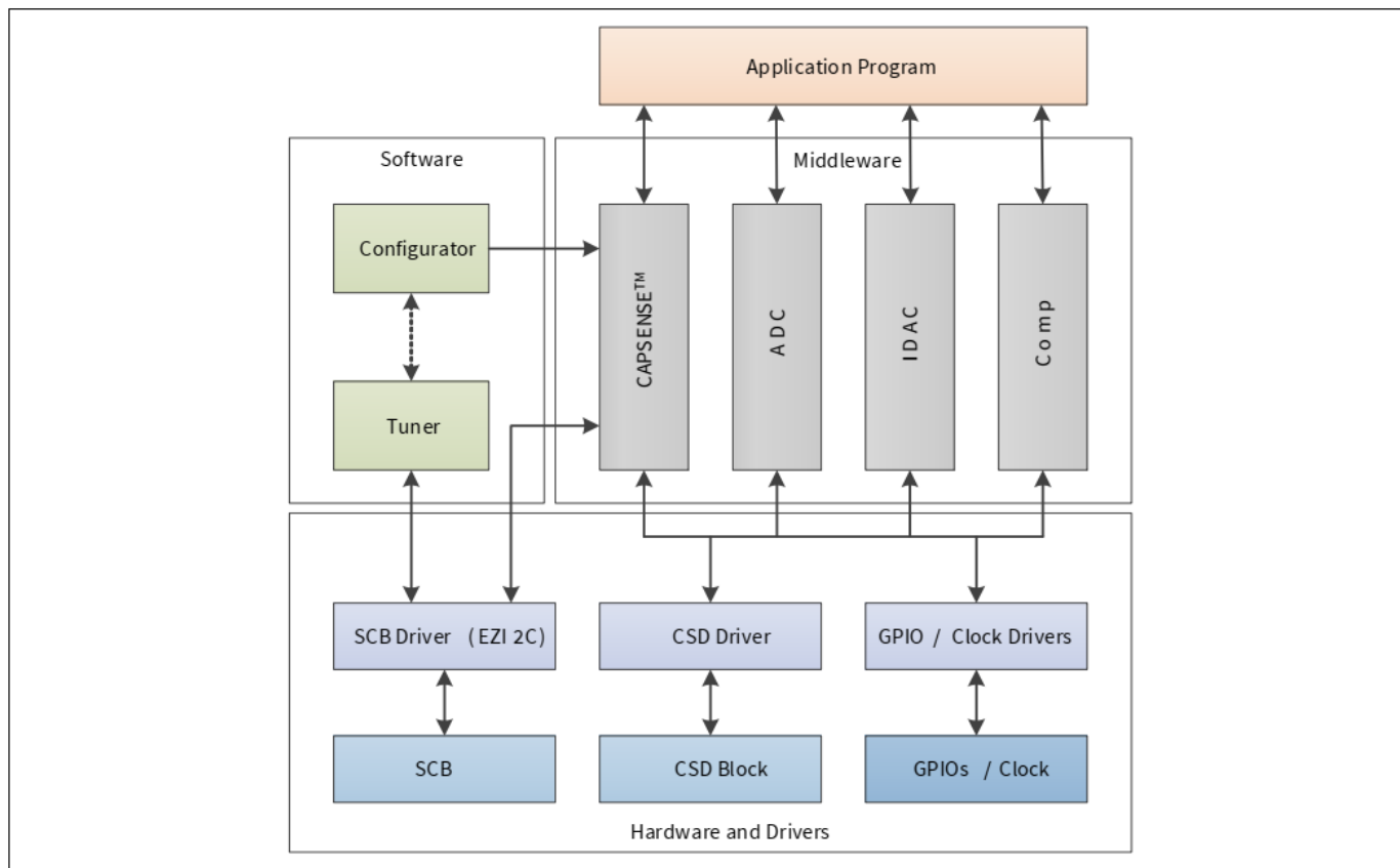
图 8 CAPSENSE™ 软件/固件子系统
