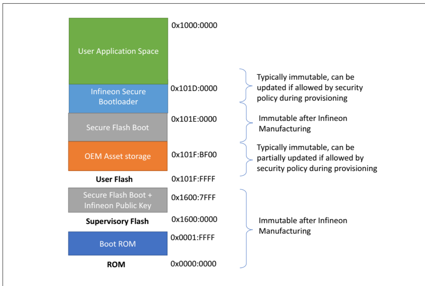
图 10 PSOC™ 64“安全”MCU 资产内存映射
