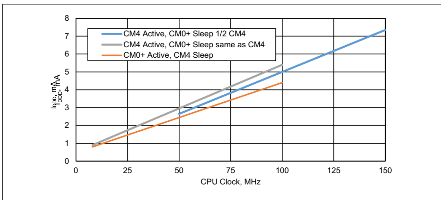
图 17 典型设备电流与 CPU 频率的关系；系统低功耗 (LP) 模式。
