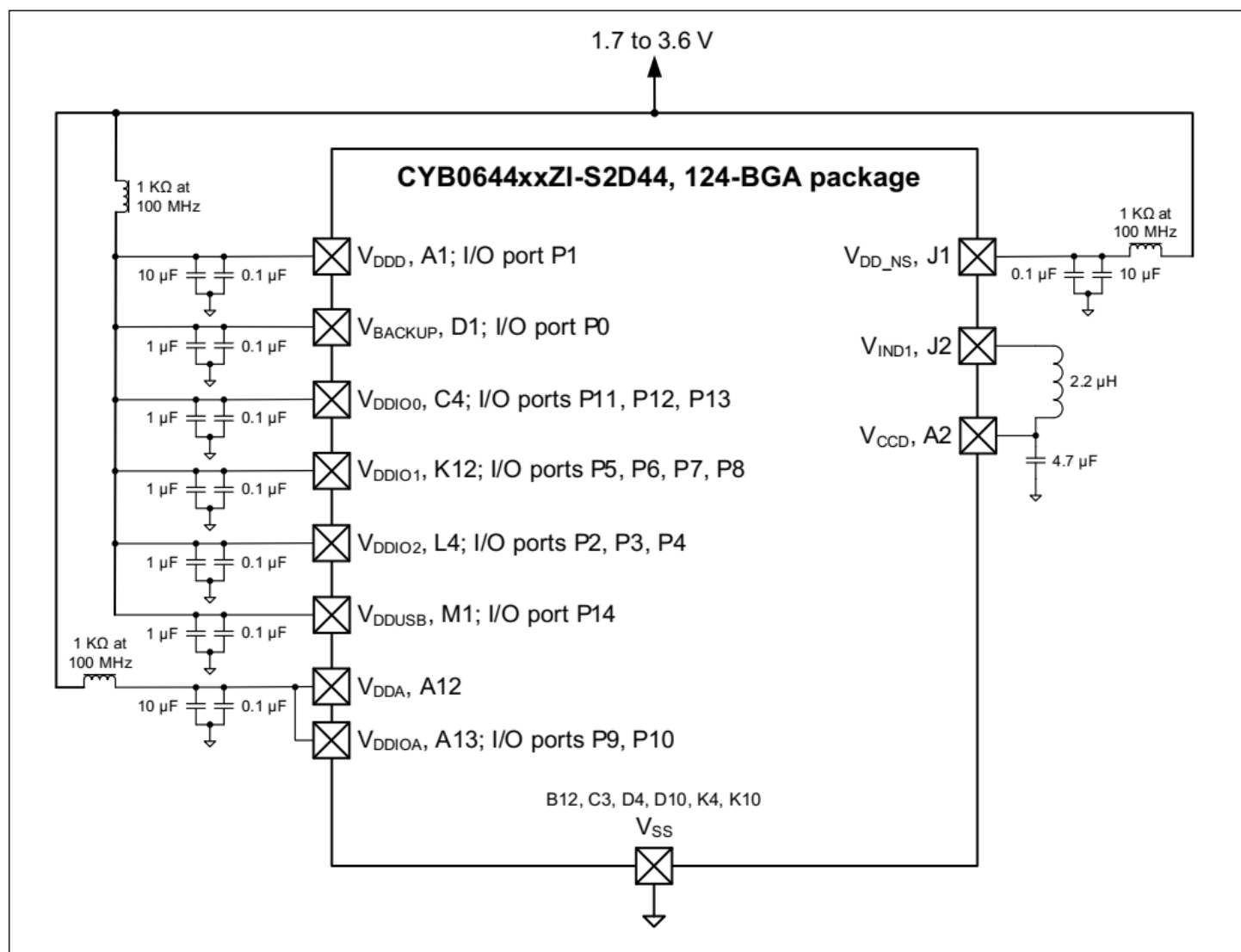
图 13 124-BGA电源连接图
