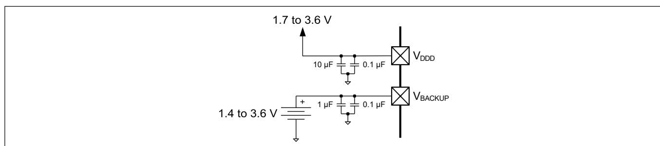
图 16 单独的电池连接到 V_{BACKUP}
