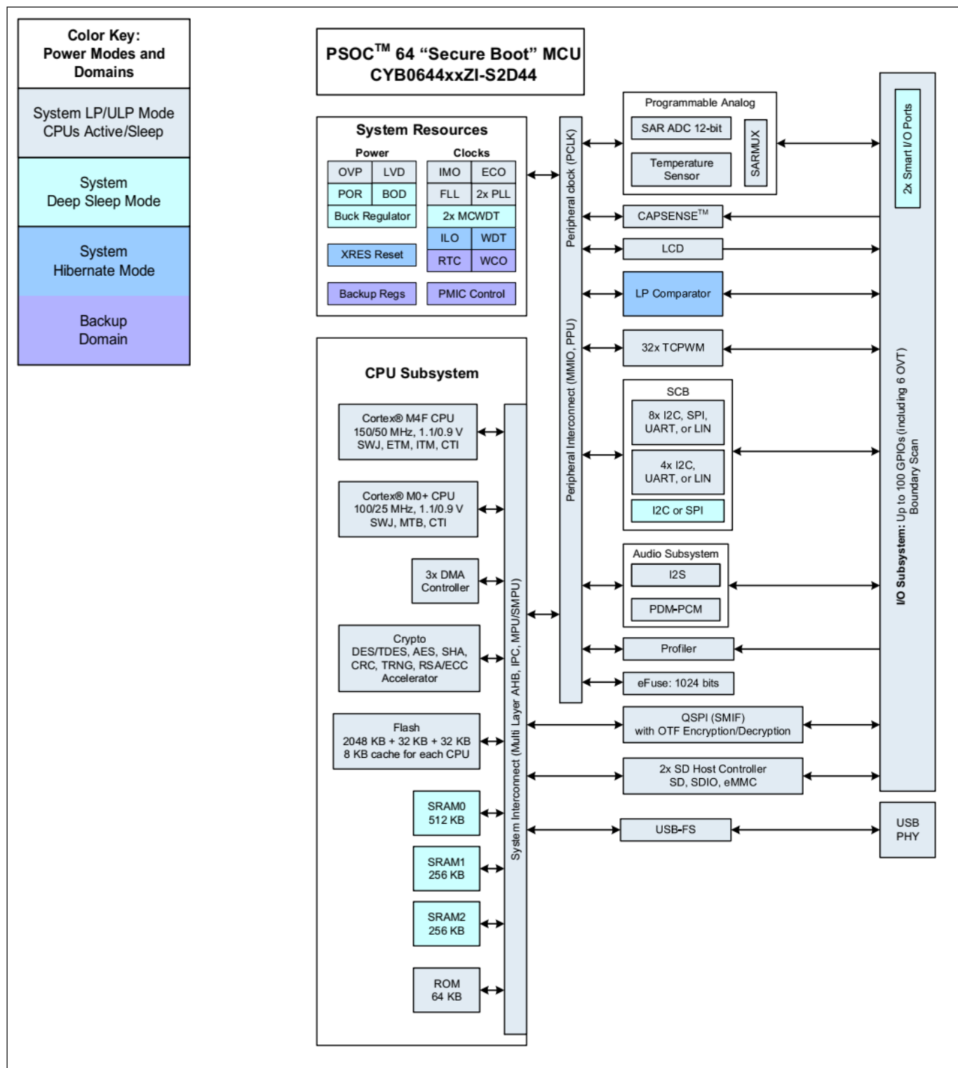
图 2 框图
