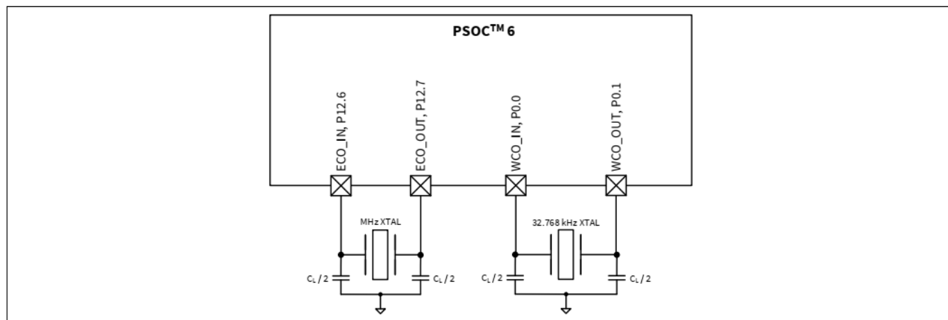
图 4 振荡器电路
