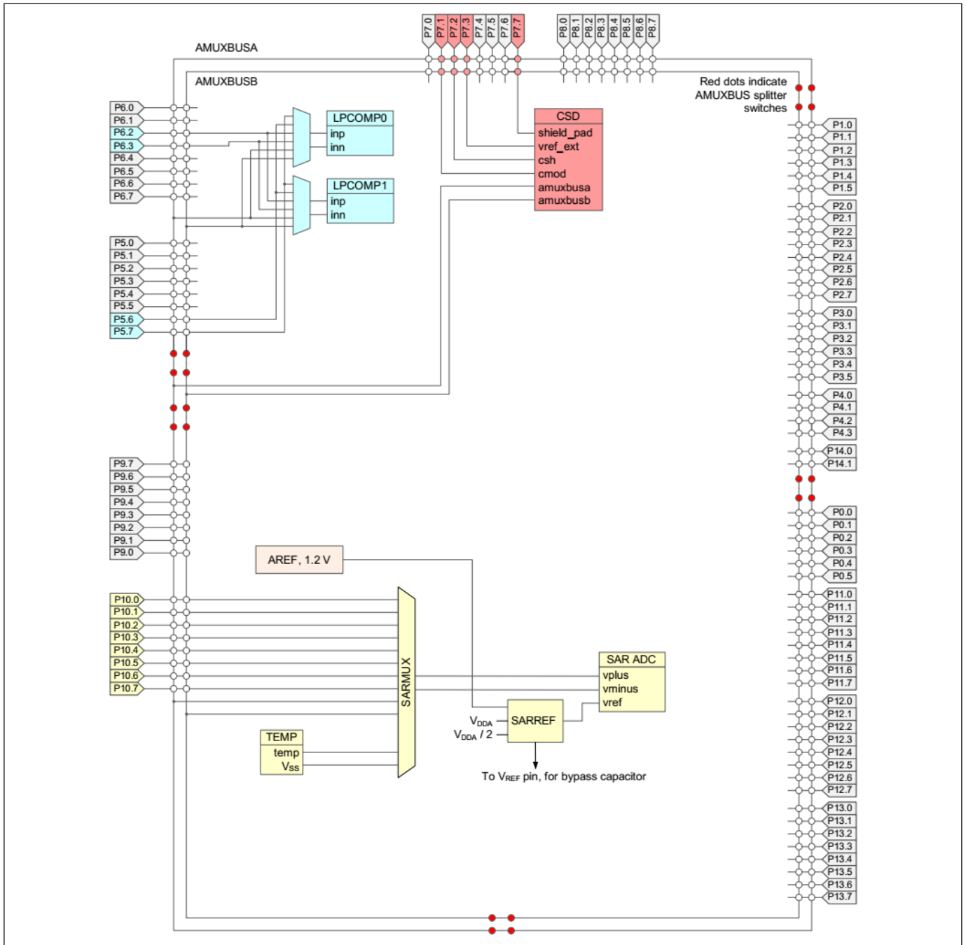
图 6 模拟子系统
