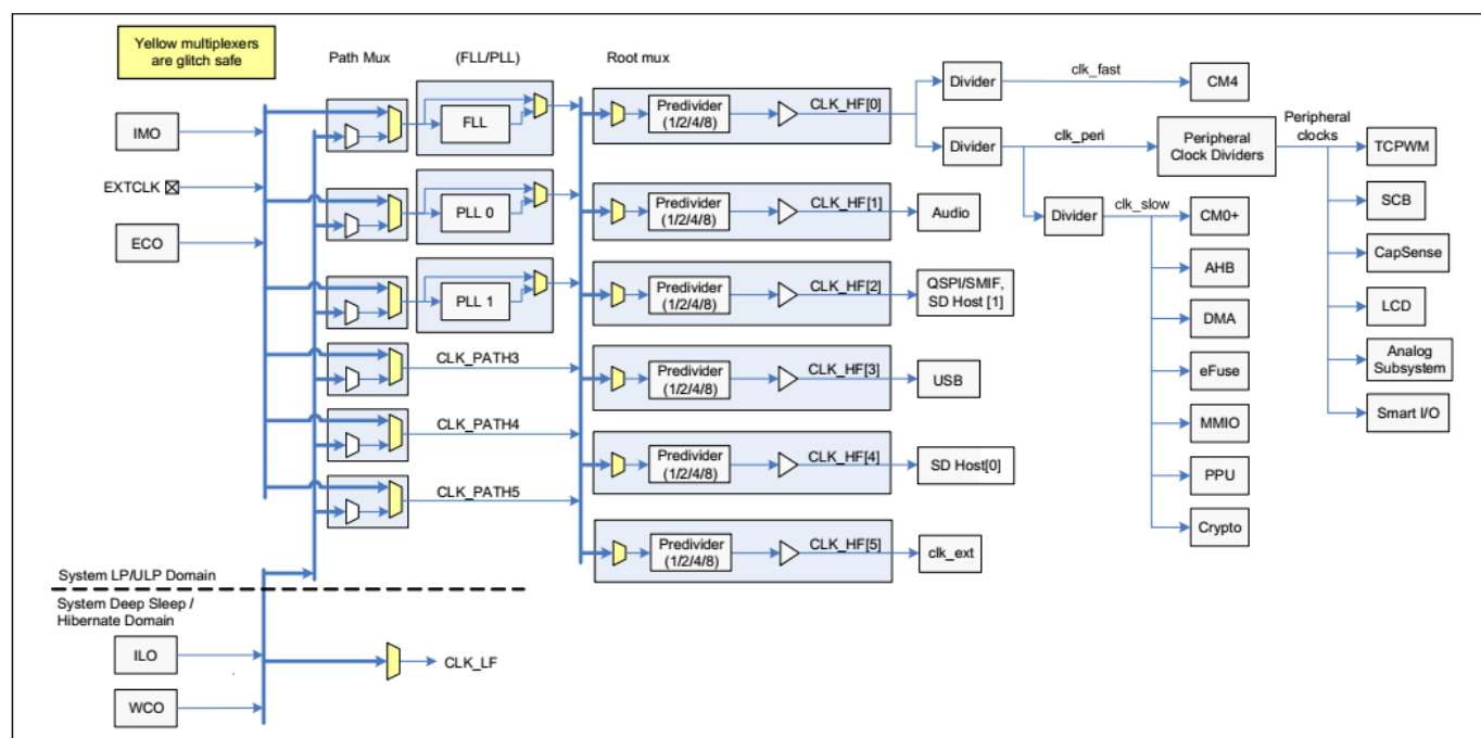
图 3 时钟图
