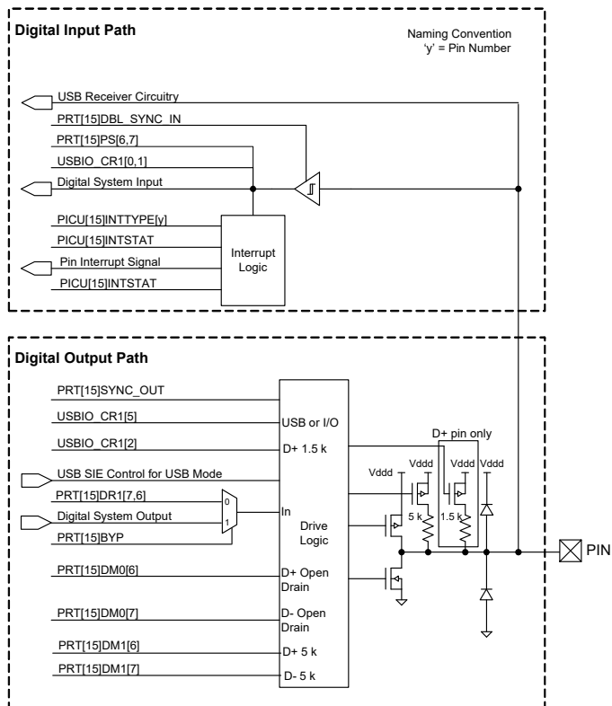
図 6-11. USBIO のブロックダイヤグラム
