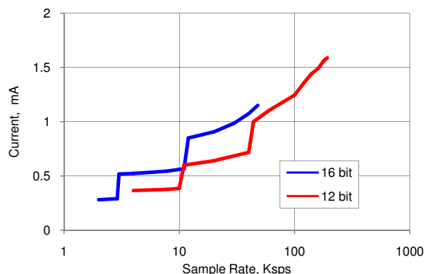
図 11-33. デルタシグマ ADC IDD 対 sps、レンジ = \pm 1.024V 、連続サンプル モード、入力バッファがバイパスされる
