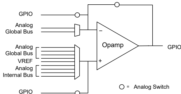
図 8-8. オペアンプ
