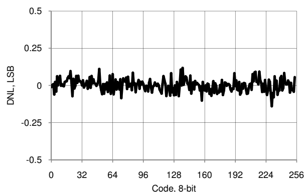
図 11-62. VDAC DNL 対入力コード、1V モード
