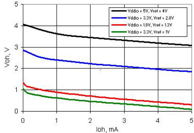
図 11-19. SIO 出力 HIGH 電圧および電流、安定化モード
