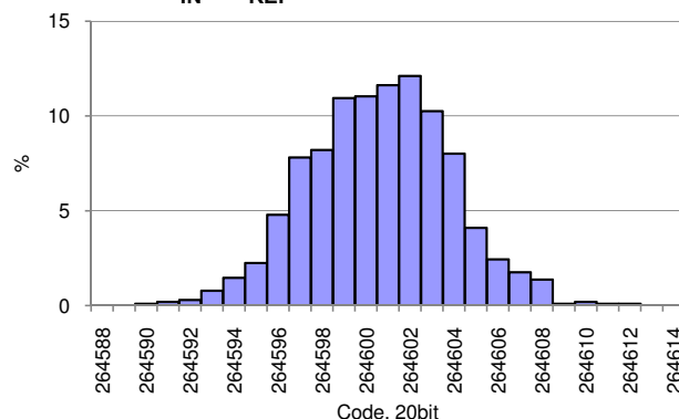
図 11-34. デルタシグマ ADC ノイズ ヒストグラム、1000 サンプル、20 ビット、187sps、外部リファレンス、 V_{IN} = V_{REF}/2 、レンジ = \pm 1.024V
