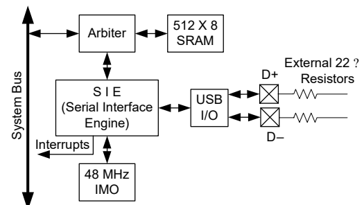
図 7-16. USB
