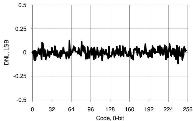
図 11-50. IDAC DNL 対入力コード、レンジ = 255 \mu A、シンク モード
