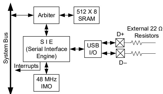
図 7-16. USB
