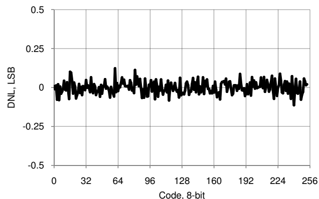
図 11-45. IDAC DNL 対入力コード、 レンジ = 255 \mu A、シンク モード
