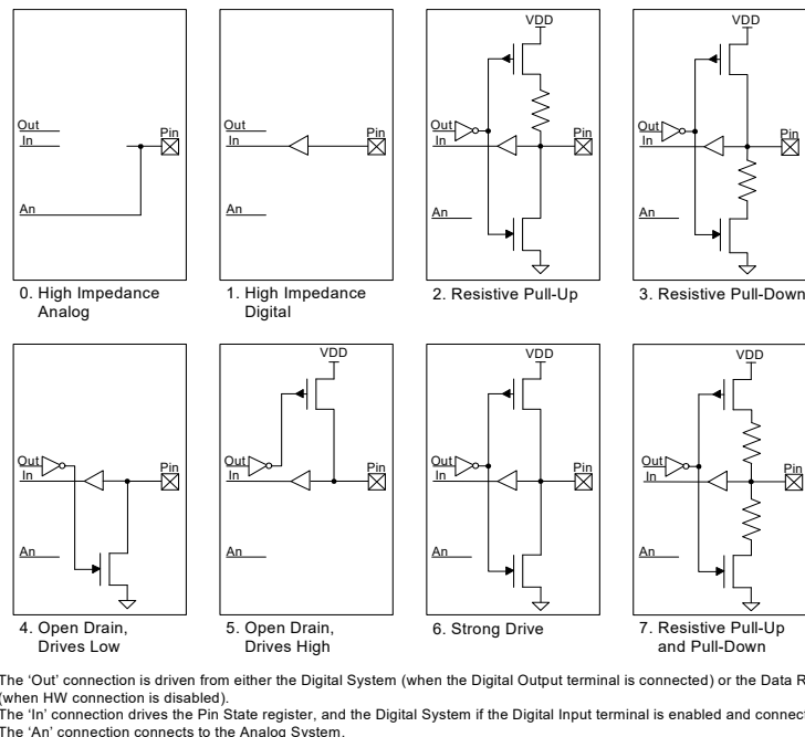
図 6-12. 駆動モード
