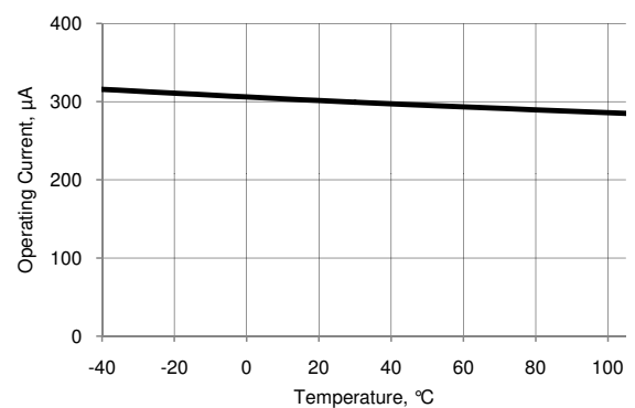
図 11-63. VDAC 動作電流対温度、1V モード、高速モード
