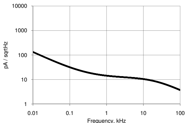
図 11-53. IDAC 電流ノイズ、255 \mu A モード、 ソース モード、高速モード、 V_{DDA} = 5V
