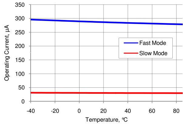
図 11-49. IDAC 動作電流対温度、範囲 = 255 \mu A、コード = 0、 シンク モード
