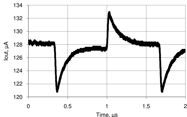
図 11-53. IDAC 電流ノイズ、255 \mu A モード、 ソース モード、高速モード、 V_{DDA} = 5V
