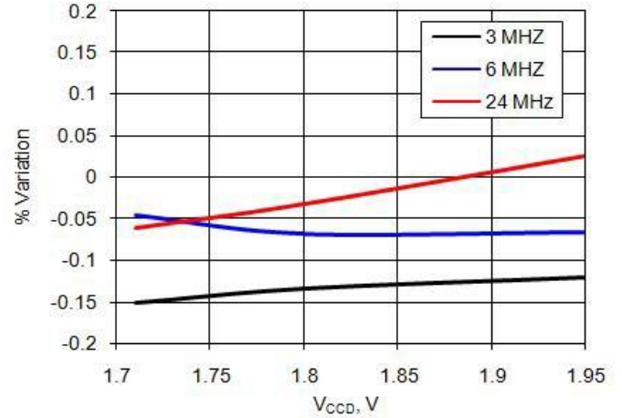
图 11-76. IMO 频率变化与 V CC
