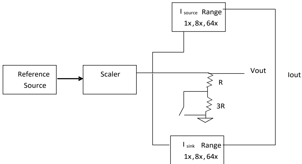
图 8-12. DAC 框图
