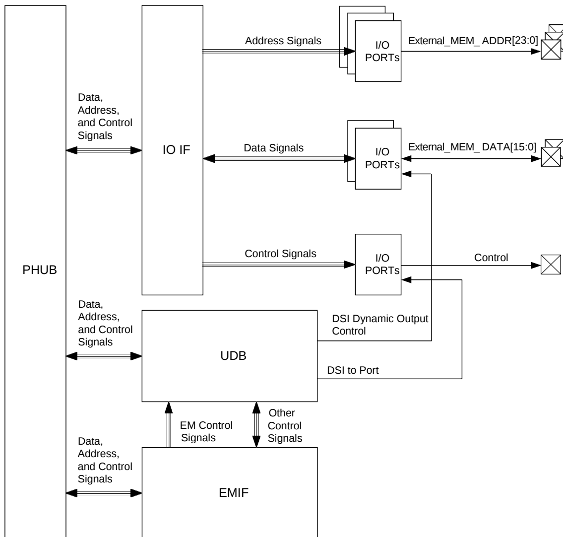
图 5-1. EMIF 框图
