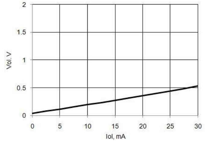
图 11-23. USBIO 输出低电平电压和电流，GPIO 模式
