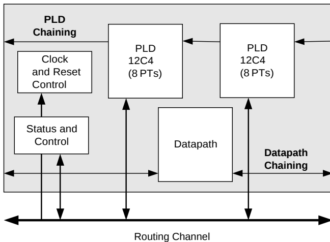
图 7-2. UDB 框图
