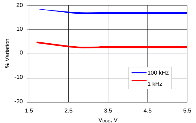
图 11-78. ILO 频率变化与 V_{DD}
