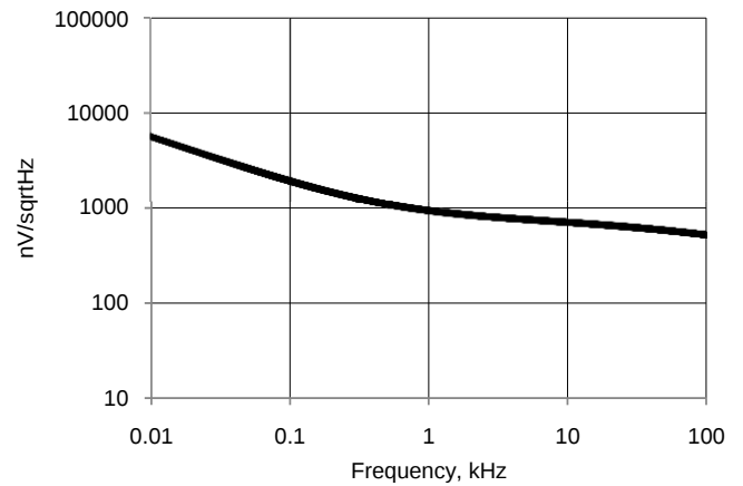
图 11-65. VDAC 电压噪声, 1 V 模式, 快速模式, V_{DDA} = 5\text{ V}
