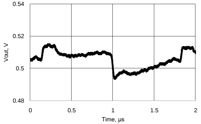
图 11-65. VDAC 电压噪声, 1 V 模式, 快速模式, V_{DDA} = 5\text{ V}
