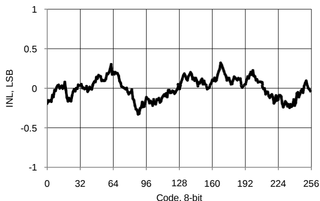
图 11-41. IDAC INL 与输入代码，范围 = 255 \mu A，灌电流模式
