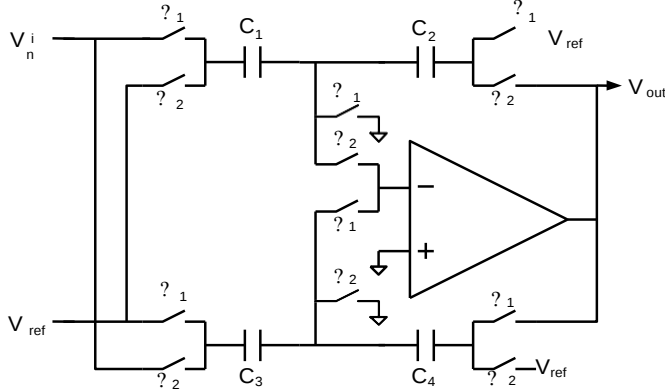
图 8-14. 采样和保持拓扑（Φ1 和 Φ2 是时钟的两个对立相）
