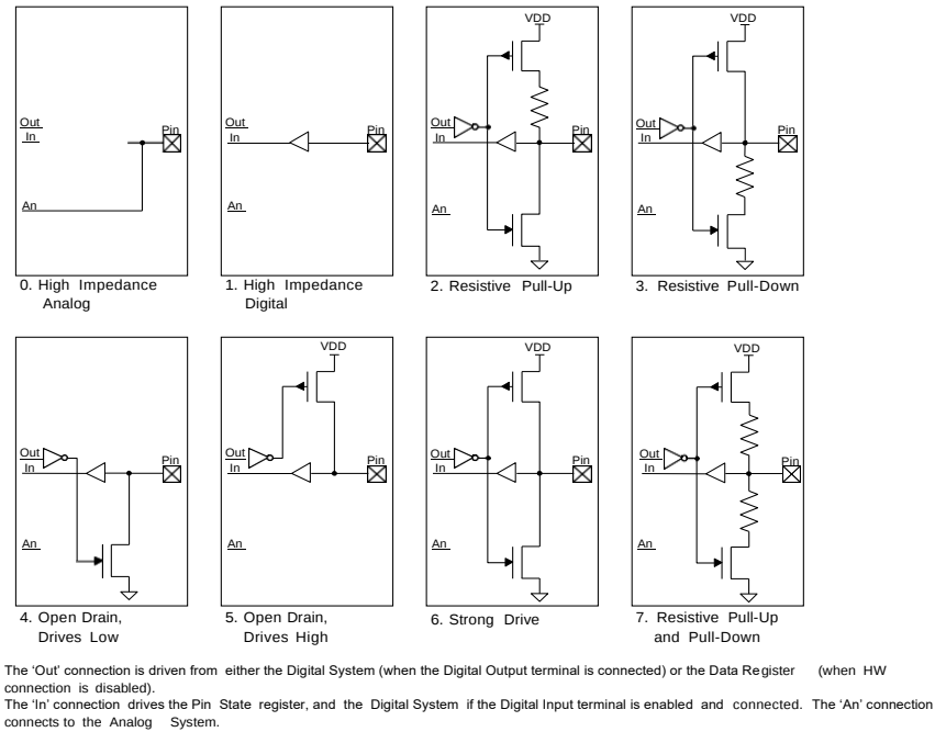
图 6-12. 驱动模式
