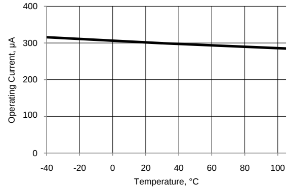
图 11-61. VDAC 工作电流与温度，1 V 模式，快速模式
