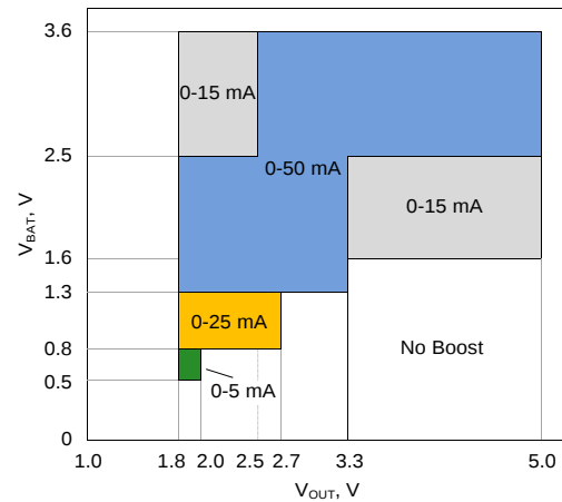
图 11-9. 在 V_{\text{BAT}} 与 V_{\text{OUT}} 范围内的 I_{\text{OUT}} 范围
