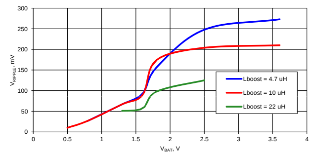
图 11-14. V_{RIPPLE} 与 V_{BAT} [30]
