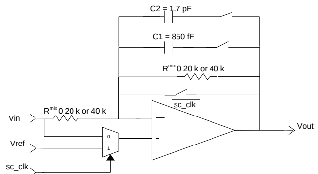
图 8-13. 混频器配置
