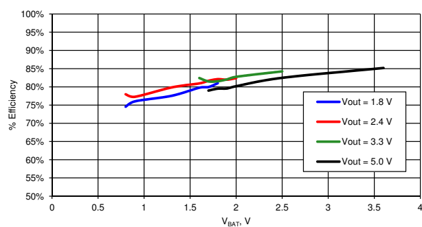
図 11-12. V_{BAT} 、 L_{BOOST} = 10\mu H [28] の時の効率
