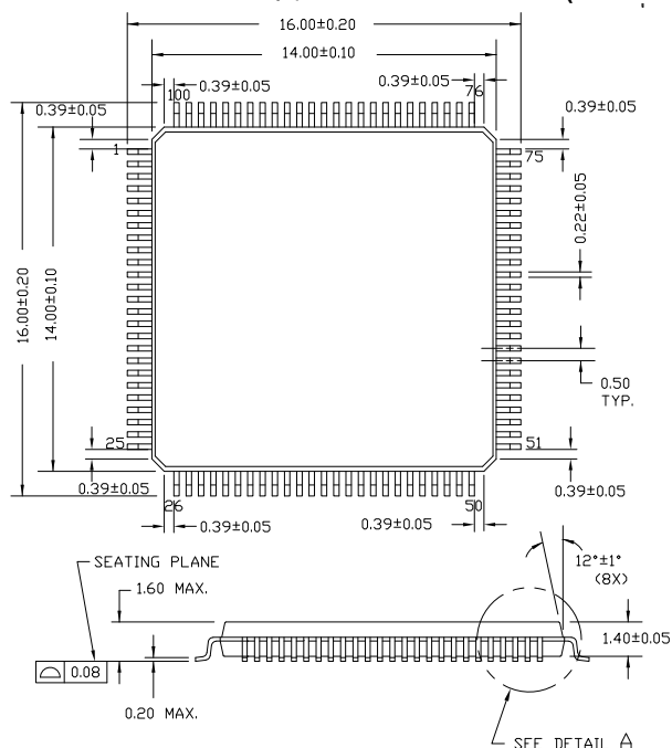
図 13-2. 100 ピン TQFP (14×14×1.4 mm) のパッケージ外形図 (PG-TQFP-100)
