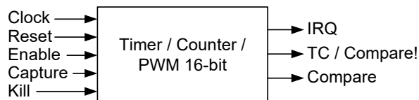
図 7-15. タイマー / カウンター / PWM
