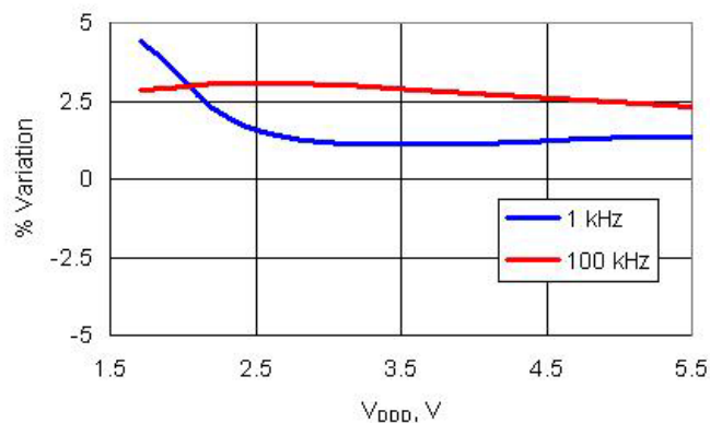
図 11-66. ILO 周波数変化対 V_{DD}
