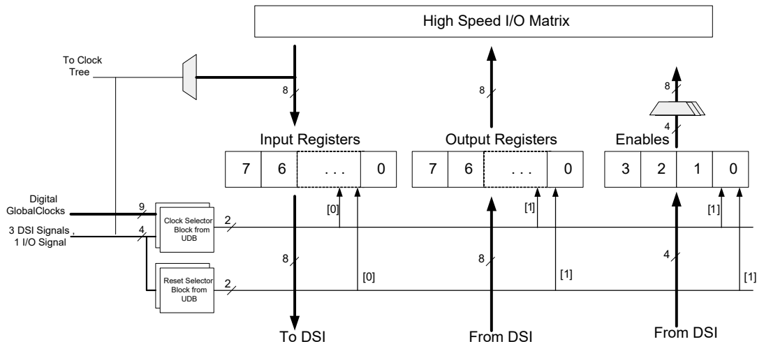
图 7. 端口接口
