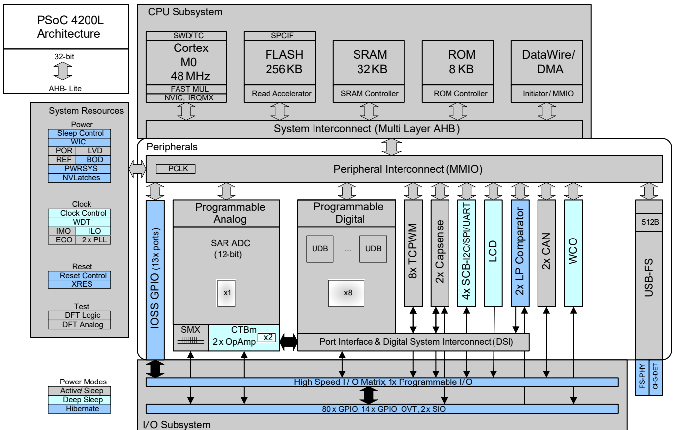
图 2. 框图
