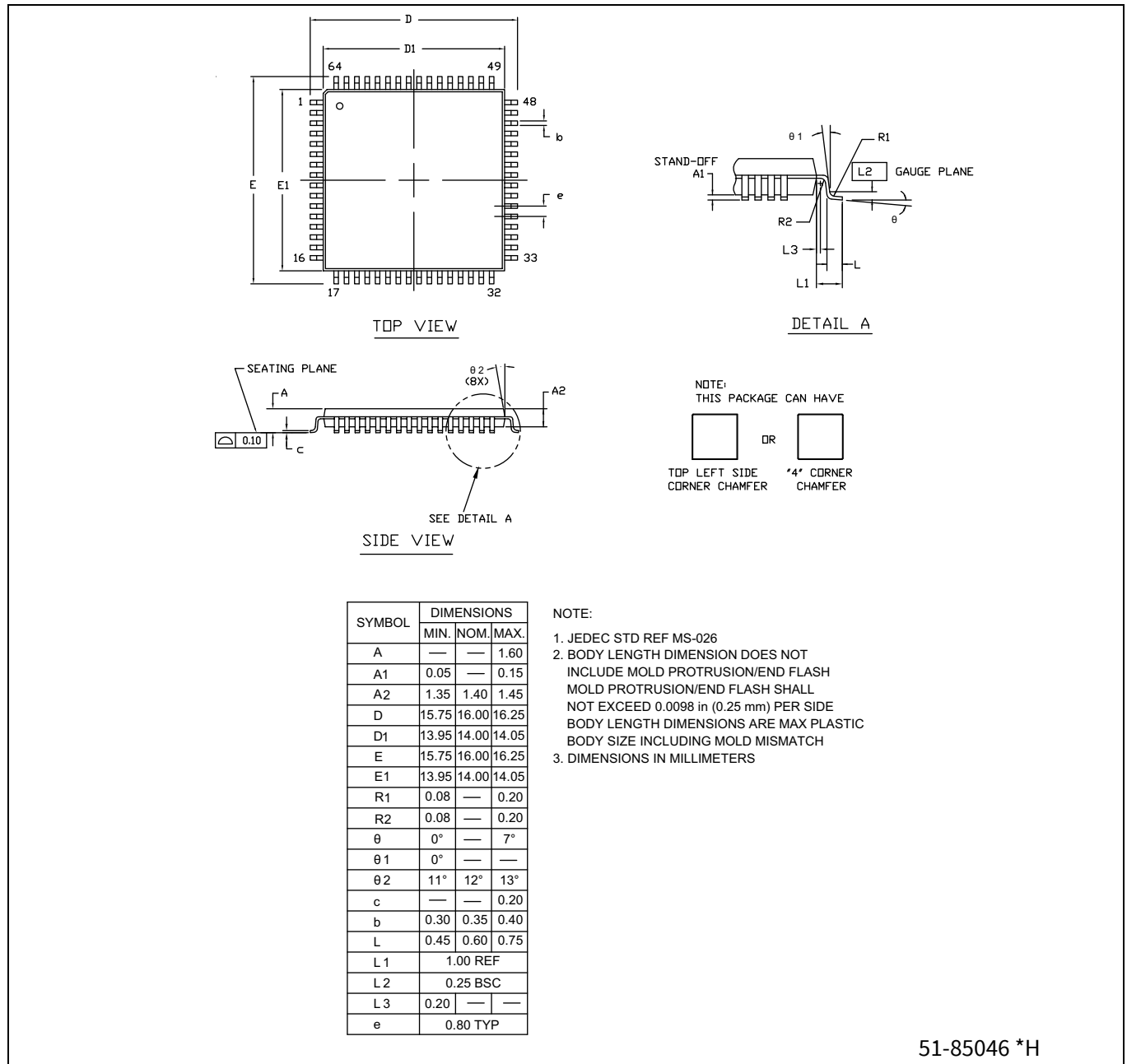
Figure 7 64LD TQFP 14.0x14.0x1.4 MM A64SA パッケージ外形図 (PG-TQFP-64)
