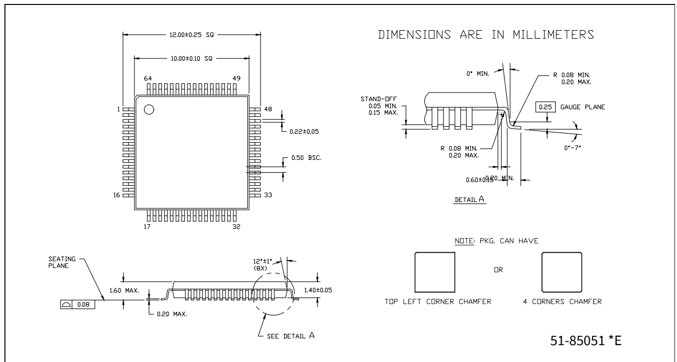
Figure 8 64LD TQFP 10x10x1.4 MM A64SB パッケージ外形図 (PG-TQFP-64)
