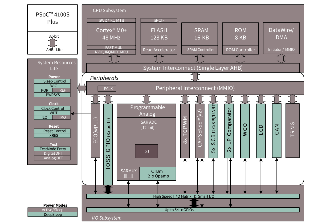
框图
