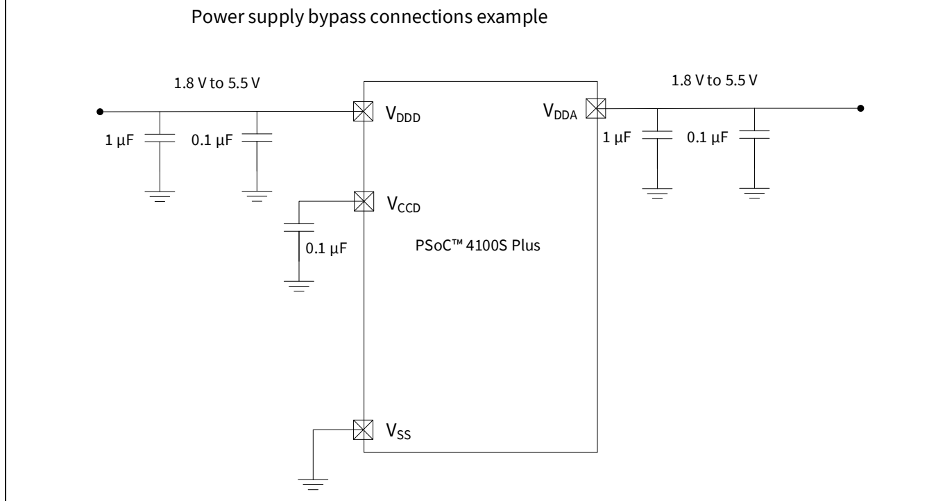
Figure 6 外部电源 ( 电压范围从 1.8 V 到 5.5 V, 使能内部电压调节器 )
