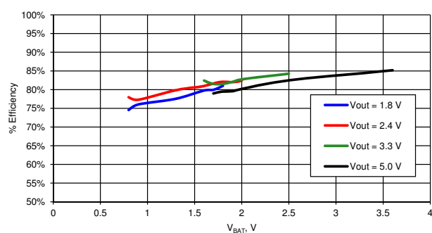
图 11-12. 效率与 V_{BAT} , L_{BOOST} = 10 \mu H [37]
