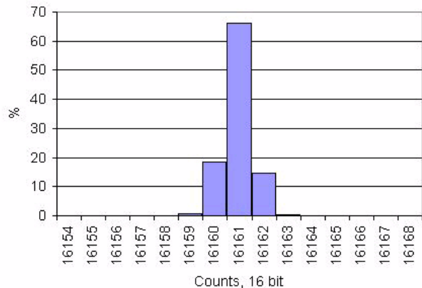
图 11-35. Delta-sigma ADC 噪声柱状图，1000 件样本，16 位，48 kspss，外部参考， V_{IN} = V_{REF}/2 ，范围 = \pm 1.024 V
