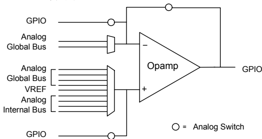
图 8-6. 运算放大器
