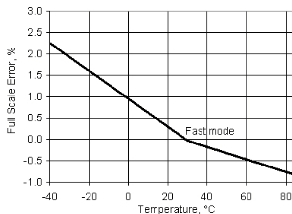
图 11-48. IDAC 全量程误差与温度，范围 = 255 \mu A，灌电流模式
