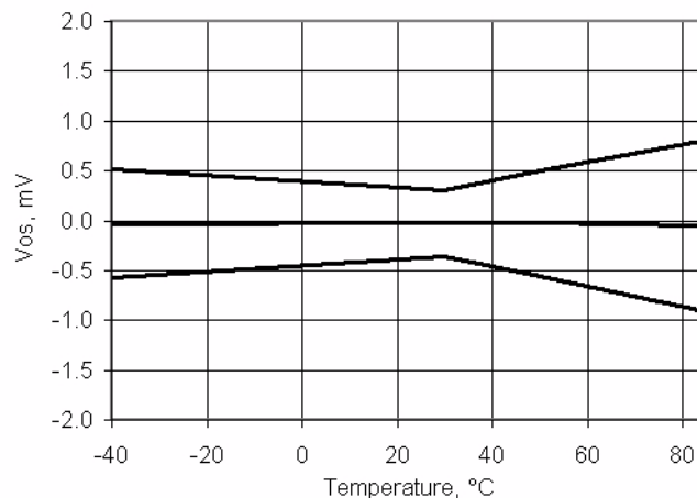
图 11-26. 运算放大器偏移与温度, V_{DDA} = 5\text{ V}
