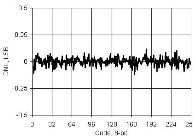
图 11-56. VDAC DNL 与输出代码，1 V 模式
