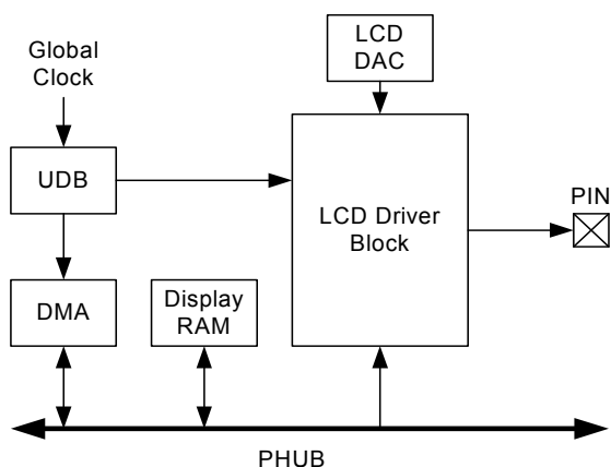
图 8-10. LCD 系统
