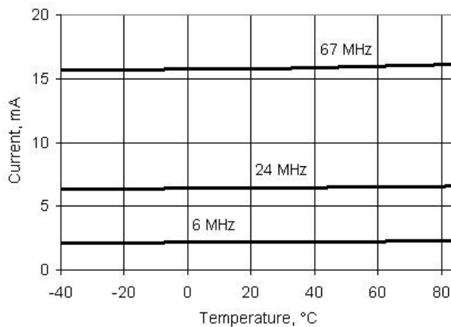
图 11-2. 活动模式电流与温度和 F_{CPU} , V_{DD} = 3.3\text{ V}
