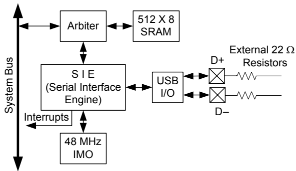
图 7-16. USB
