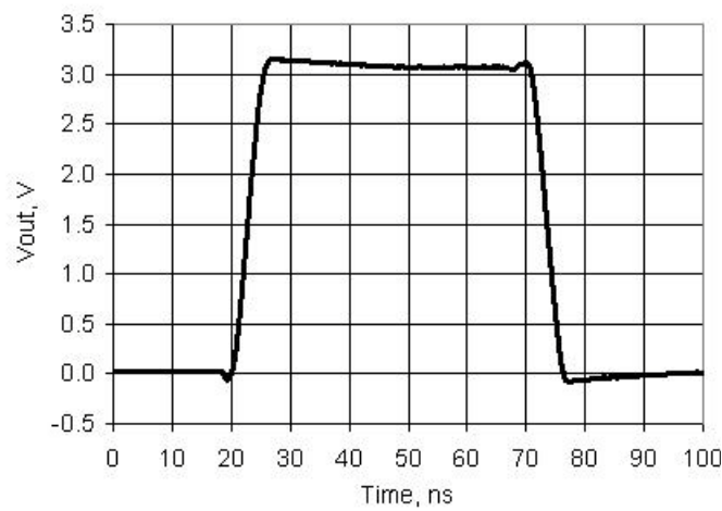
图 11-24. USBIO 输出上升和下降时间，GPIO 模式，V DD = 3.3 V，25 pF 负载
