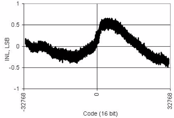
图 11-38. Delta-sigma ADC INL 与输出代码，16 位，48 ksp/s，25 °C V_{DDA} = 3.3\text{ V}
