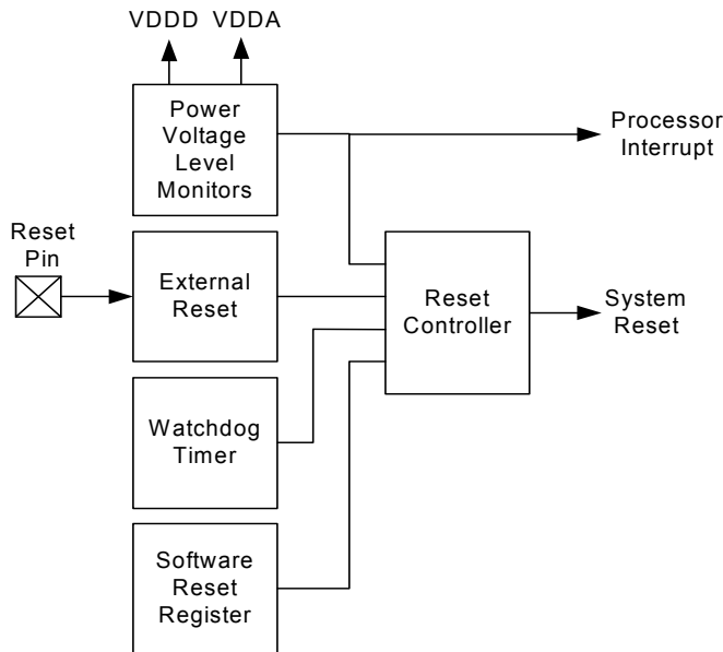
图 6-8. 复位
