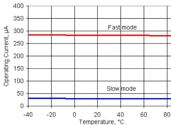
图 11-50. IDAC 工作电流与温度，范围 = 255 \mu A，代码 = 0，灌电流模式
