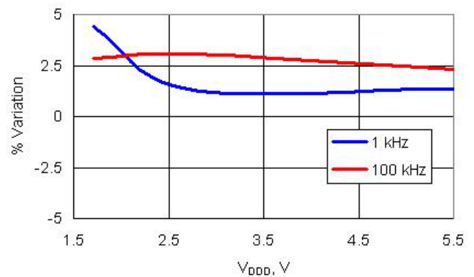
图 11-81. ILO 频率变化与 V_{DD}
