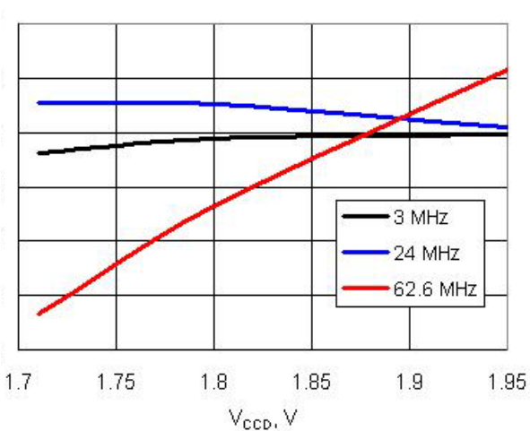
图 11-79. IMO 频率变化与 V CC
