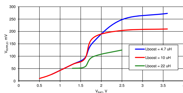
图 11-14. V_{RIPPLE} 与 V_{BAT} [37]
