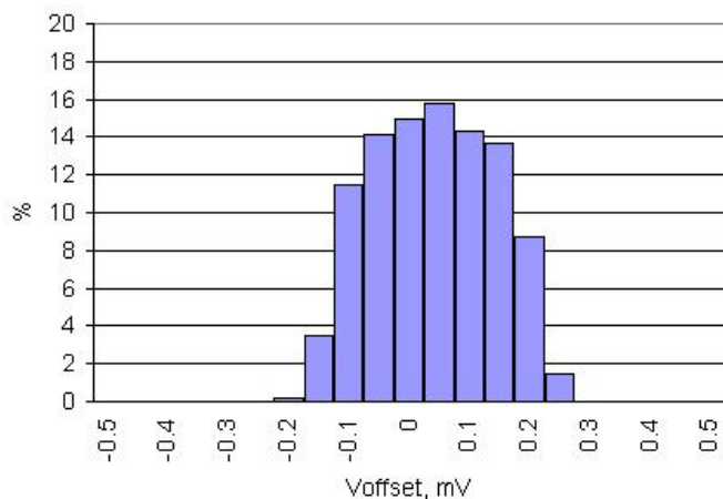
图 11-25. 运算放大器偏移柱状图, 3388 个采样 / 847 个器件, 25 °C, V_{DDA} = 5\text{ V}
