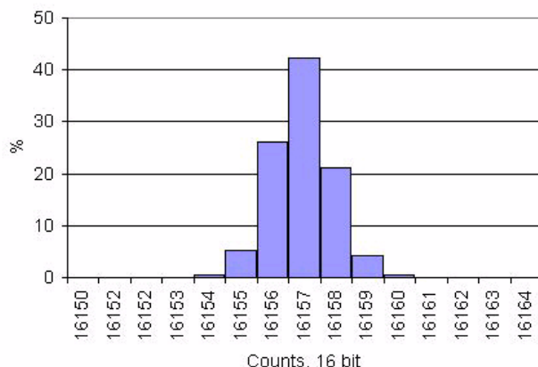
图 11-36. Delta-sigma ADC 噪声柱状图，1000 件样本，16 位，48 kspss，内部参考， V_{IN} = V_{REF}/2 ，范围 = \pm 1.024 V
