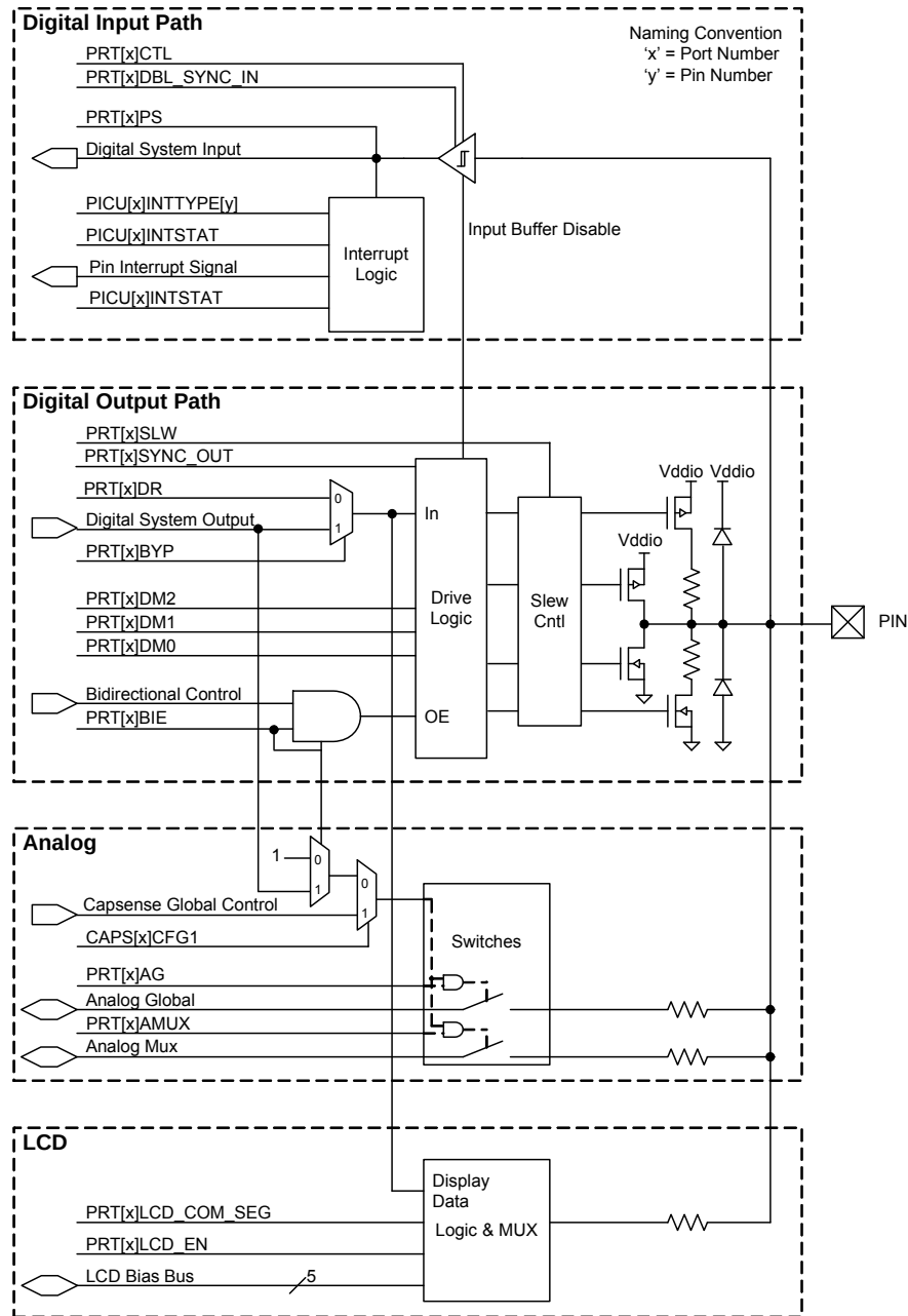
图 6-9. GPIO 框图
