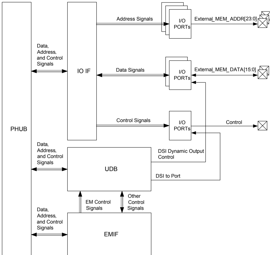
图 5-1. EMIF 框图
