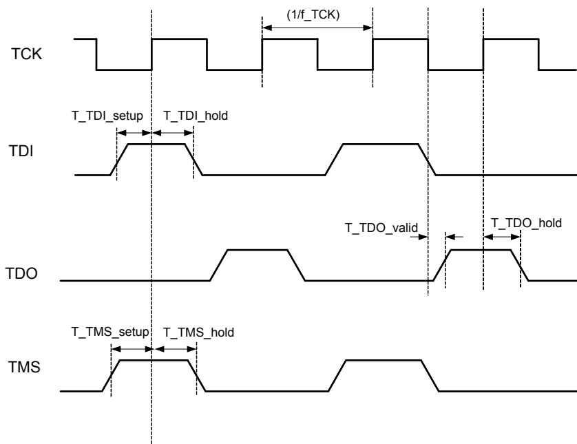
图 11-75. JTAG 接口时序
