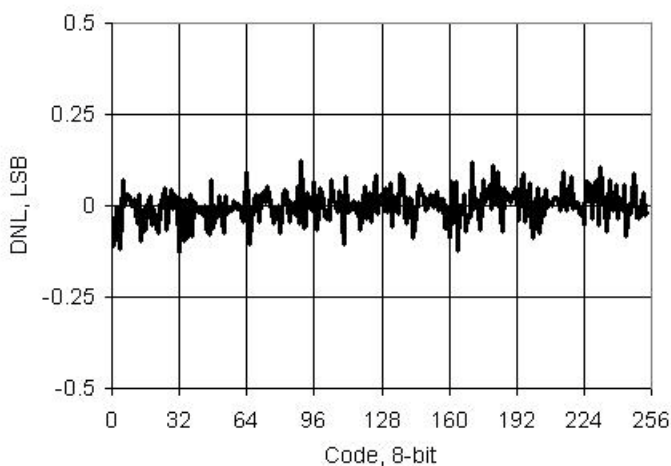
图 11-44. IDAC DNL 与输入代码，范围 = 255 \mu A，灌电流模式
