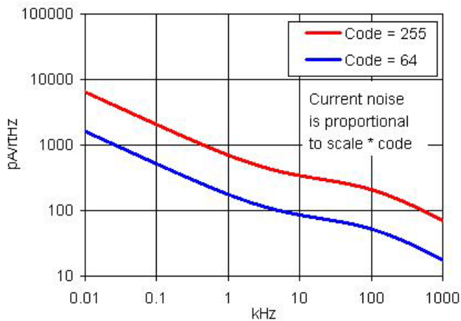
图 11-54. IDAC 当前噪声, 255 \mu A 模式, 拉电流模式, 高速模式, V_{DDA} = 5 V
