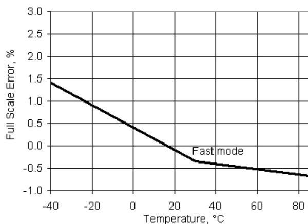
图 11-47. IDAC 全量程误差与温度，范围 = 255 \mu A，拉电流模式
