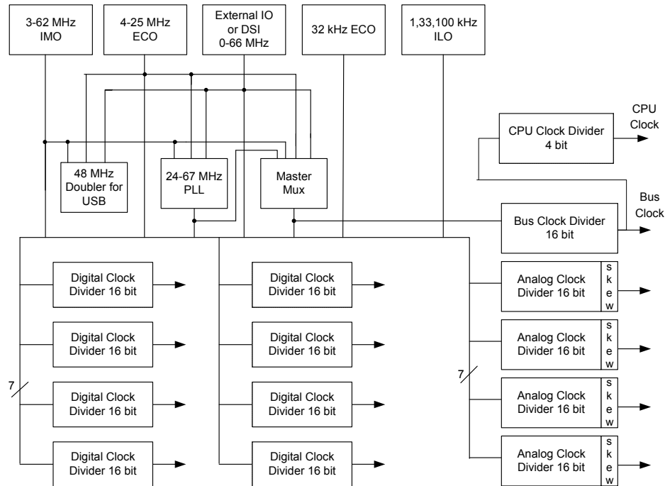
图 6-1. 时钟子系统
