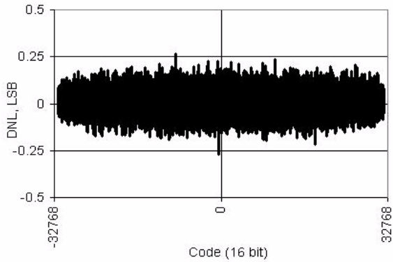
图 11-37. Delta-sigma ADC DNL 与输出代码，16 位，48 ksp/s，25 °C V_{DDA} = 3.3\text{ V}
