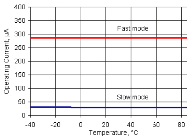
图 11-49. IDAC 工作电流与温度，范围 = 255 \mu A，代码 = 0，拉电流模式
