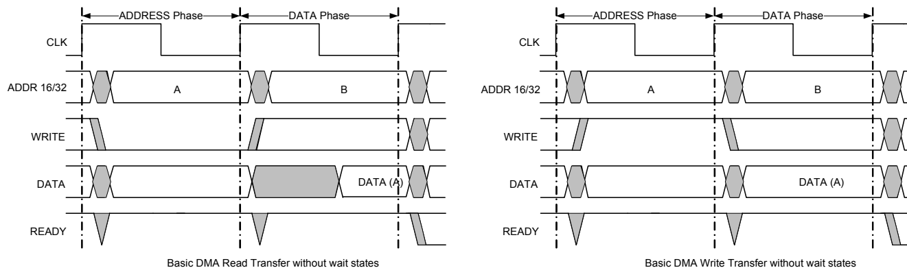
图 4-1. DMA 时序图
