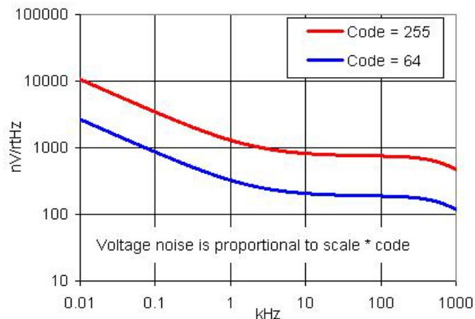
图 11-66. VDAC 电压噪声, 1 V 模式, 高速模式, V_{DDA} = 5\text{ V}
