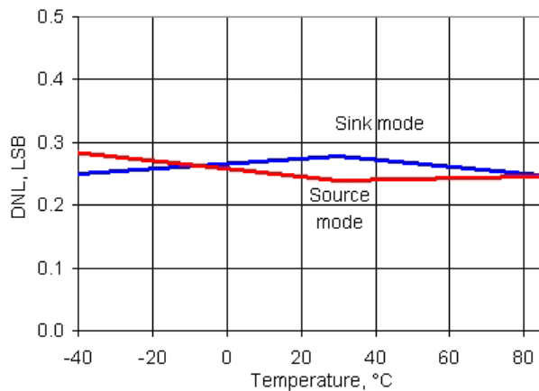
图 11-46. IDAC DNL 与温度，范围 = 255 \mu A，高速模式
