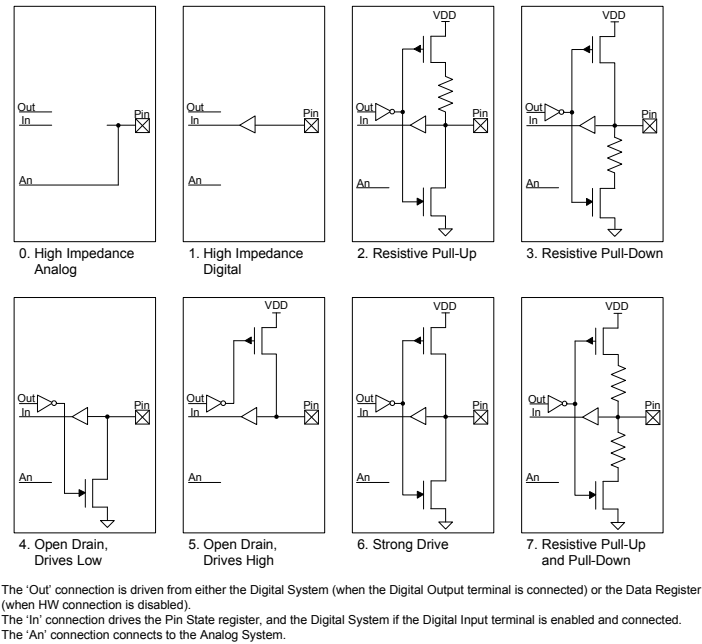
图 6-12. 驱动模式
