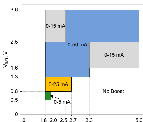
图 11-9. 与 V_{\text{BAT}} 和 V_{\text{OUT}} 相比的 I_{\text{OUT}} 范围
