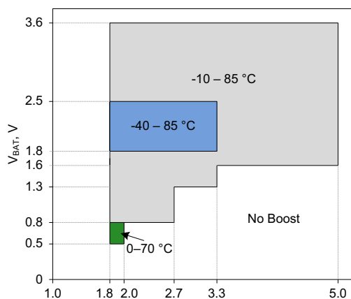
图 11-10. 与 V_{\text{BAT}} 和 V_{\text{OUT}} 相比的 L_{\text{BOOST}} 范围
