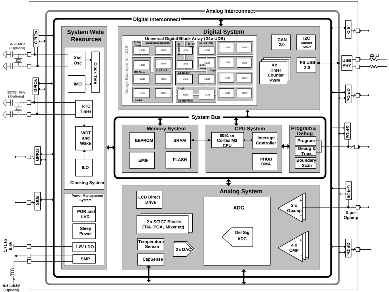
图 1-1. 简化框图
