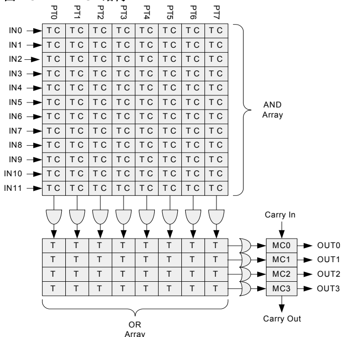
图 7-3. PLD 12C4 结构
