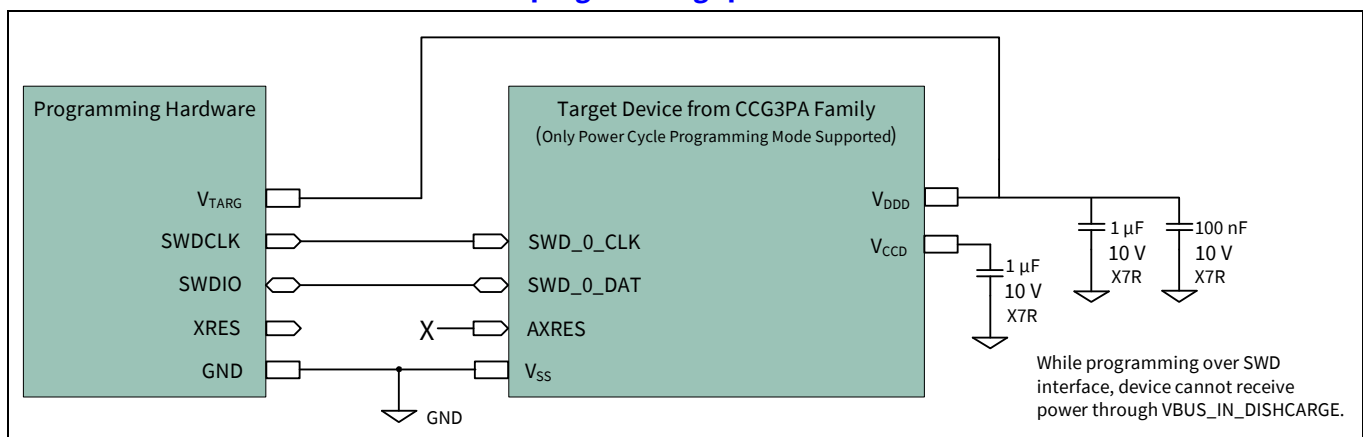
Figure 4 プログラマと CYPD317x デバイスの接続
