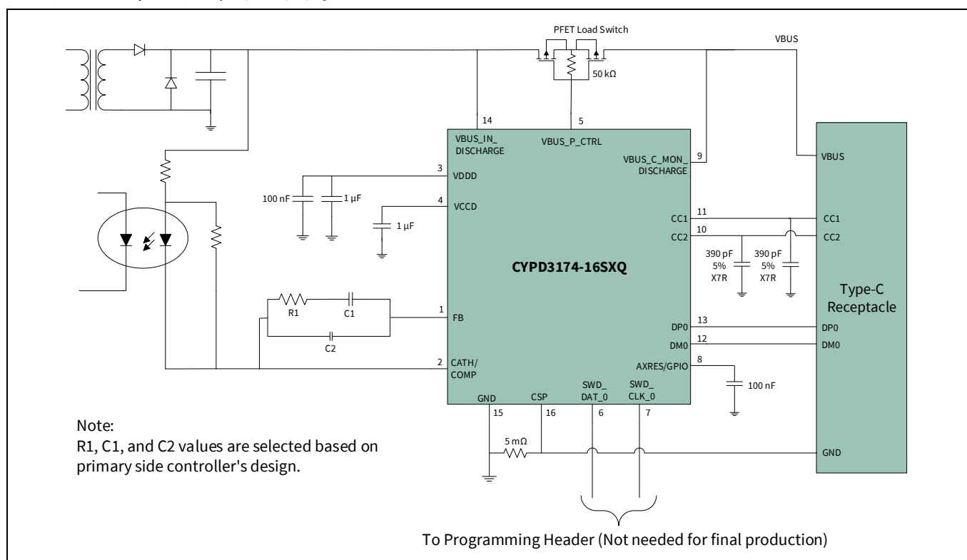
Figure 6 光カプラ フィードバック制御付き CCG3PA ベースの電源アダプタ アプリケーション (16 ピン SOIC デバイス)
