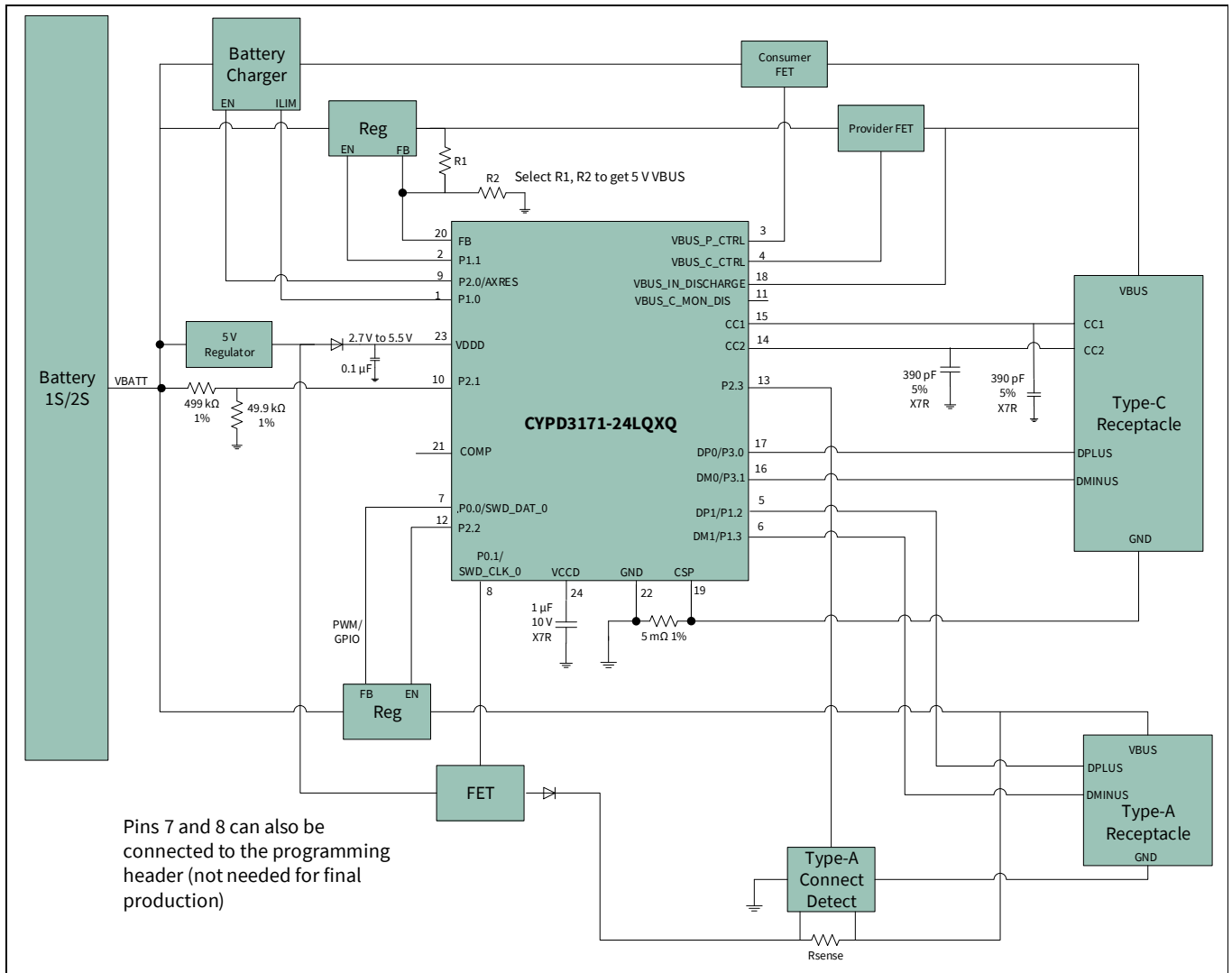
Figure 10 CCG3PA のパワーバンク アプリケーション図
