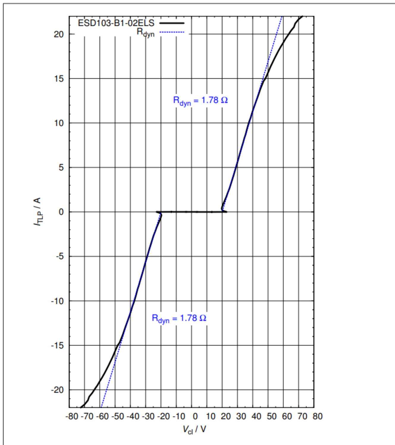
图 8 钳位电压 (TLP): I_{TLP} = f(V_{cl})
