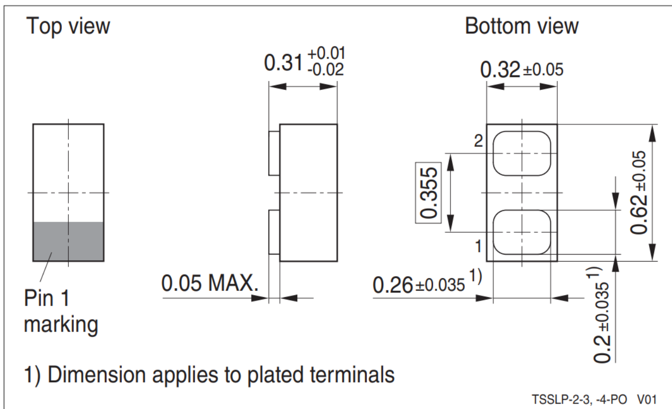
图9 TSSLP-2-4封装
