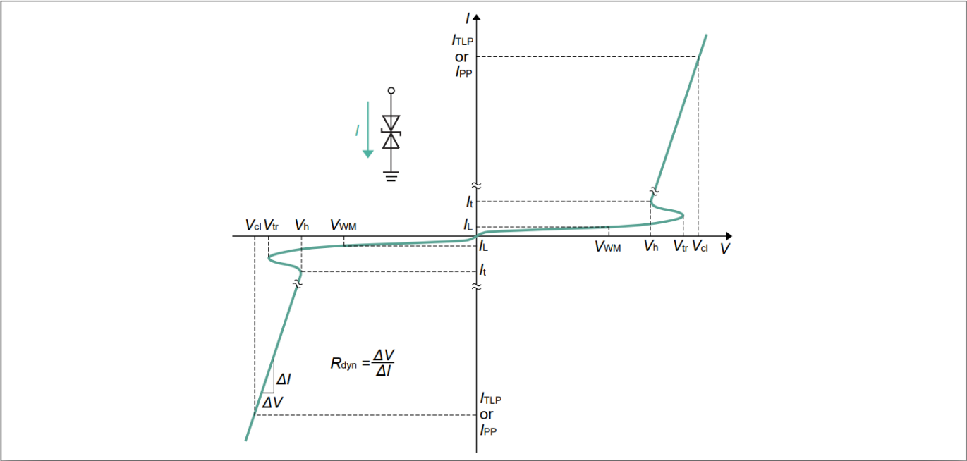
图2 I/V特性曲线
