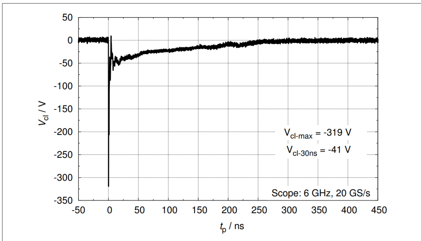
图 7 钳位电压 (ESD): V_{cl} = f(t_p) , 8 kV 负脉冲基于 IEC61000-4-2
