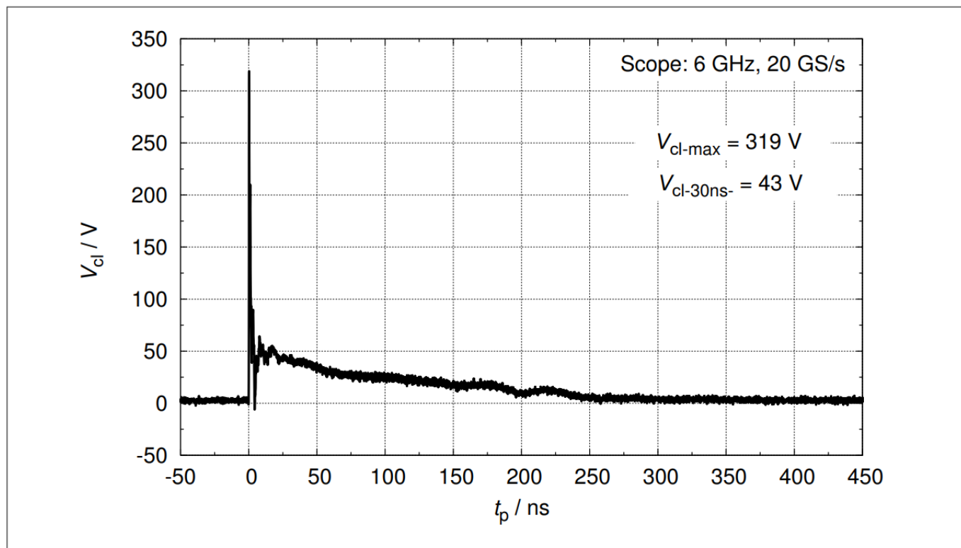
图 6 钳位电压 (ESD): V_{cl} = f(t_p) , 8 kV 正脉冲, 基于 IEC61000-4-2
