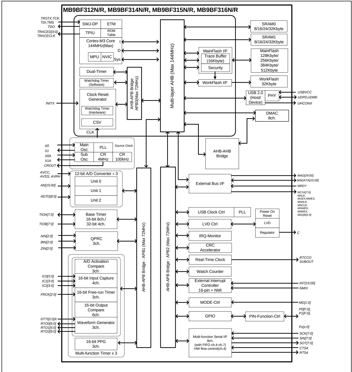
8. 框图
