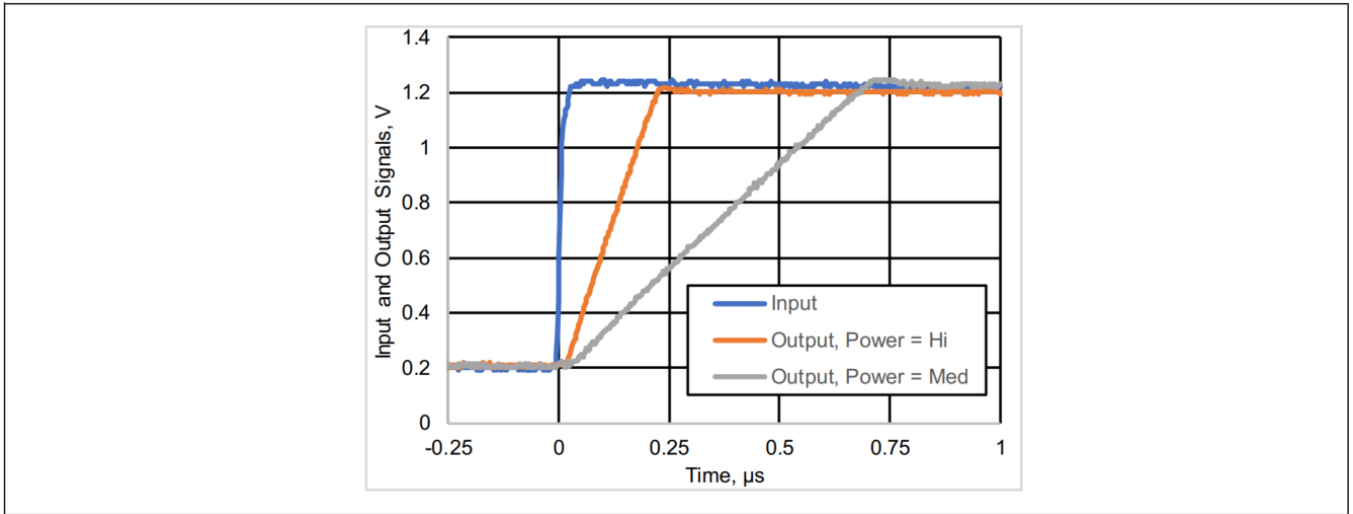
图 17 运算放大器阶跃响应，上升
