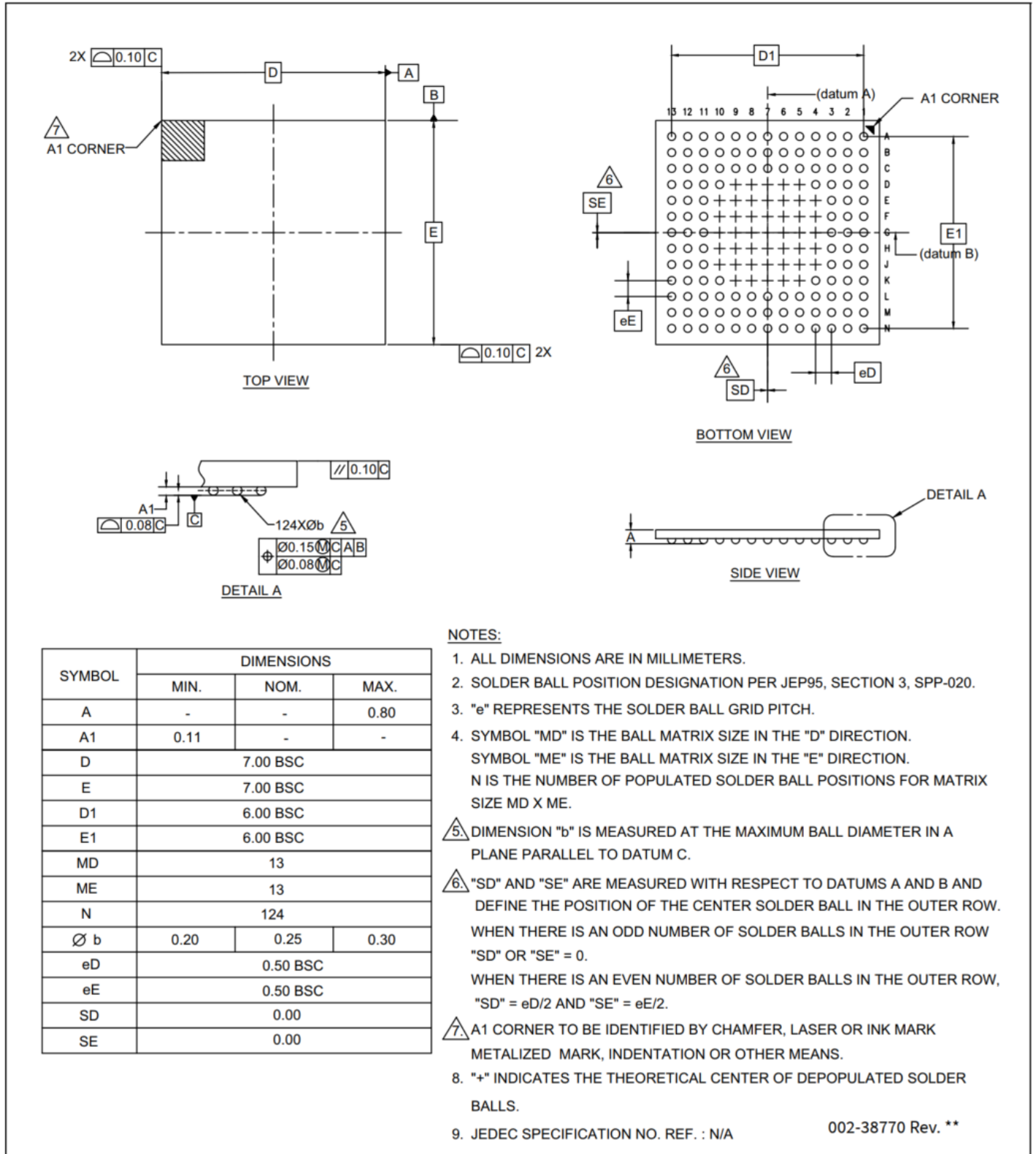
图 20 薄型 124-BGA 7.0 × 7.0 × 0.8 毫米 (PG-WFBGA-124-1)
