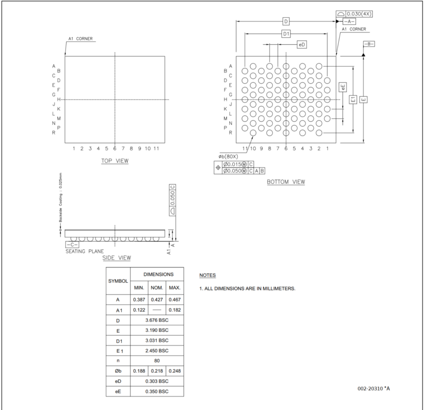
图 21 80-ball WLCSP 3.676 × 3.190 × 0.467 毫米 (SG-XFWLB-80)
