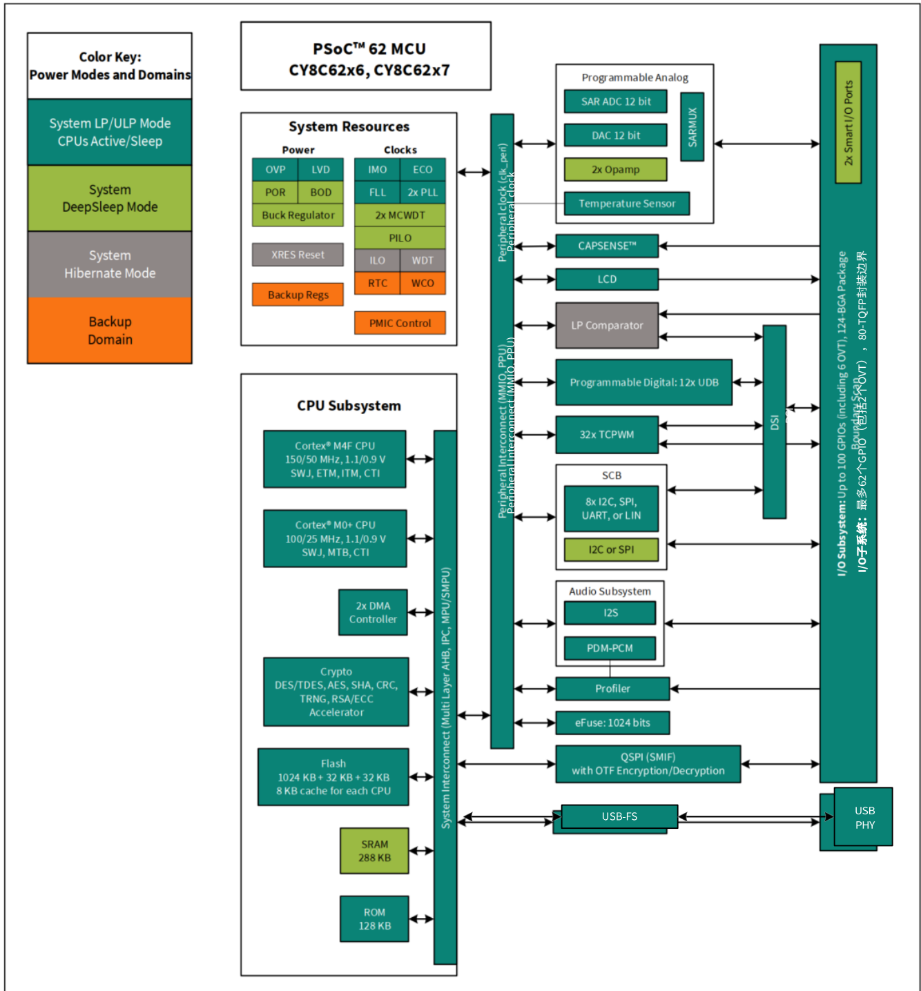
图3 框图
