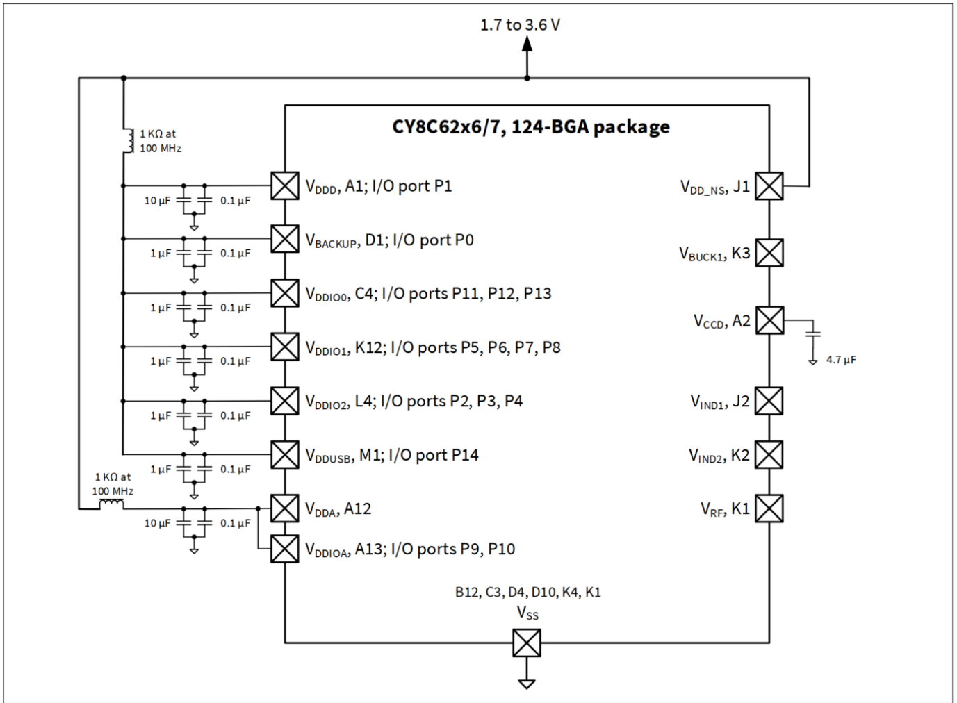
图 12 124-BGA (无降压) 电源连接图
