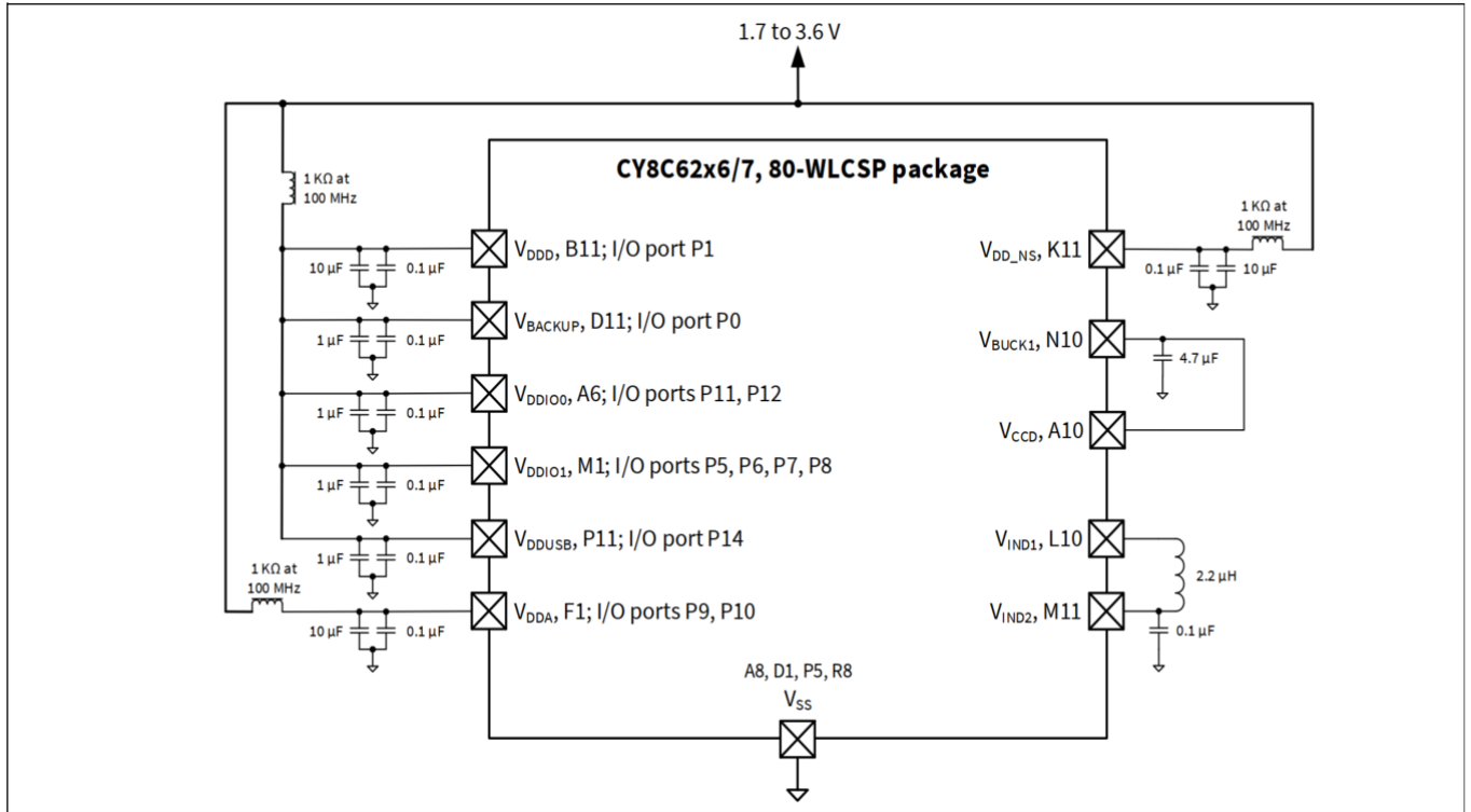
图 13 100-WLCSP电源连接图
