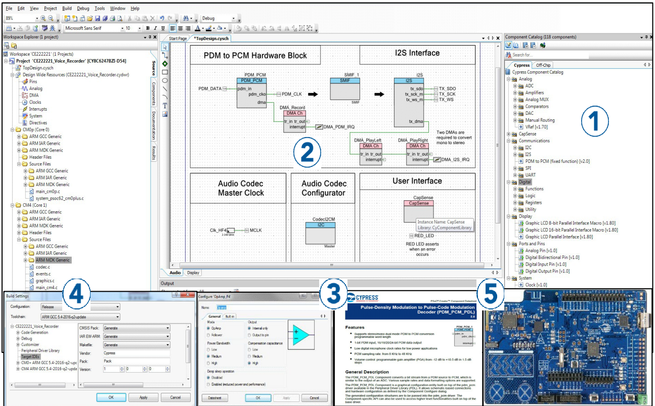
图 2 PSOC™ Creator原理图条目和组件
