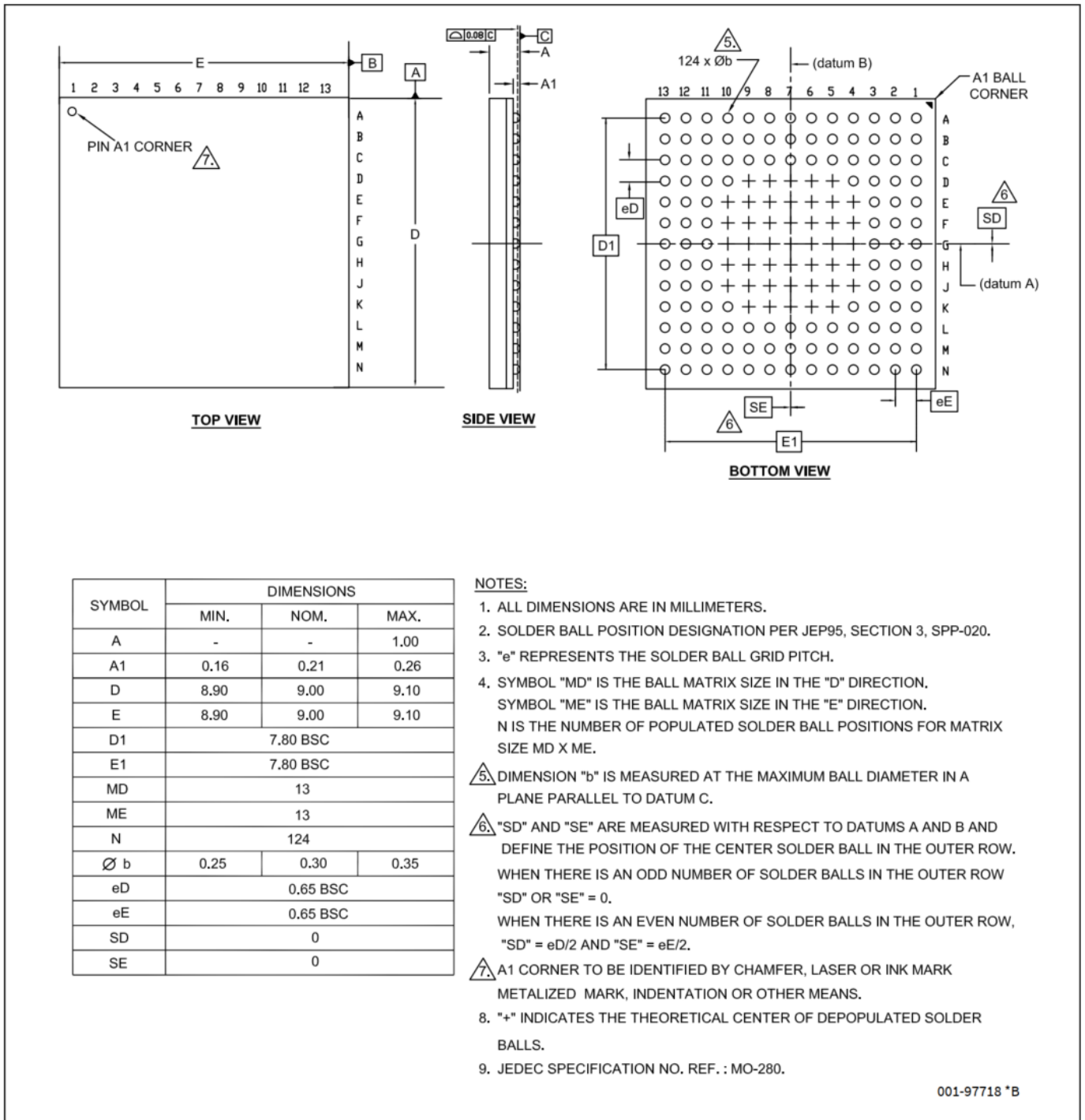
图 19 124-BGA 9.0 × 9.0 × 1.0 毫米, (PG-VBGA-124)
