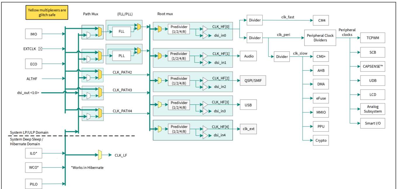
图 4 时钟图
