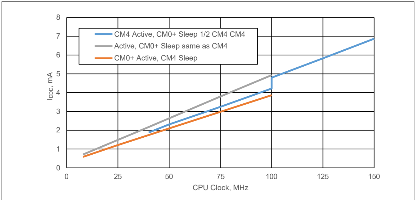
图 16 典型设备电流与 CPU 频率的关系；系统低功耗 (LP) 模式 [5]
