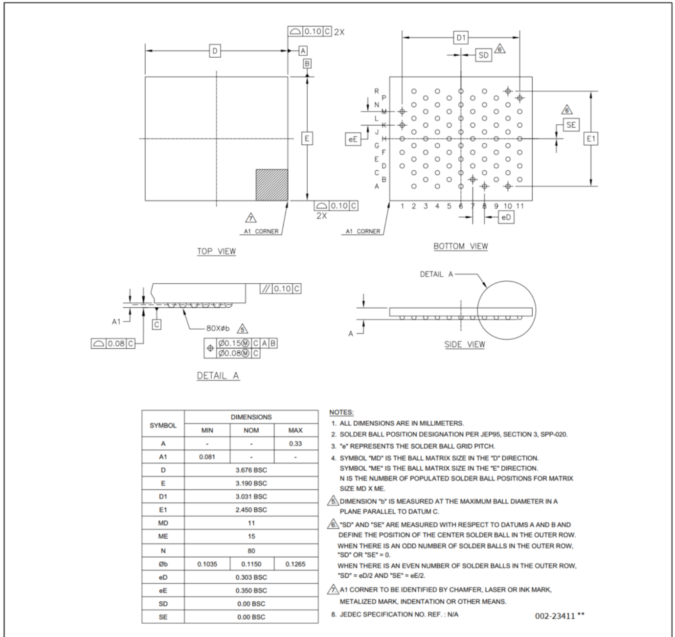
图 22 薄型 80-Ball WLCSP 3.676 × 3.190 × 0.33 毫米 (SG-XFWLB-80)
