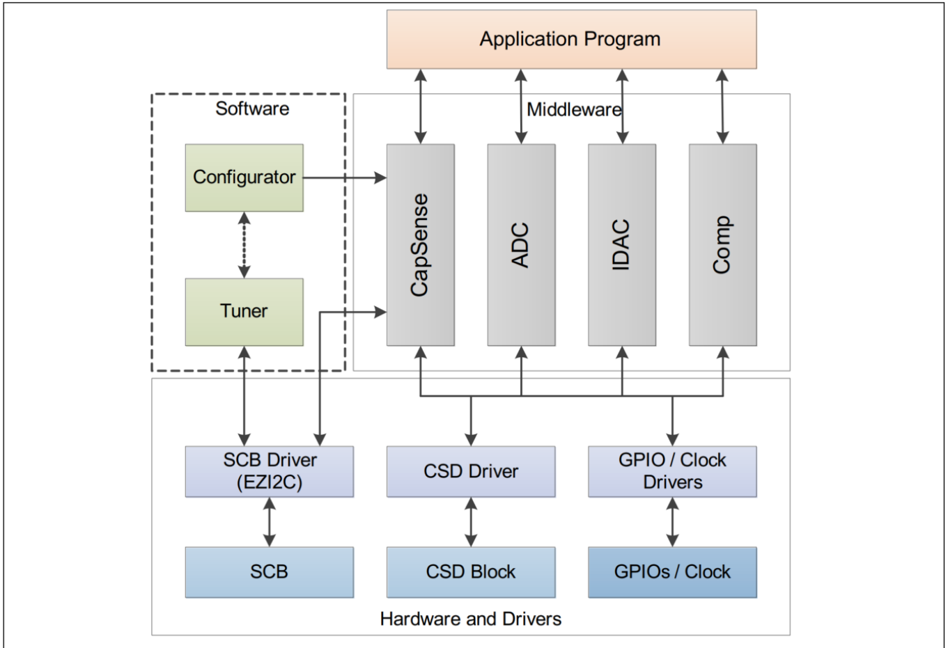
图 10 CAPSENSE™ 软件/硬件子系统
