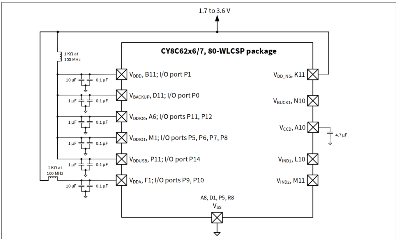
图 14 100-WLCSP (无降压) 电源连接图
