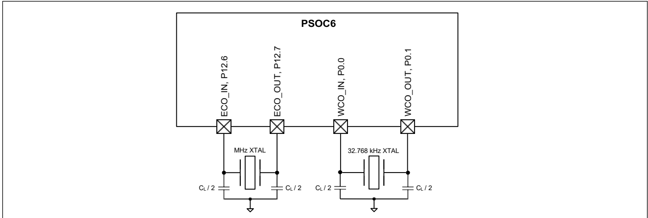
图 5 振荡器电路
