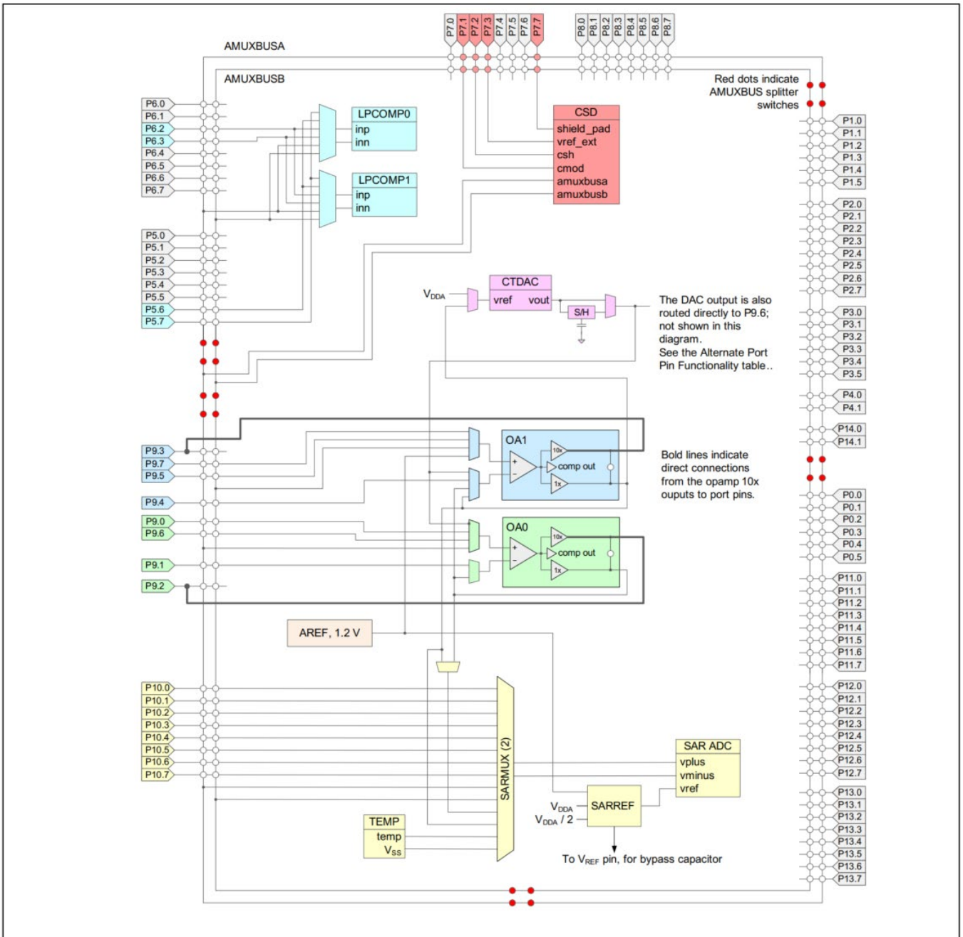
图 7 模拟子系统
