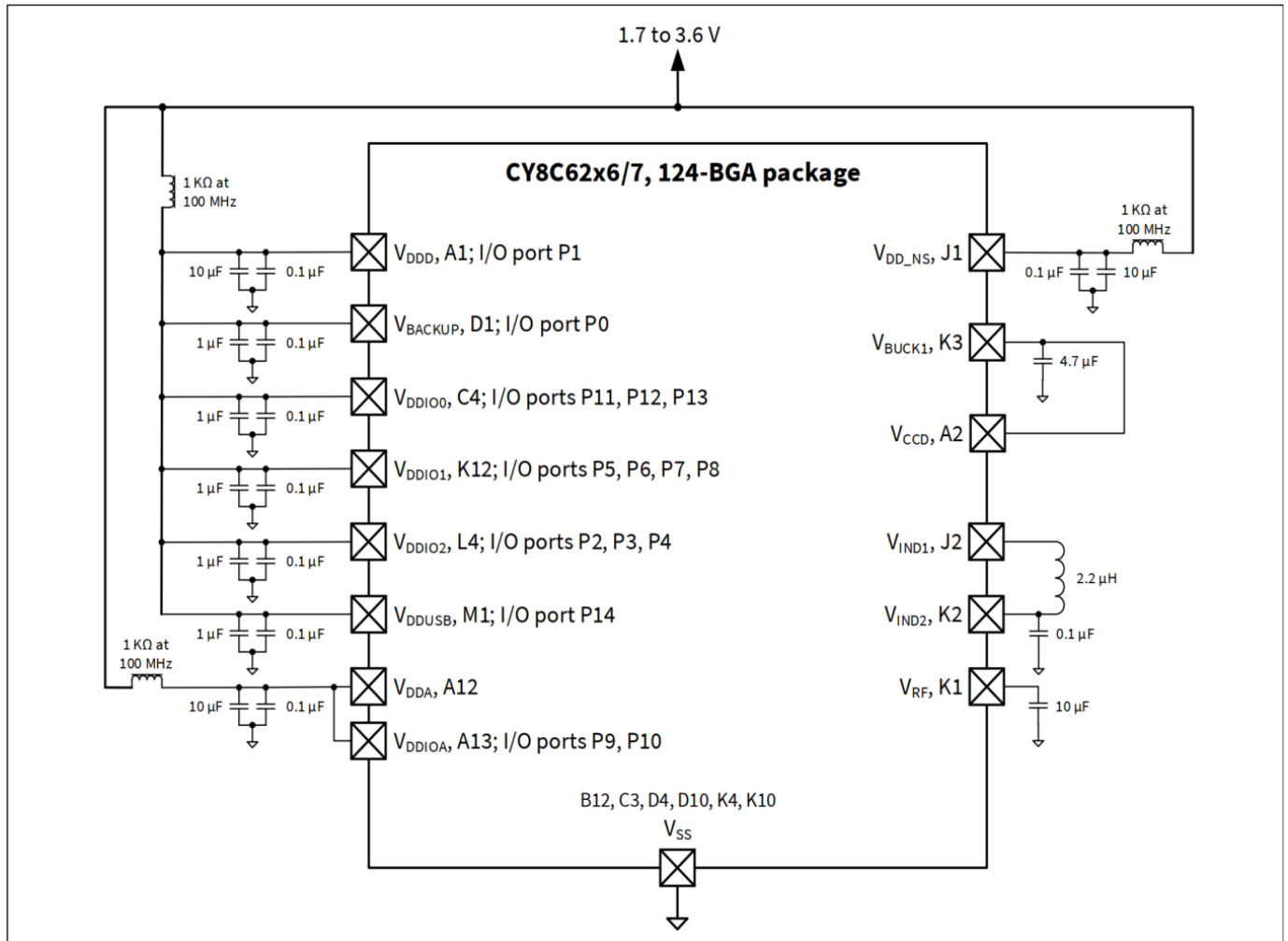
图 11 124-BGA电源连接图
