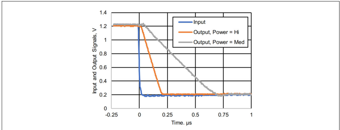
图 18 运算放大器阶跃响应，下降
