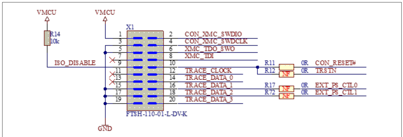
Figure 19 ETM header
