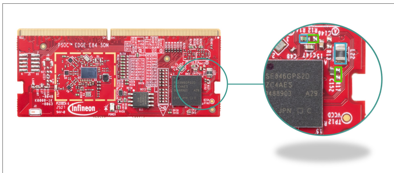
Figure 88 1.8 V VDD Rework 1 on SOM
