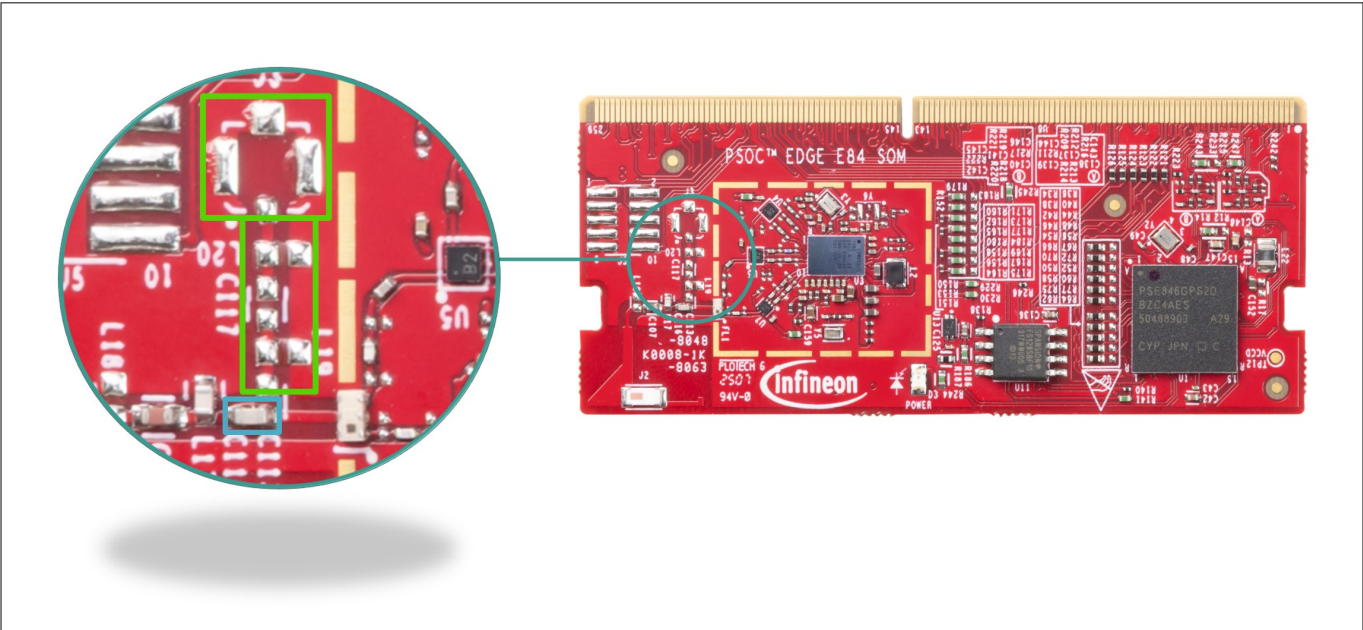
Figure 87 Rework on SoM for enabling external antenna interface
