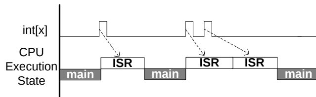
图 4. 边沿触发中断
