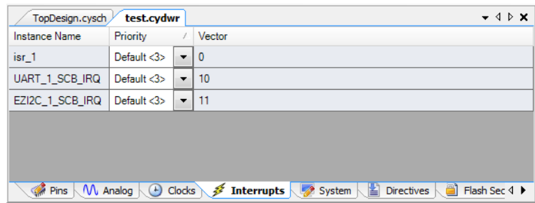
图 13. cydw 窗口中的中断向量编号
