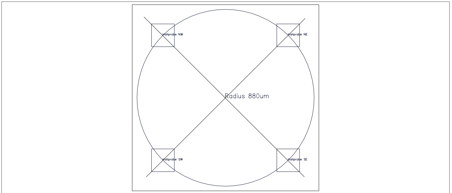
图 28 TLE49SR 霍尔元件半径
