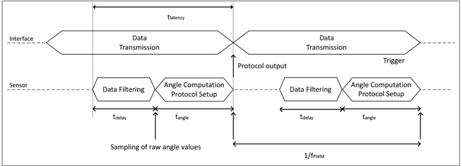
图 4 PWM 接口时序概览
