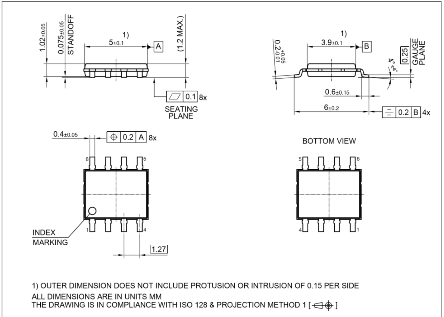
图 25 PG-TDSO-8-1 封装图
