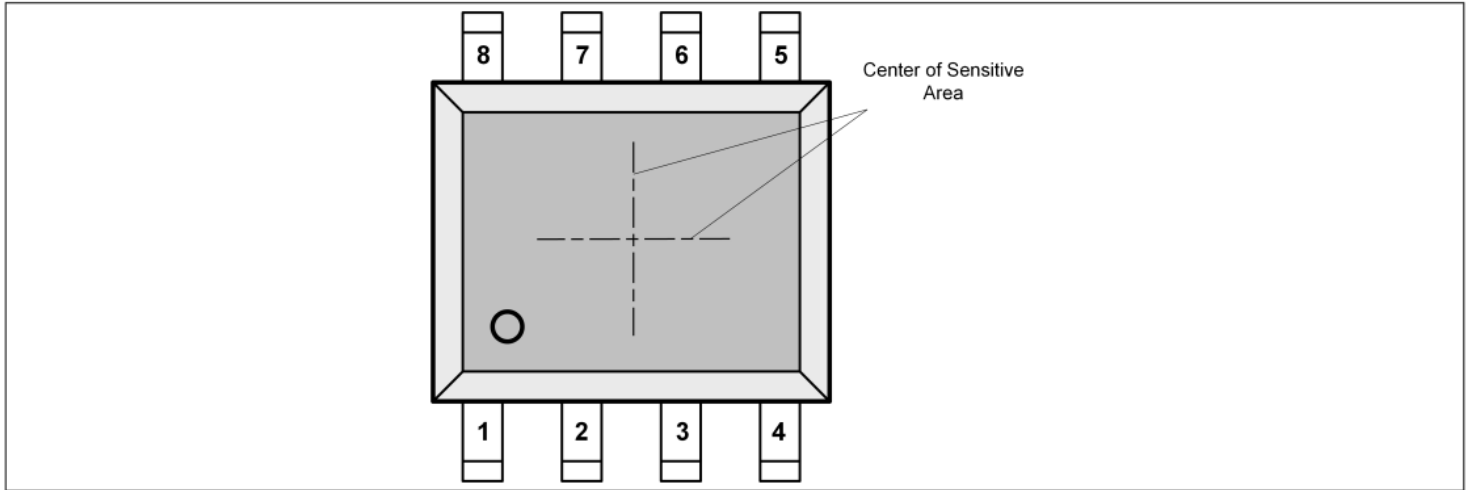
图2 引脚配置 (顶视图)
