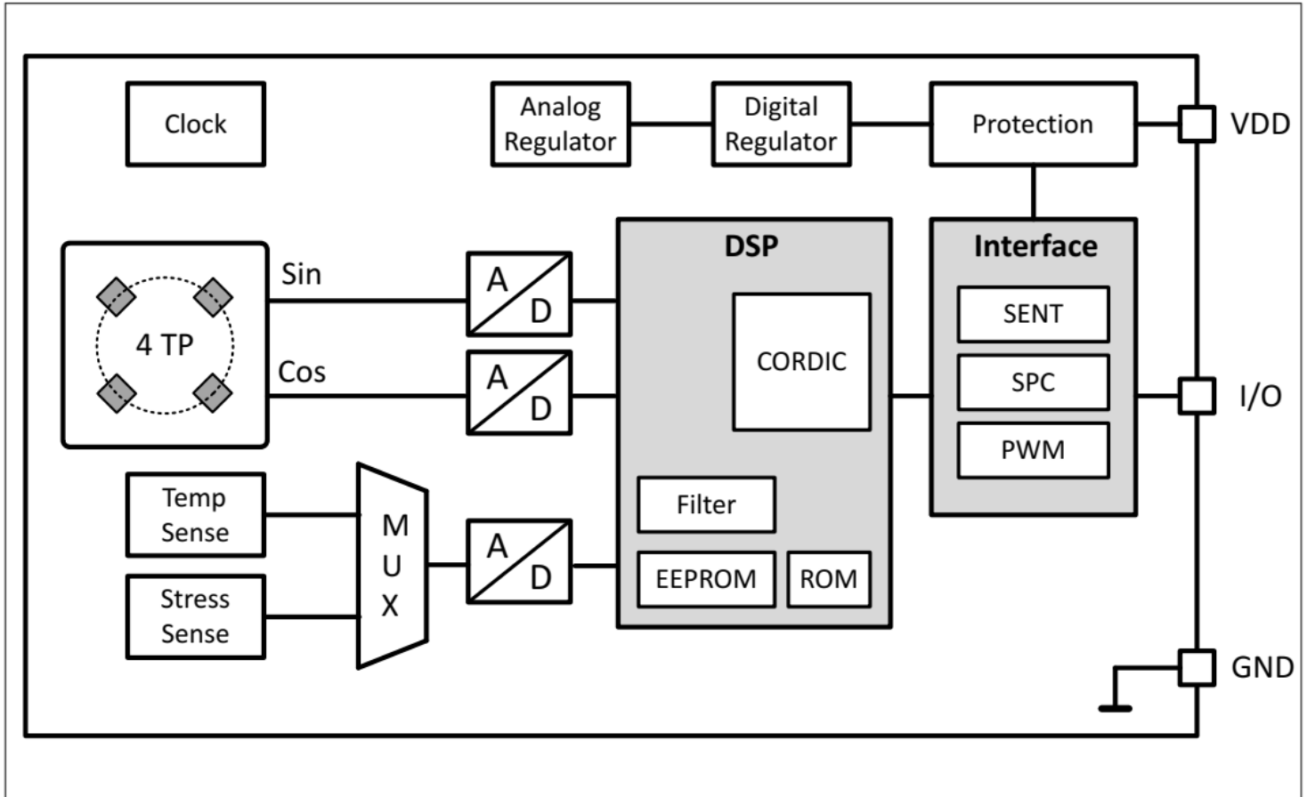
图 1 TLE49SR 的功能框图
