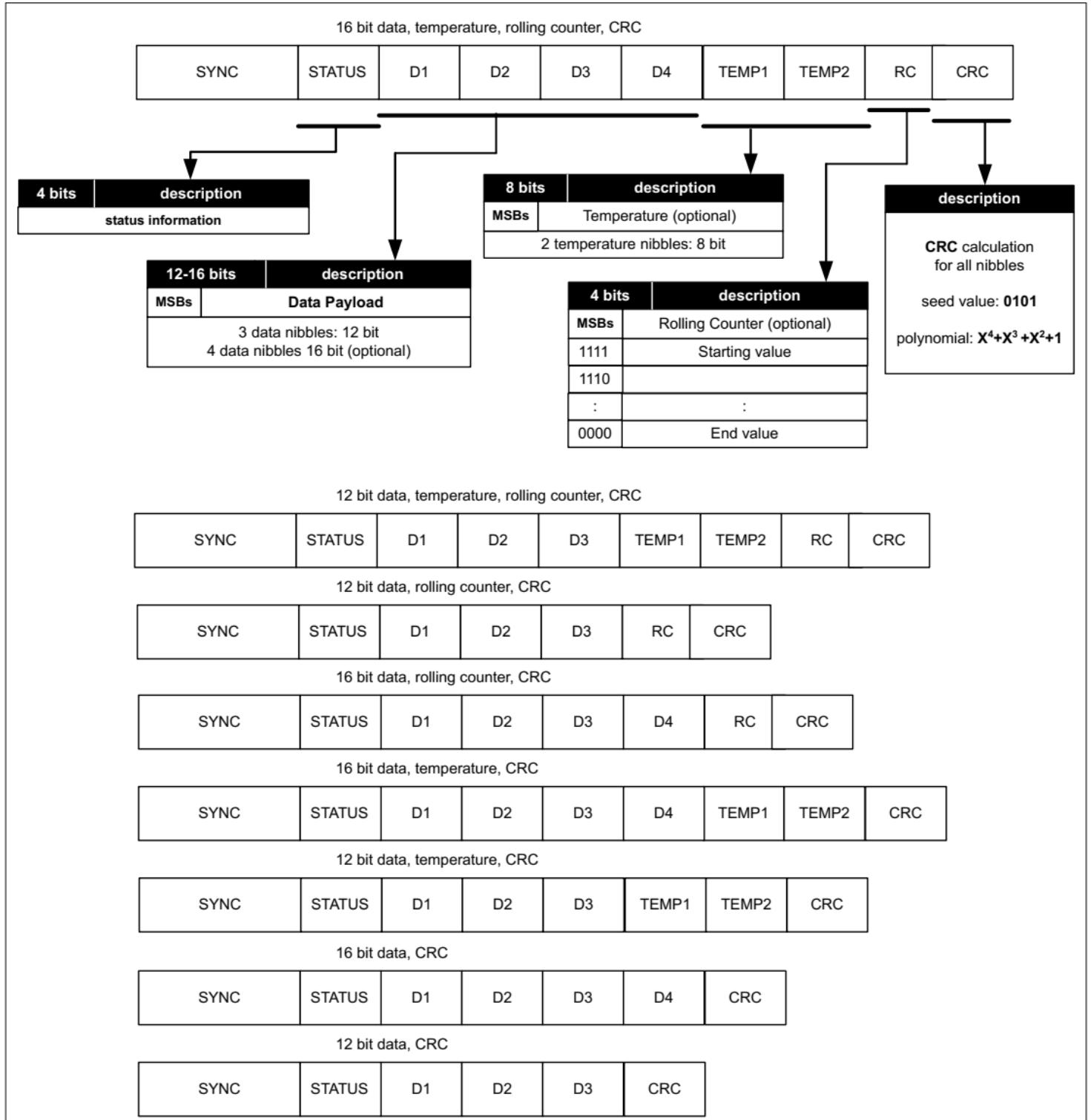
图 12 SENT 帧选项
