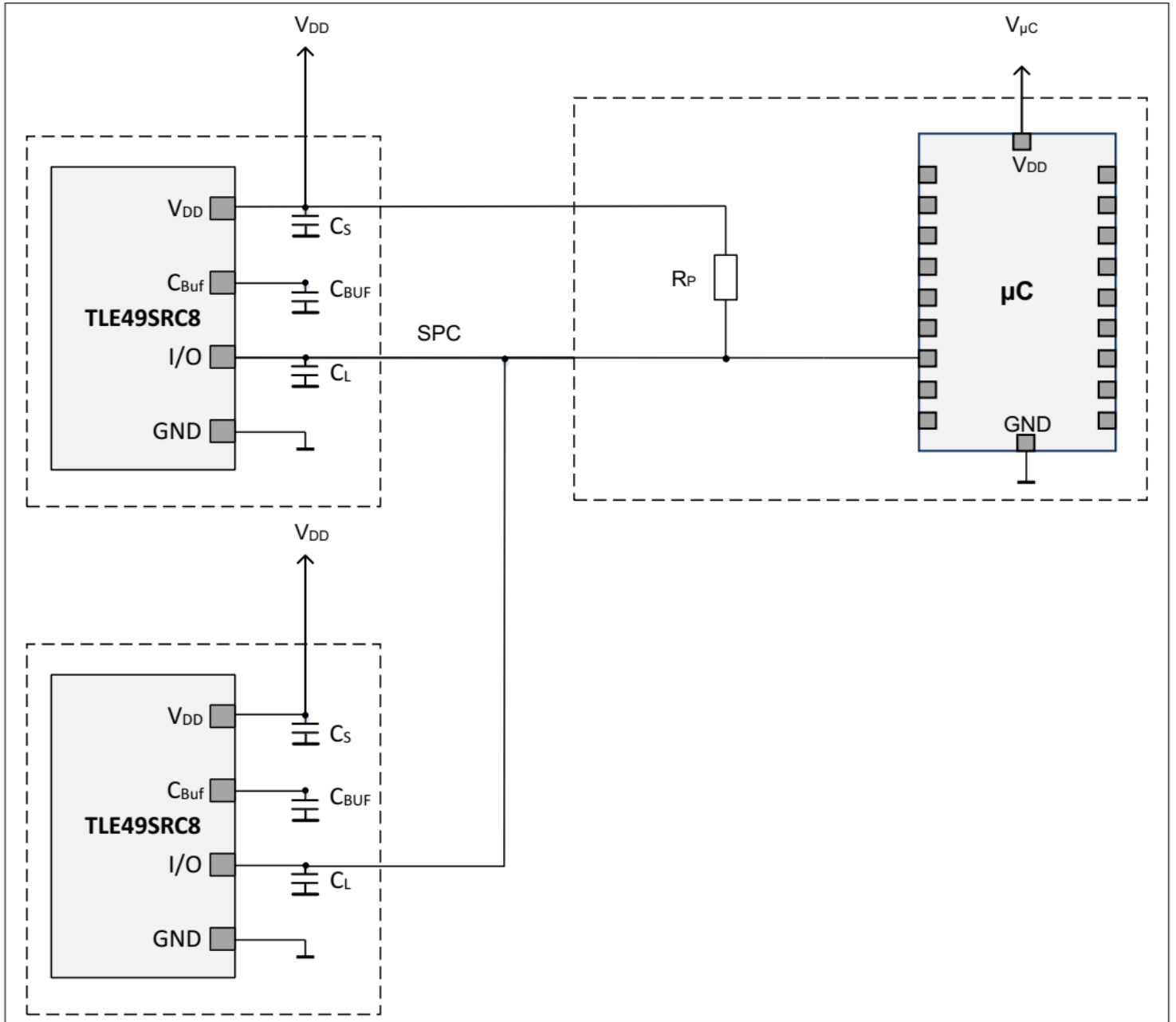
图 23 SPC 接口的应用电路
