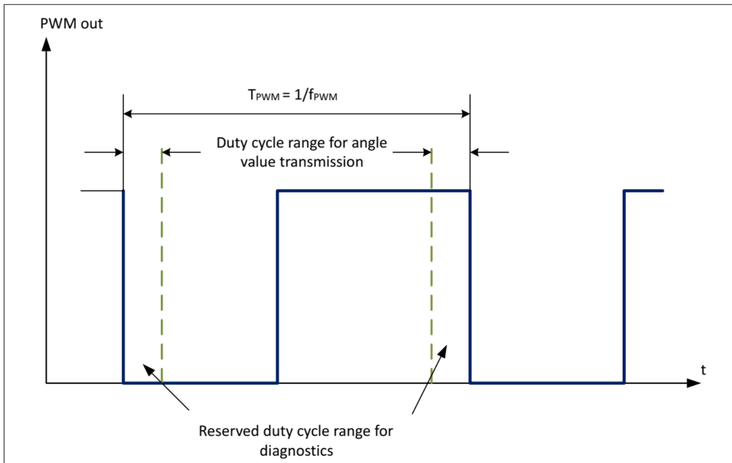
图 8 PWM 接口，占空比范围从上升沿开始
