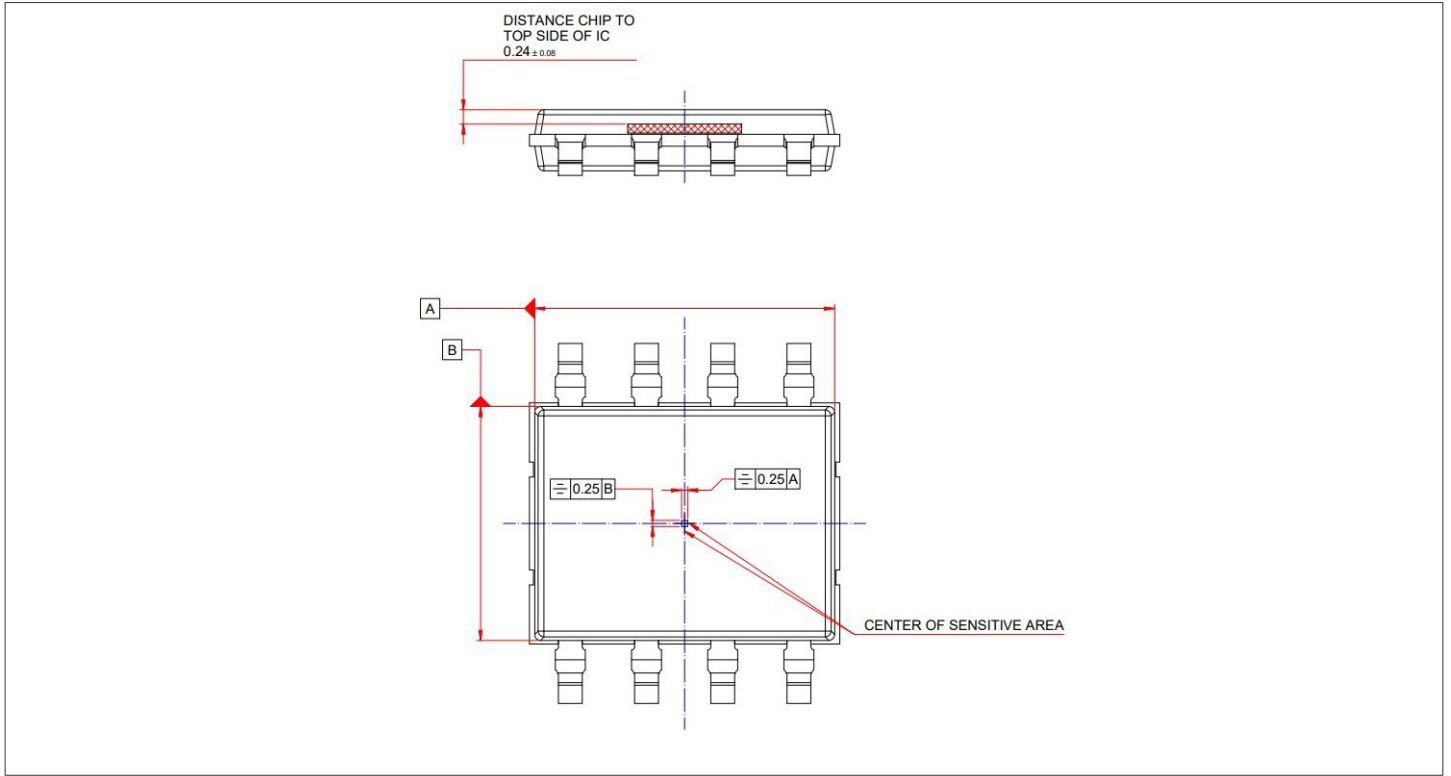
图 27 PG-TDSO-8-1 敏感区中心
