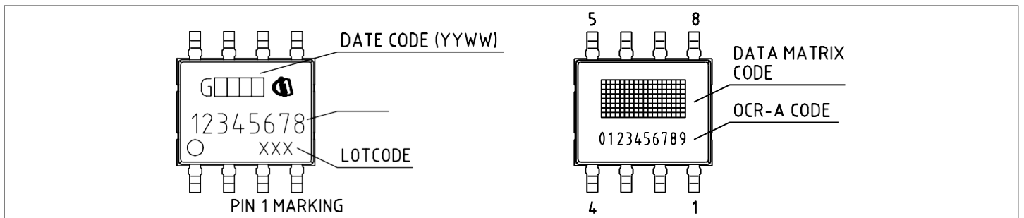
图 26 PG-TDSO-8 封装标记
