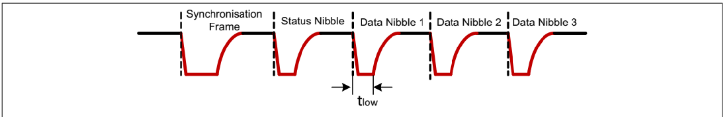
图 11 SENT 半字节低电平时间
