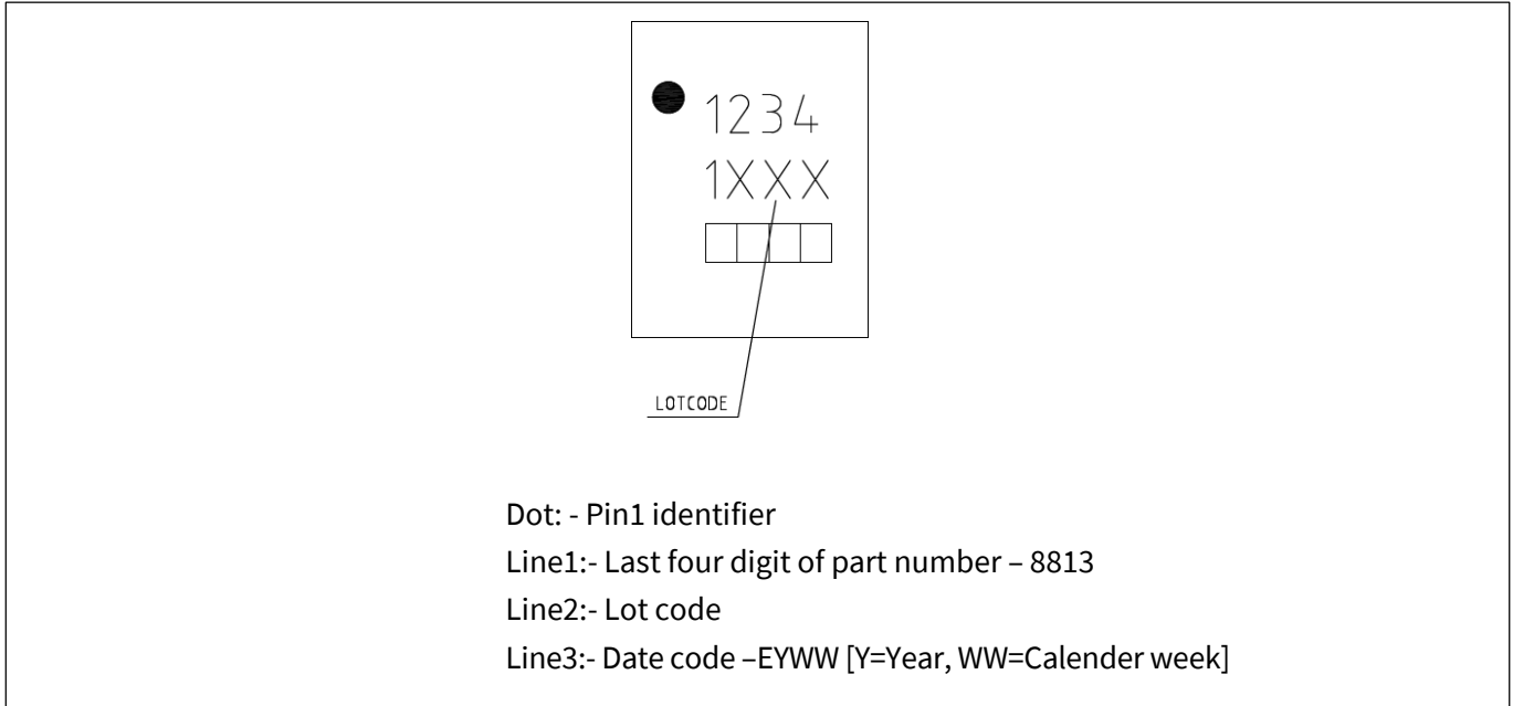
图 28 封装标记
