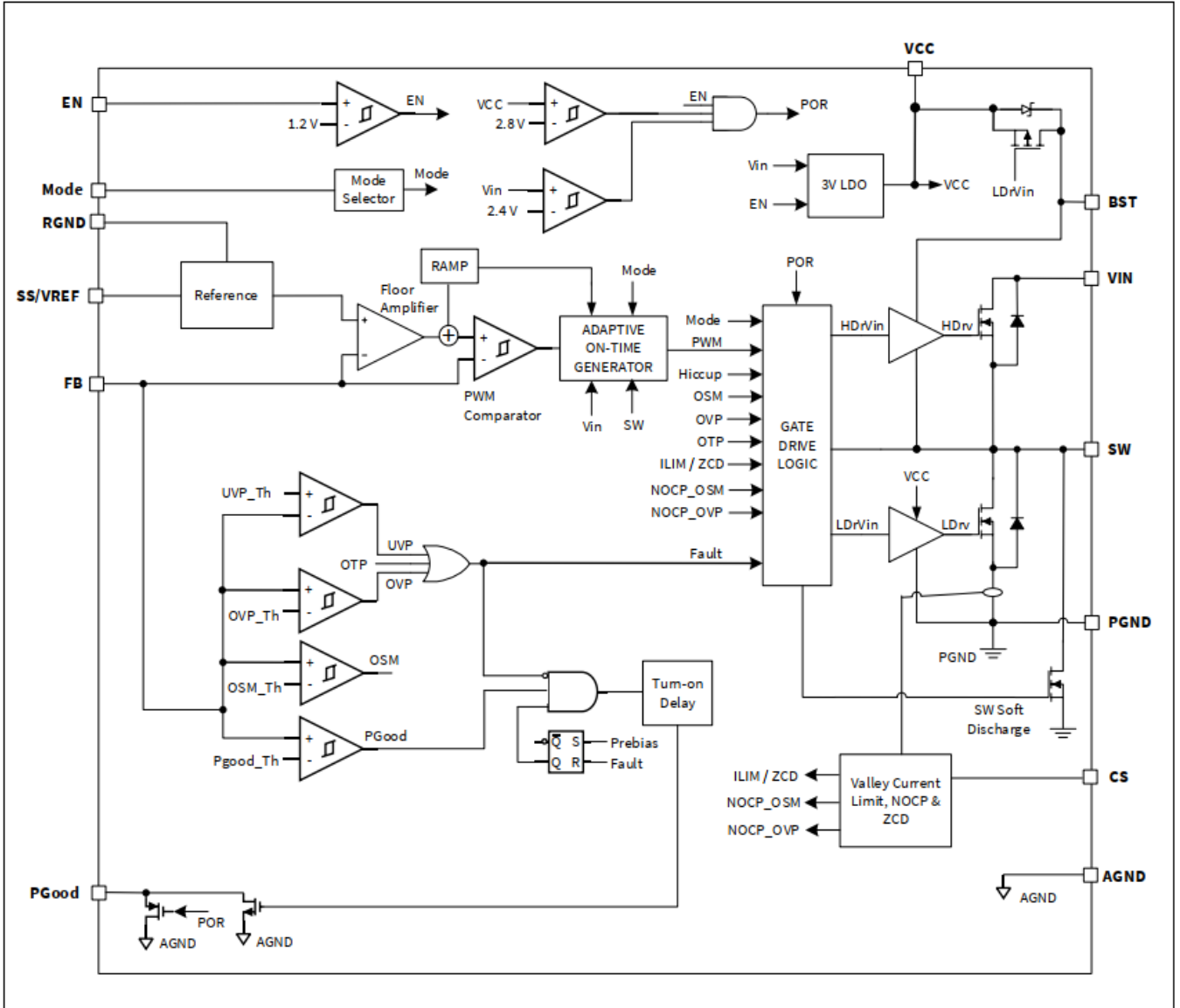
图 2 框图
