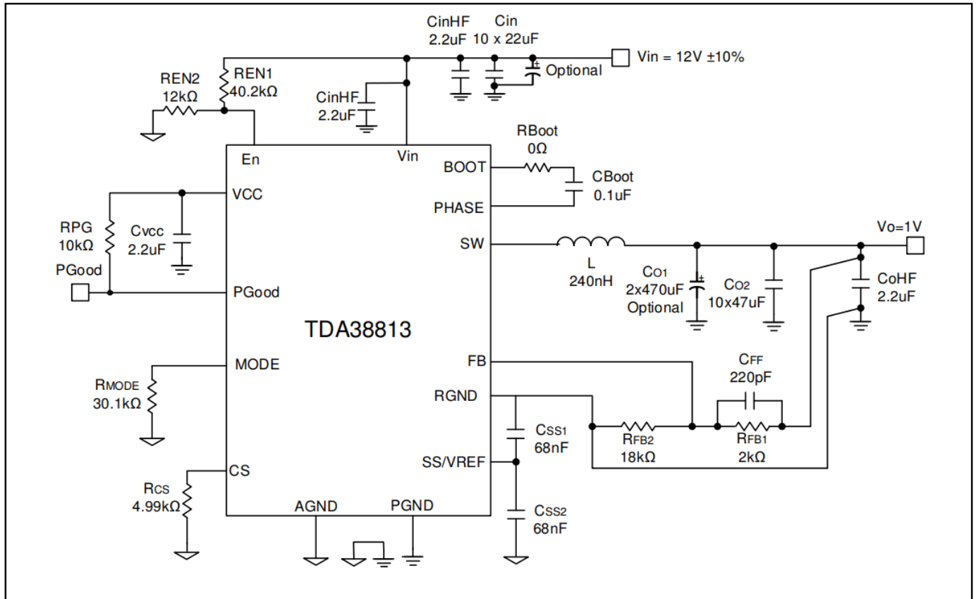
图 13 TDA38813 的典型应用图。Vin = 12 V, Vo = 1V, Io = 12 A, Fsw = 800 kHz。
