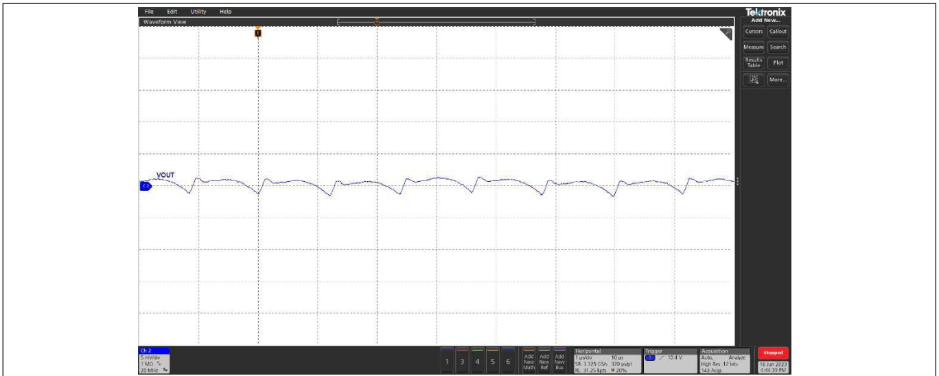
图 16 12A 负载时的输出电压纹波, F_{sw} = 800 \text{ kHz} ,（通道 2: Vo）
