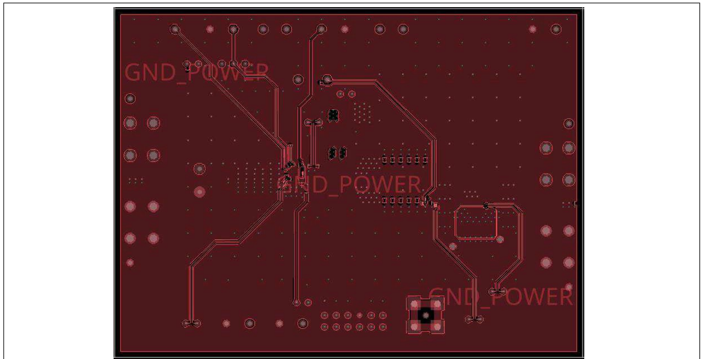
图 24 TDA38813 演示板 - 第 3 层 (接地& 信号)
