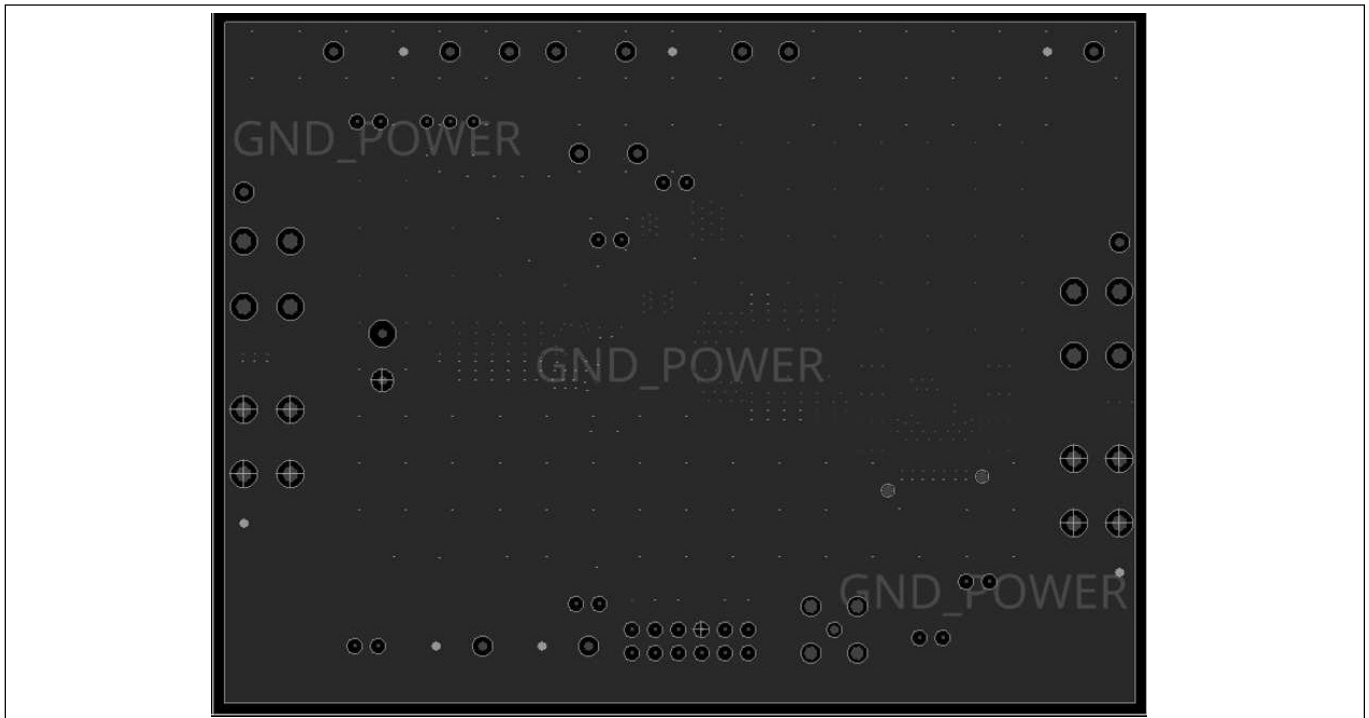
图 26 TDA38813 演示板 - 第 5 层 (接地)
