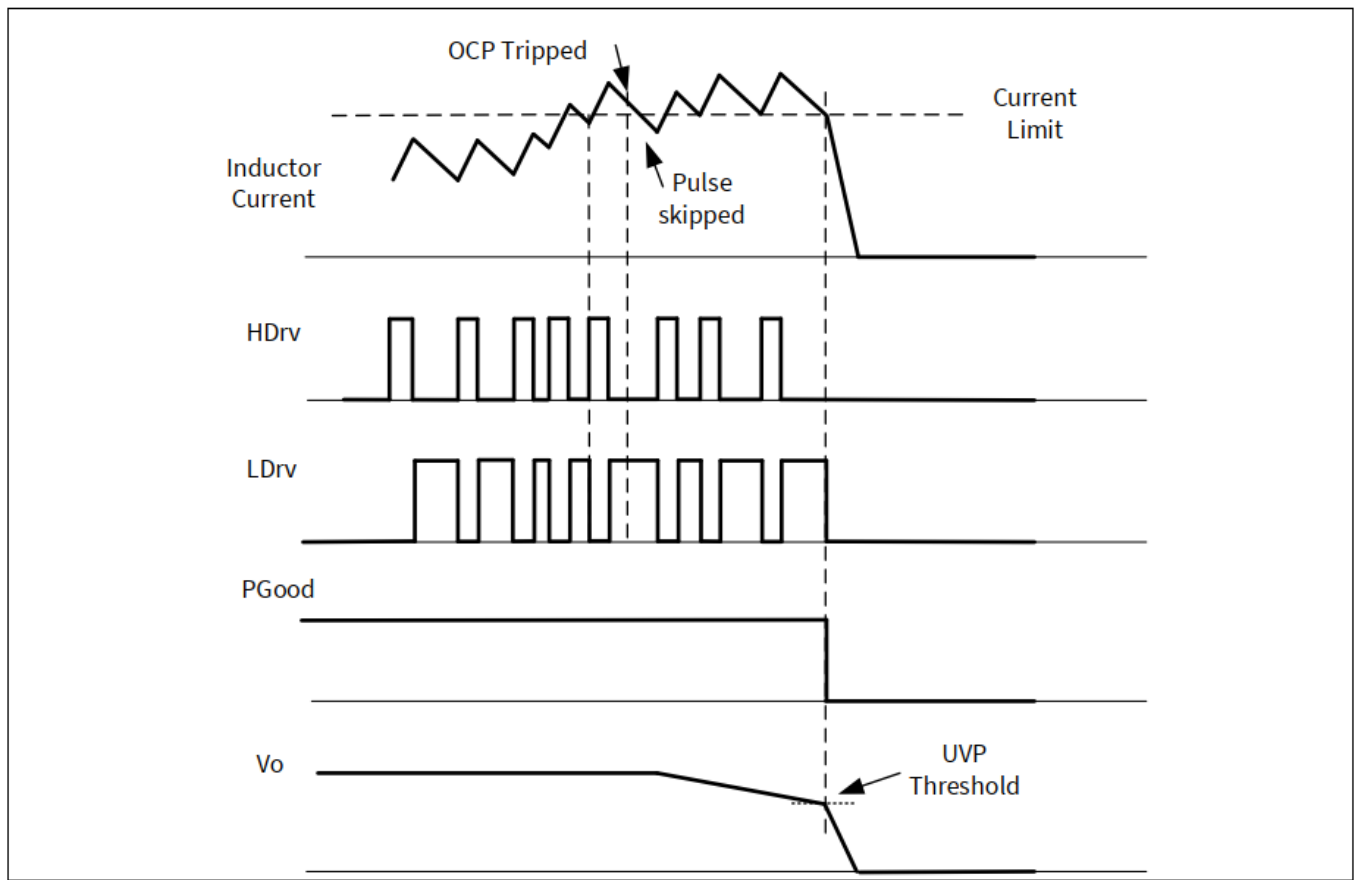
图 11 逐周期 OCP 响应
