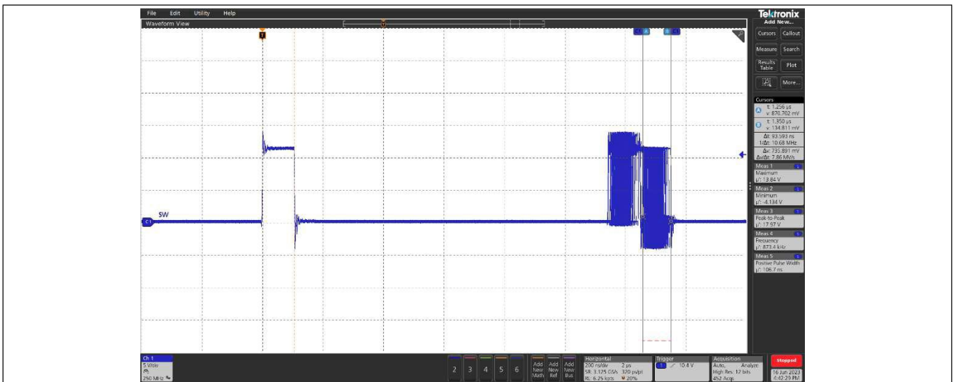
图 17 SW 节点抖动, 12A 负载, F_{sw} = 800 \text{ kHz}
