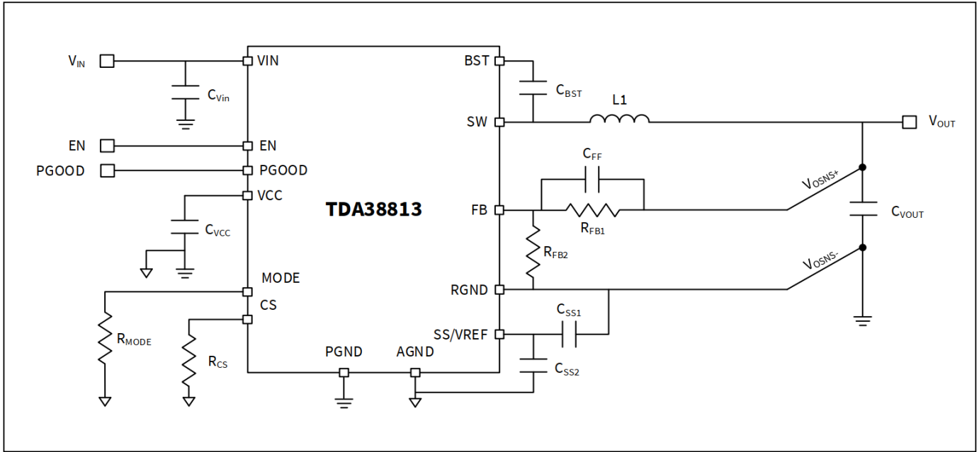
图3 TDA38813 应用电路
