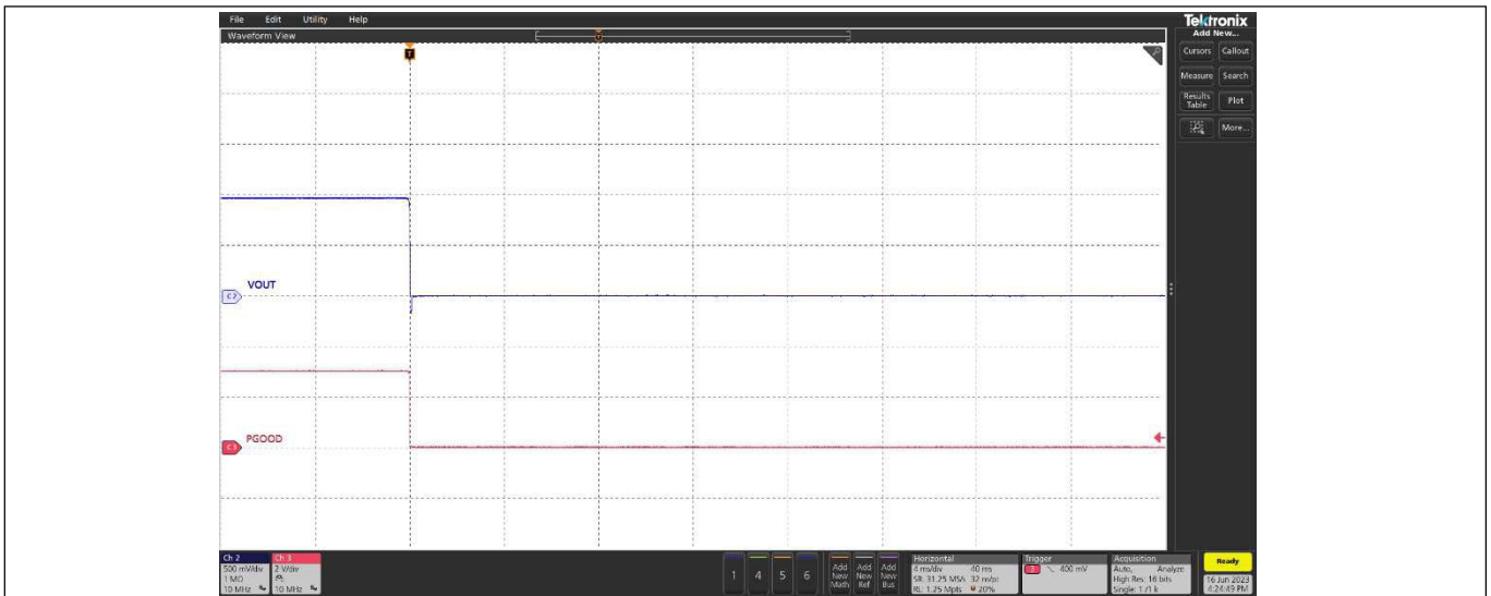
图 19 短路和 UVP (关断), (通道2: Vo, 通道3: PGood)
