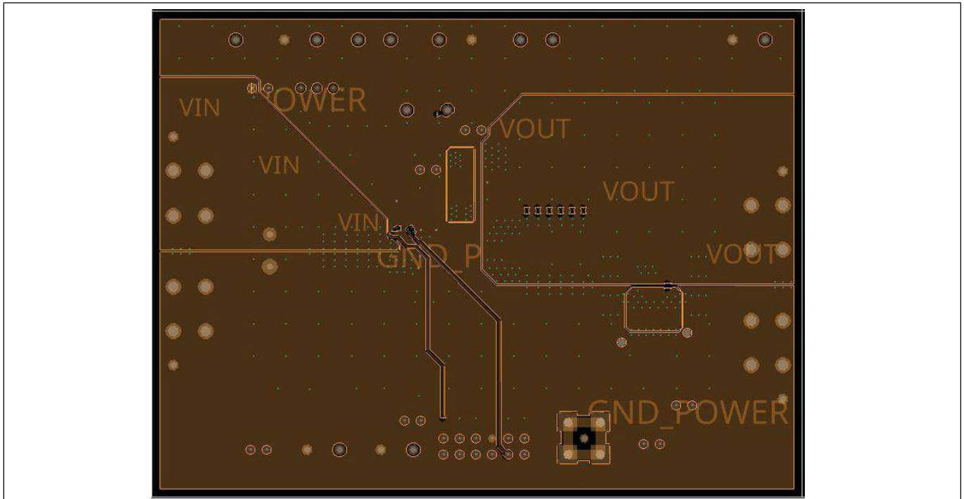
图 25 TDA38813 演示板 - 第 4 层 (接地&amp; 信号)
