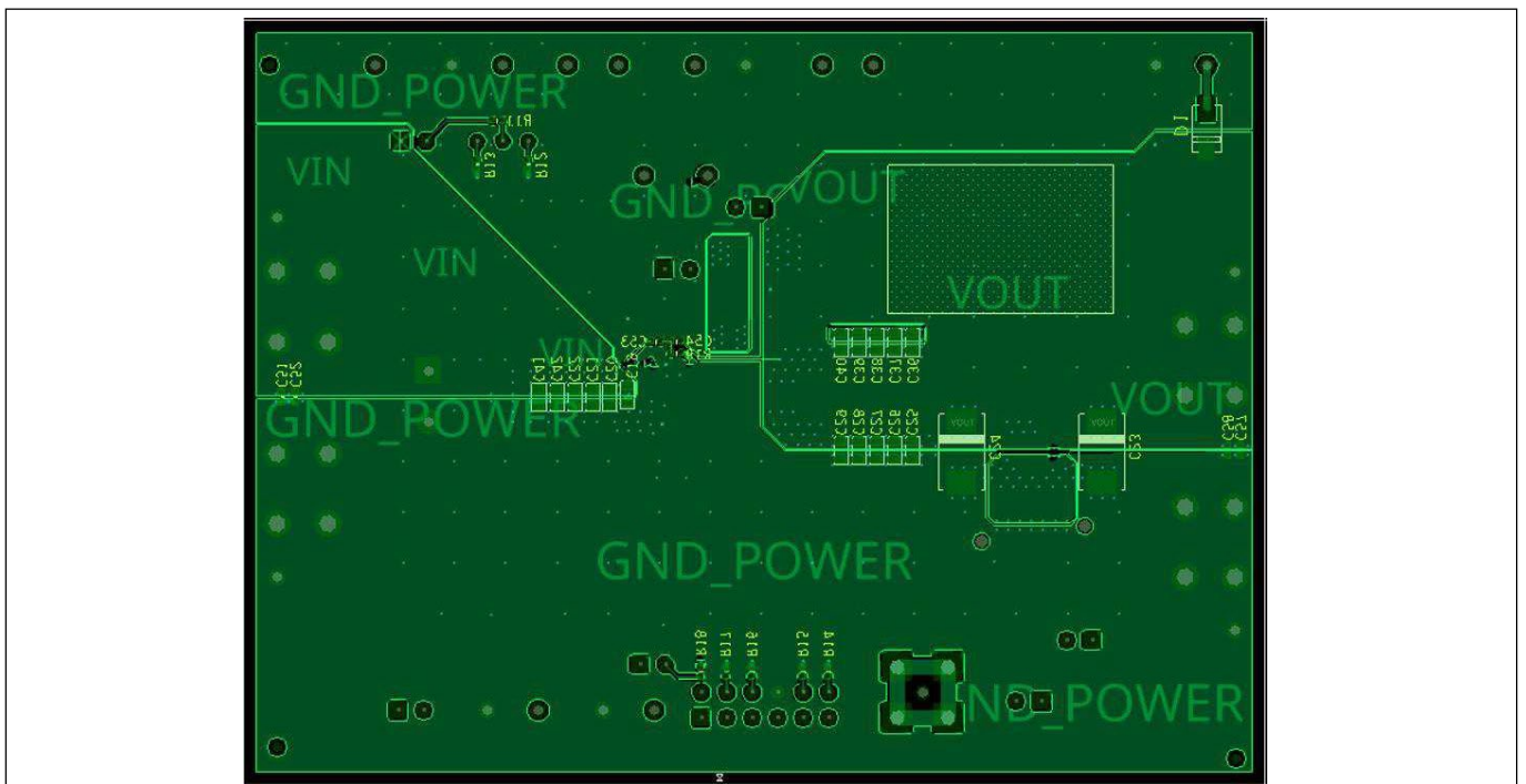
图 22 TDA38813 演示板 - 底层
