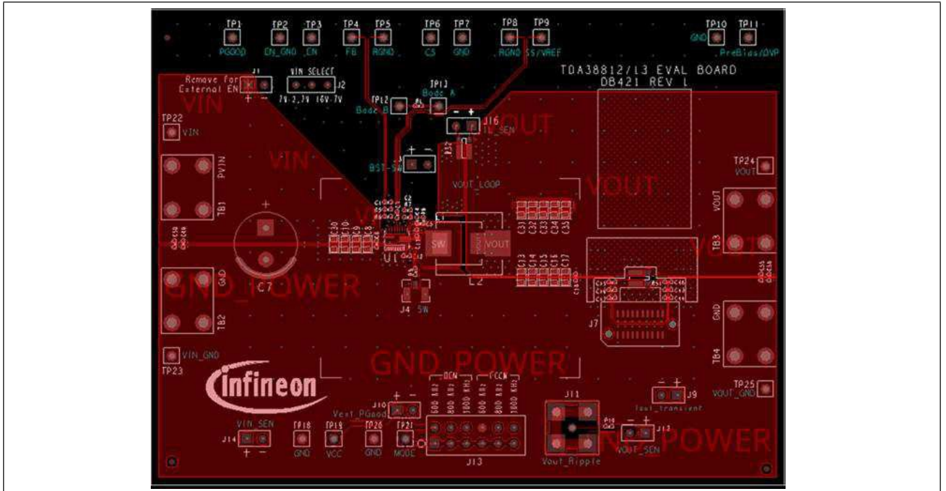
图 21 TDA38813 演示板 - 顶层
