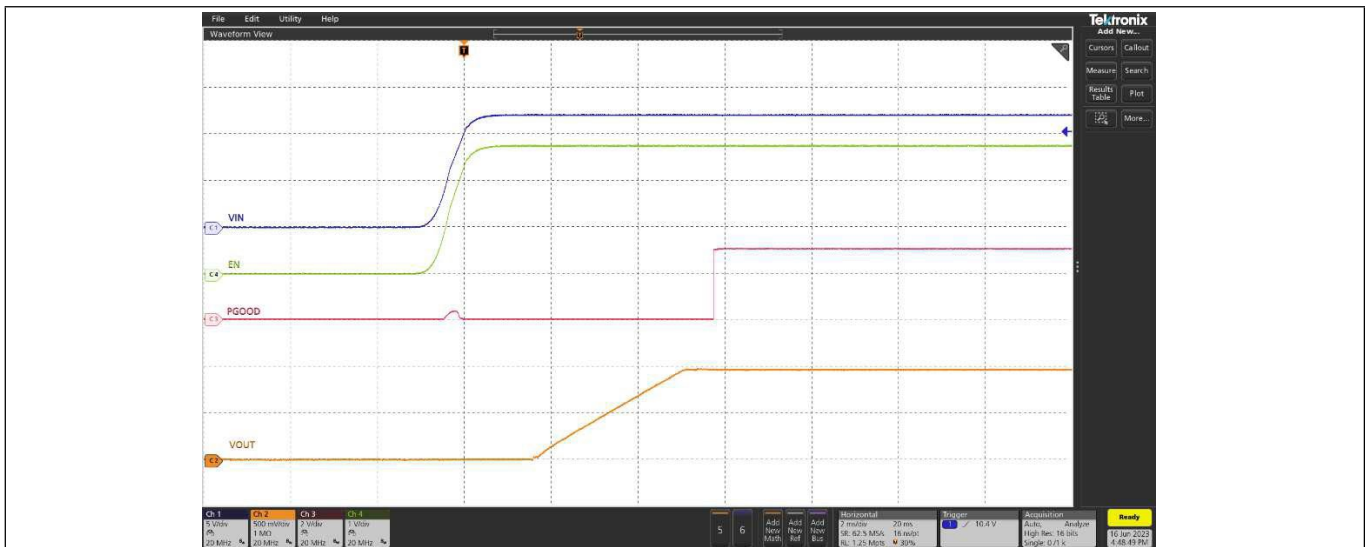
图 14 12 A 负载时的启动, (通道 1: Vin, 通道 2: Vout, 通道 3: PGood, 通道 4: 使能)
