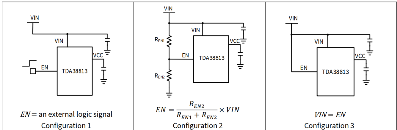
图 8 使能配置
