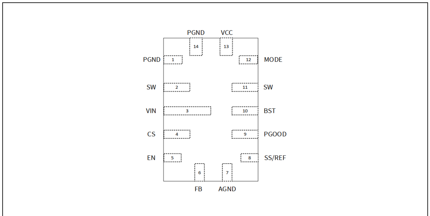
图 1 封装俯视图 - TDA38807
