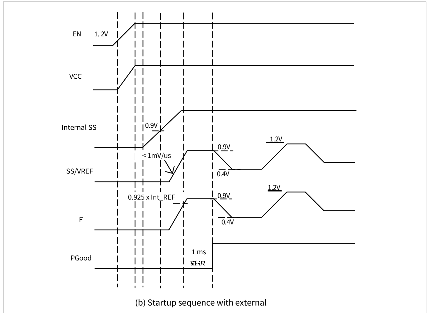
图 5 采用电压跟踪和外部基准的启动顺序
