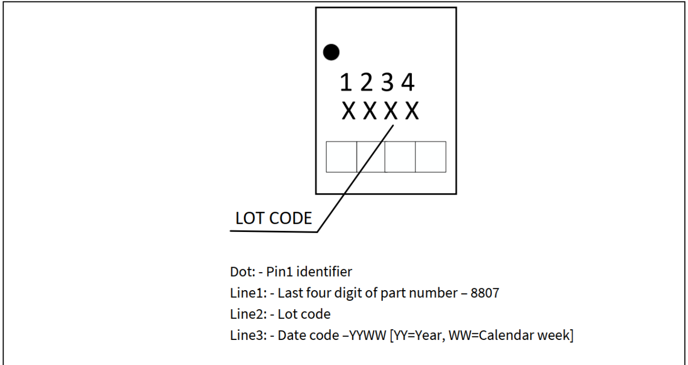
图 15 封装标记
