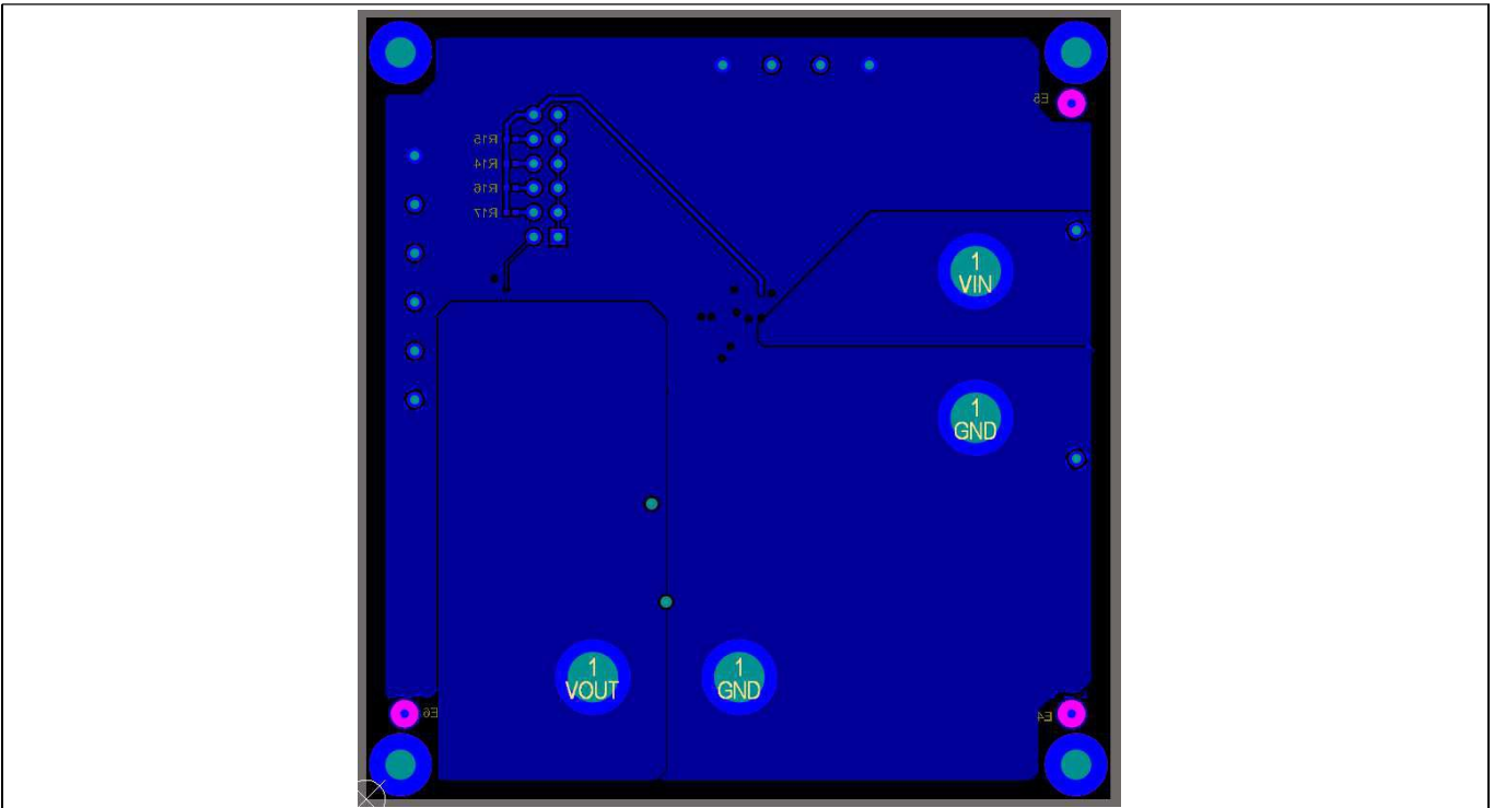
图 11 TDA38807 演示板 - 底层
