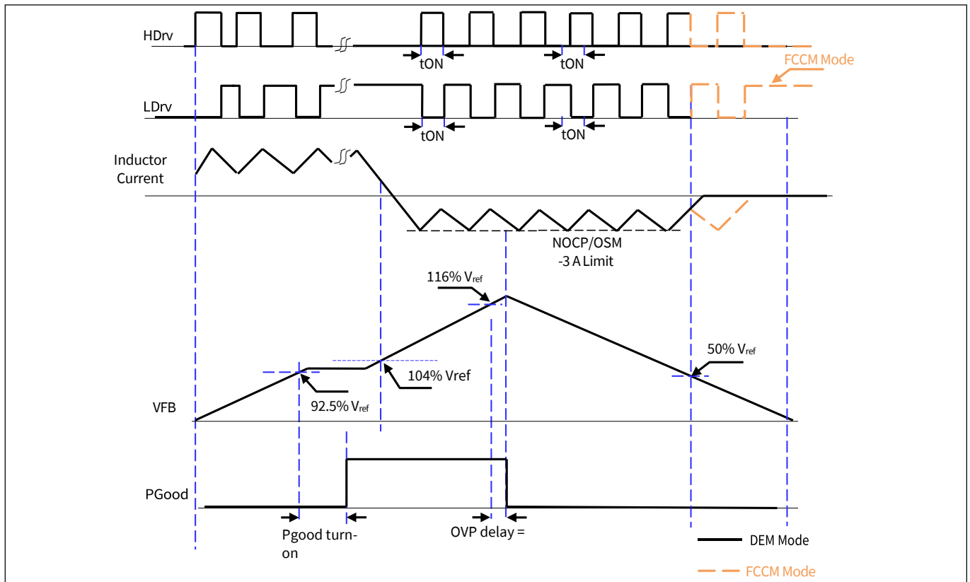
图 8 过电压保护响应和 PGood 性能
