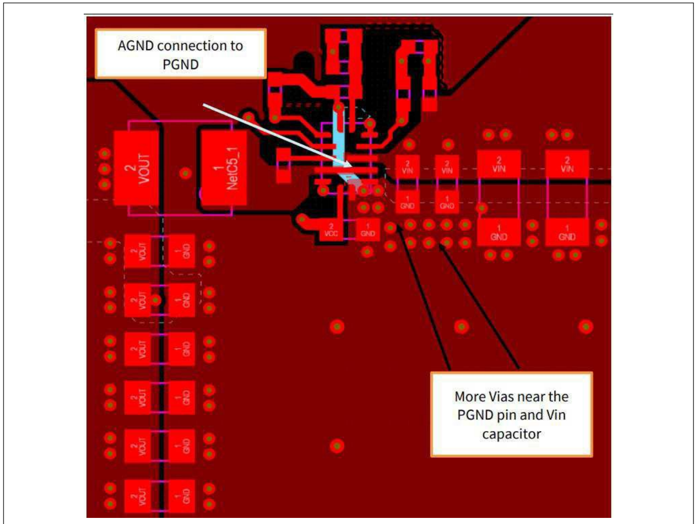
图 9 布局图
