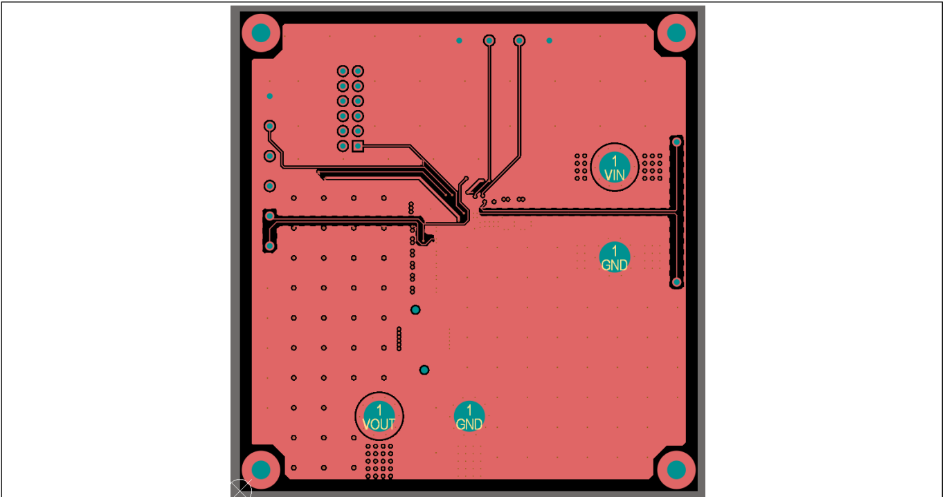
图 13 TDA38807 演示板 - 第 3 层
