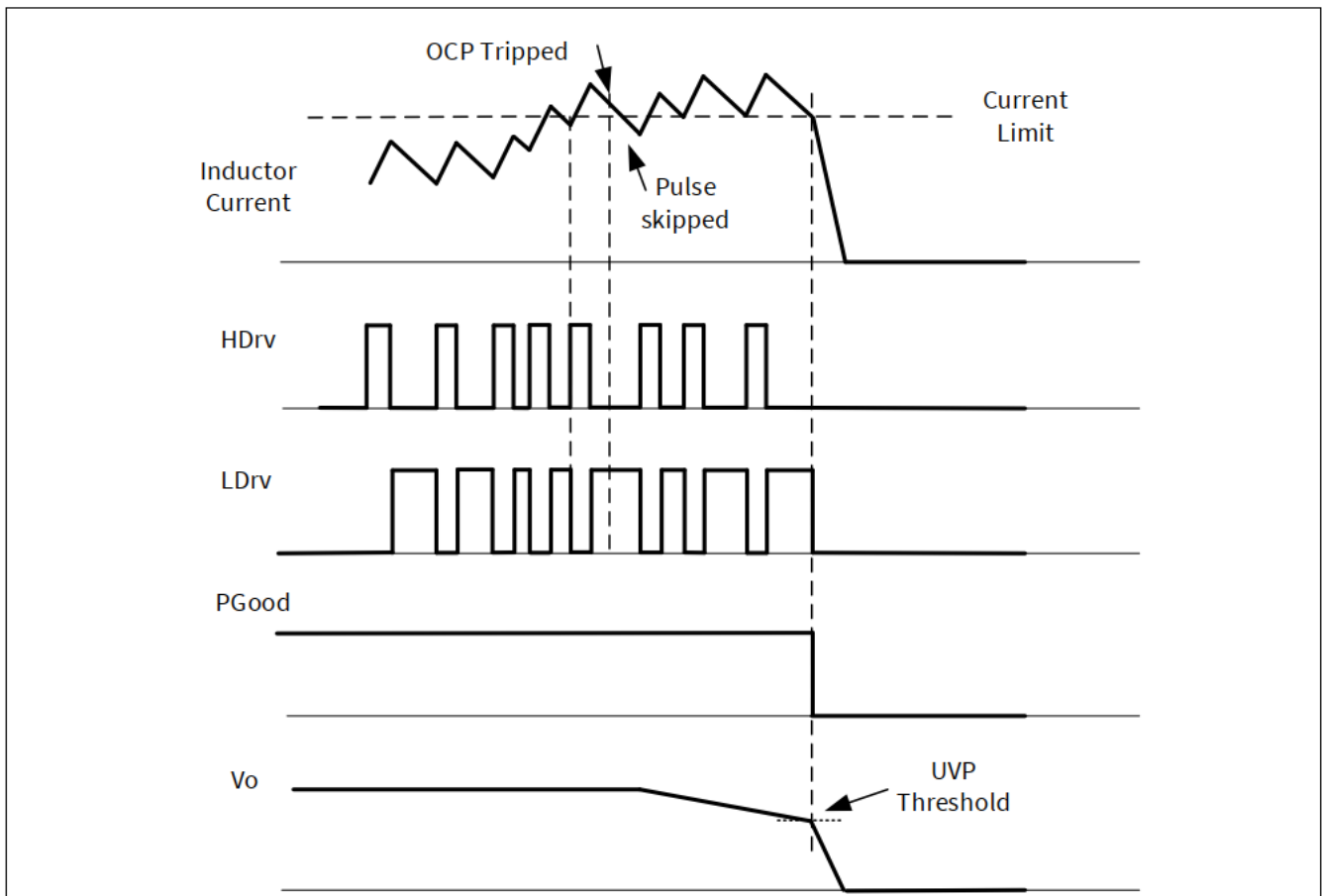
图 7 逐周期 OCP 响应
