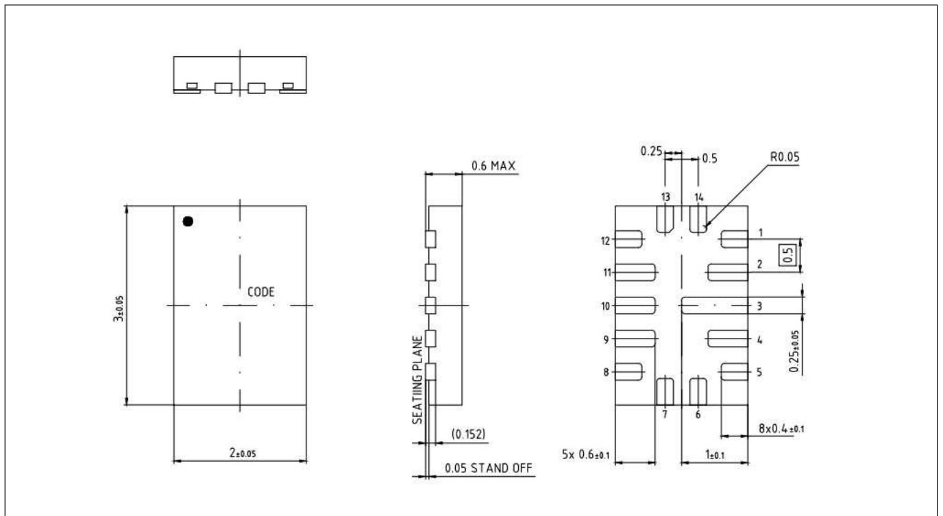
图 16 封装尺寸 (所有尺寸均以毫米为单位)
