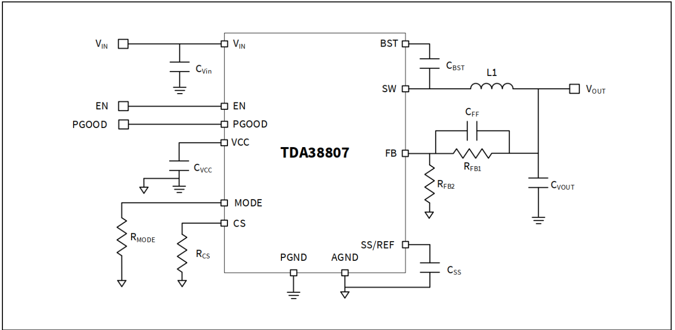
图 3 TDA38807 应用电路
