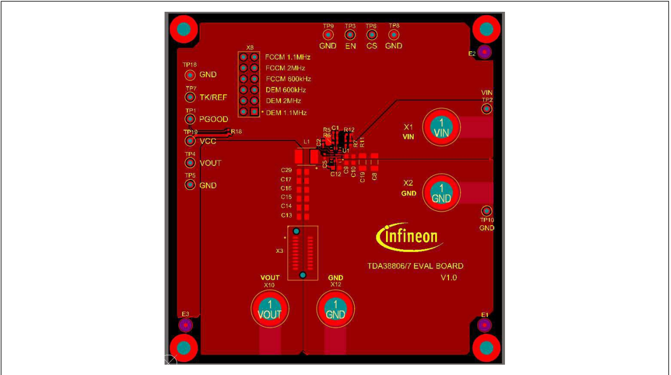
图 10 TDA38807 演示板 - 顶层
