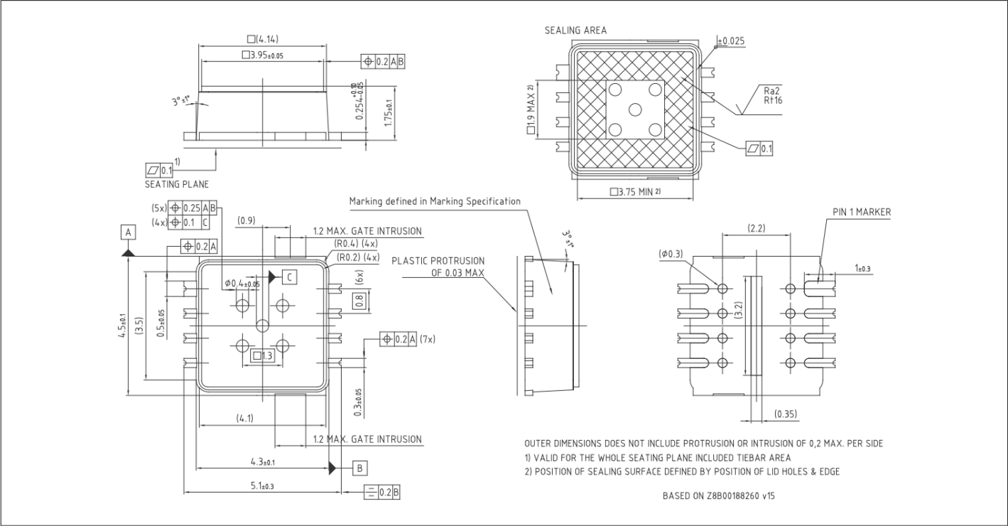
图 41 PG-DFN-8-1 概述
