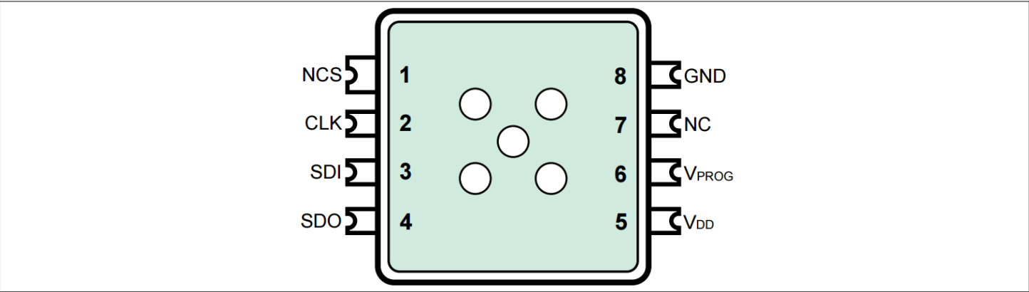
图 2 引脚配置（俯视图，图未按比例绘制）
