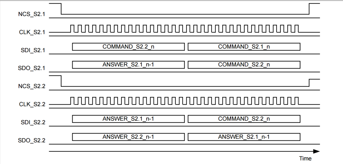
图 35 菊花链信号图示例
