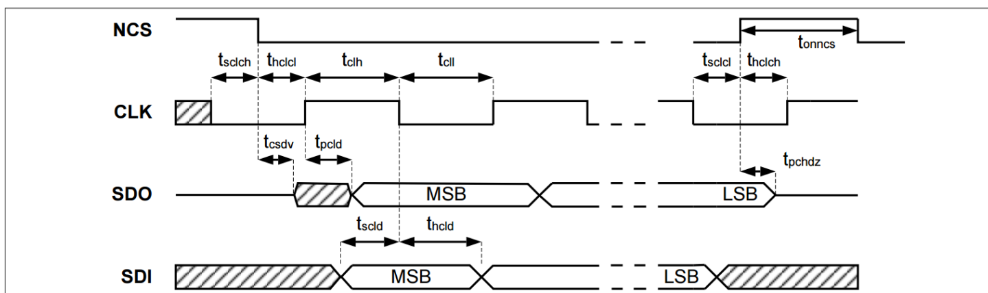
图 6 SPI 时序
