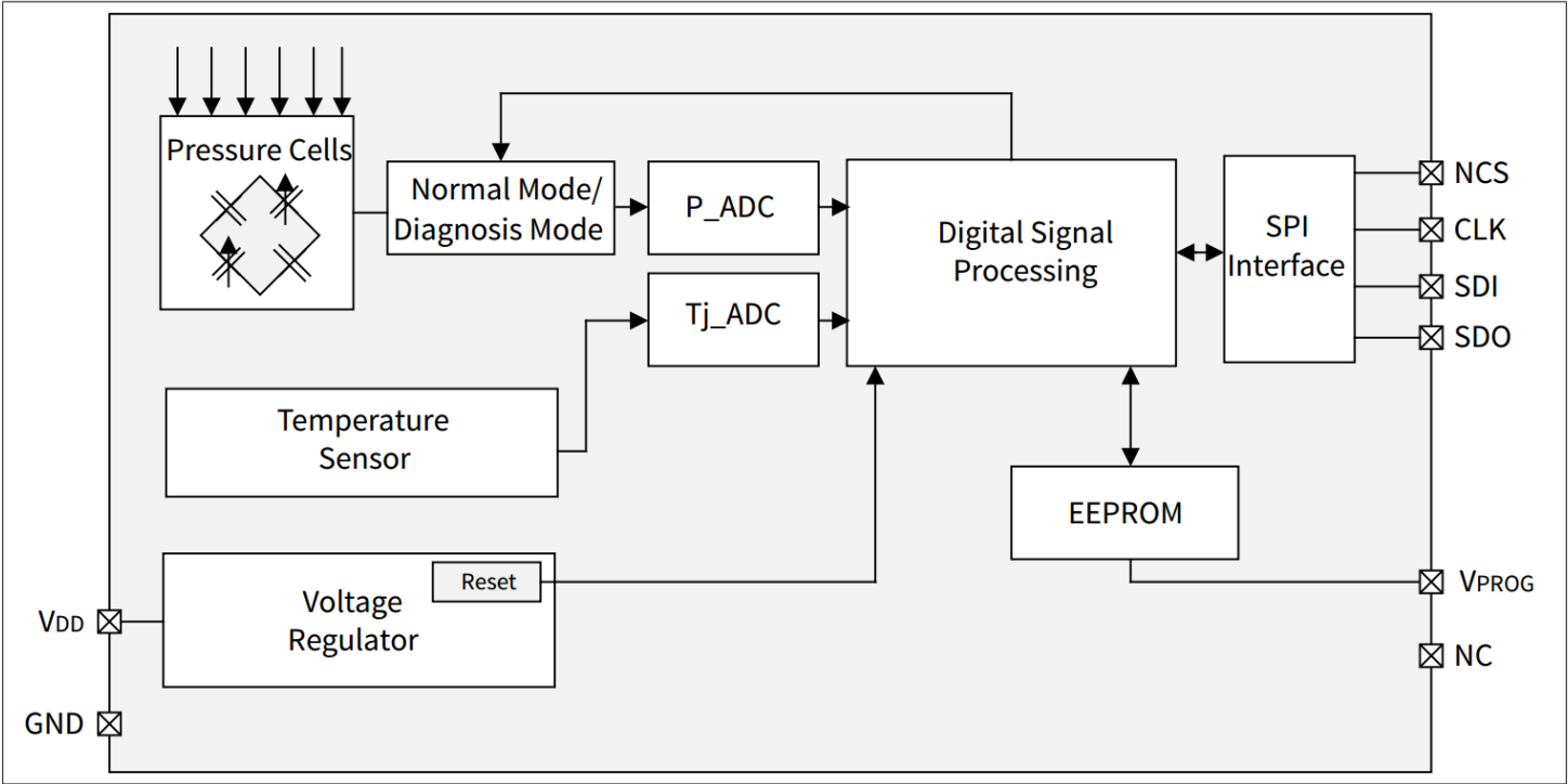
图 1 功能框图
