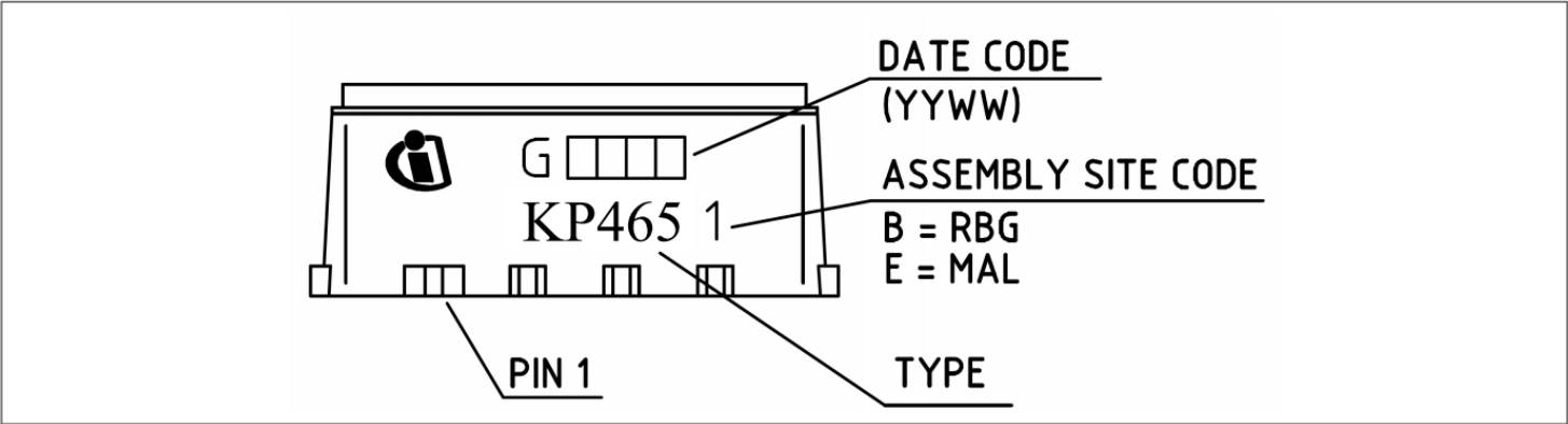
图 43 识别代码
