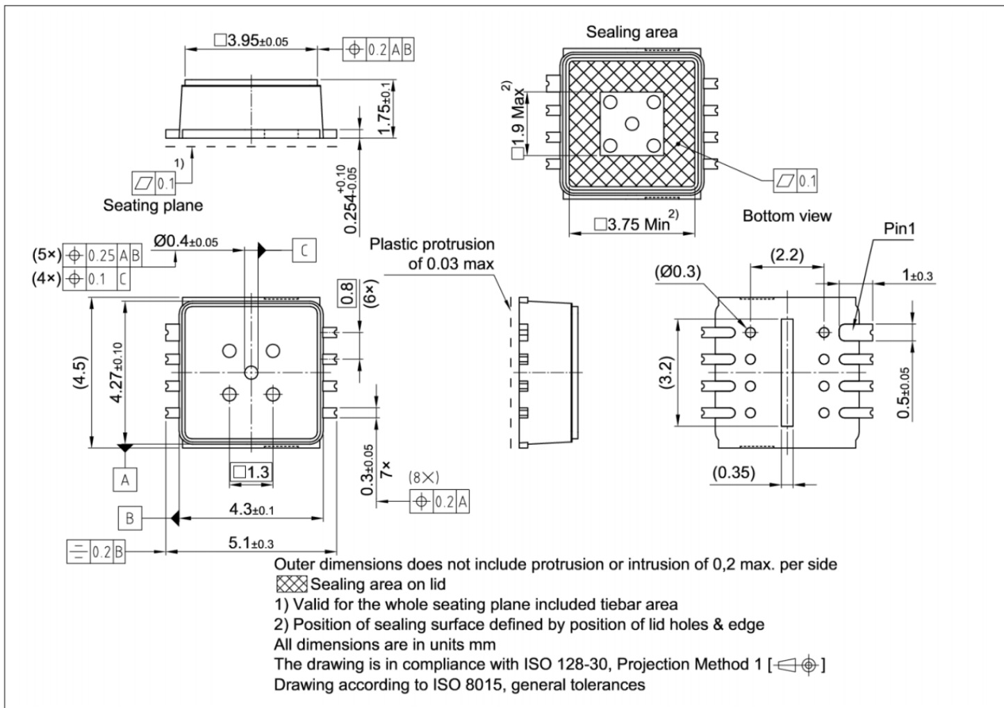
图 41 PG-DFN-8-1 概述
