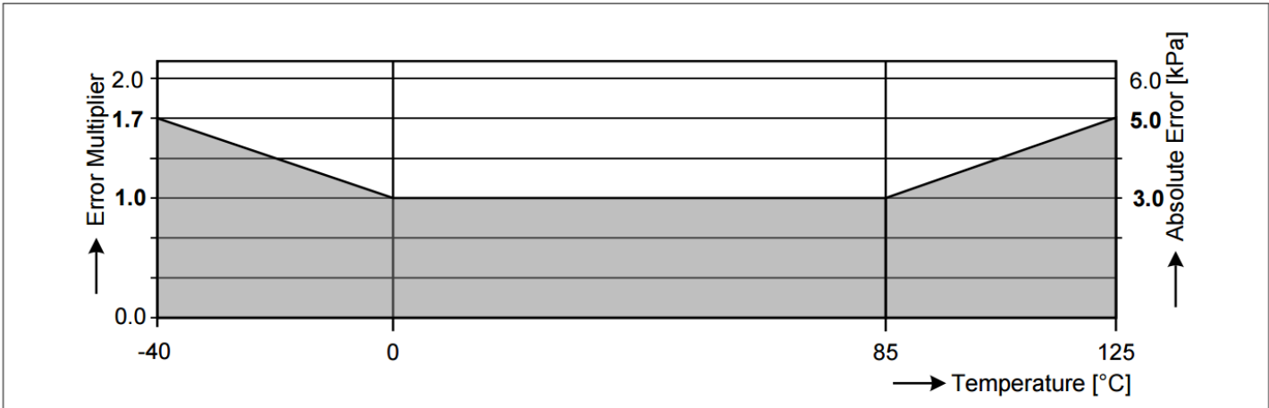
图 4 压力采集精度
