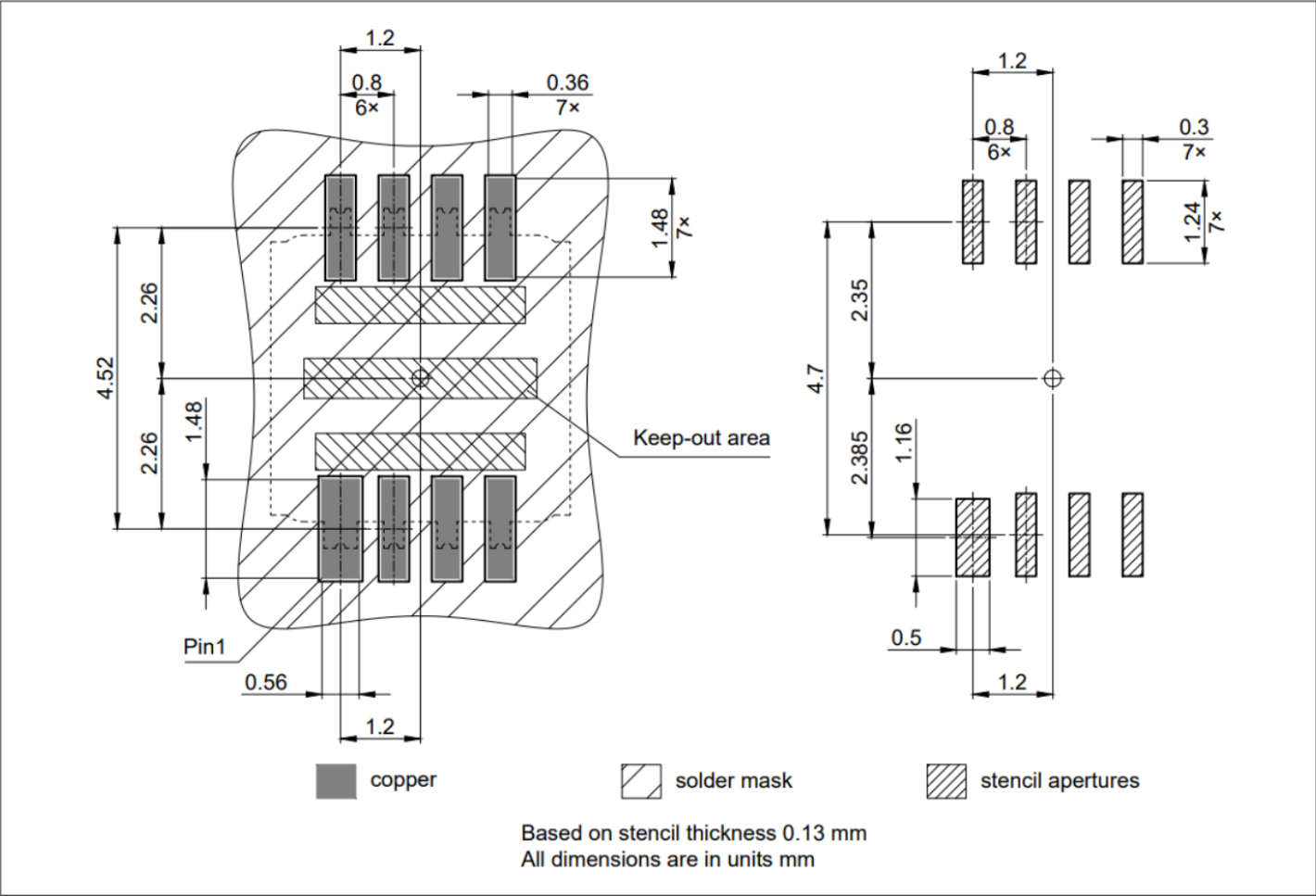
图 42 封装占板图
