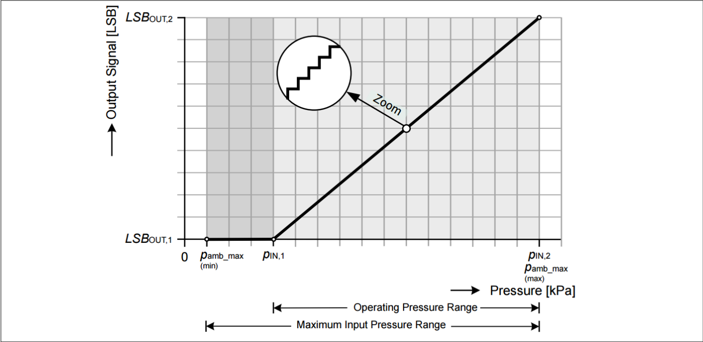
图 3 压力传递函数
