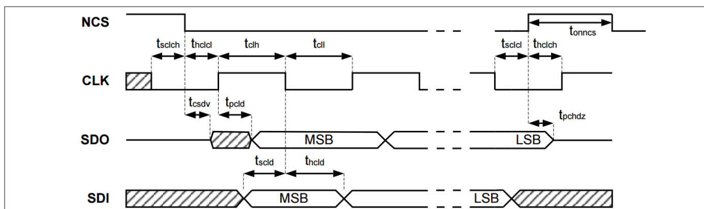
图 6 SPI 时序
