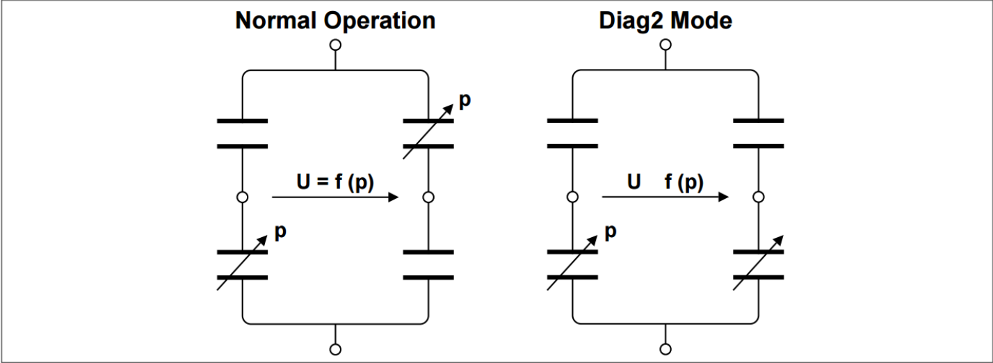
图 39 Diag2 功能
