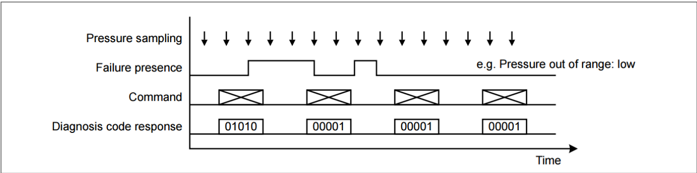
图 36 复位策略示例复位位 C12 = '1'
