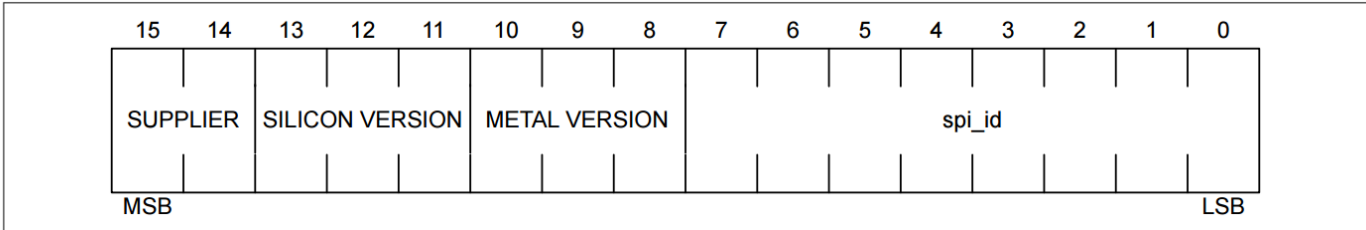
图 11 标识符的 SPI 响应结构
