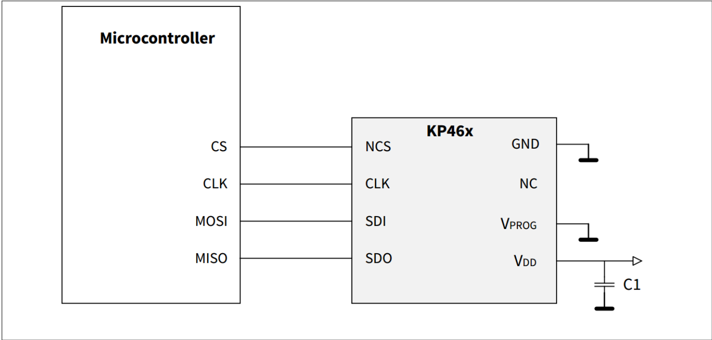
图 40 应用示意图
