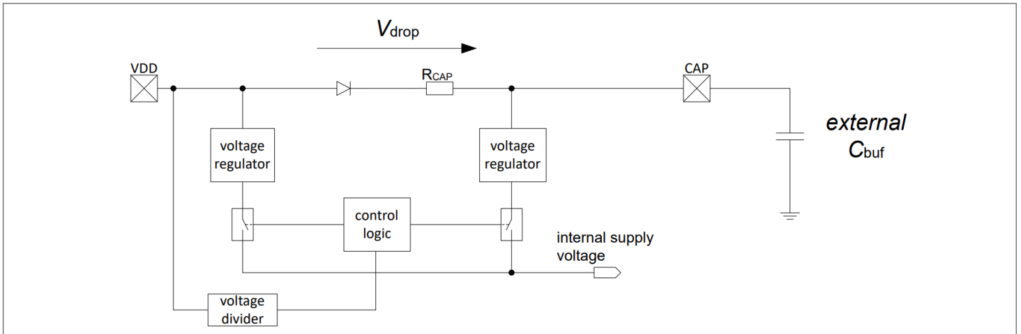
图 18 微断功能的简化框图
