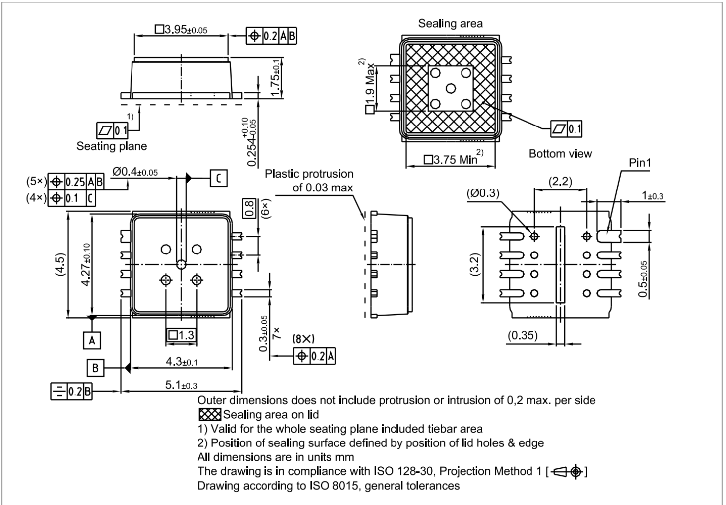
图 21 PG-DFN-8-1 封装外形
