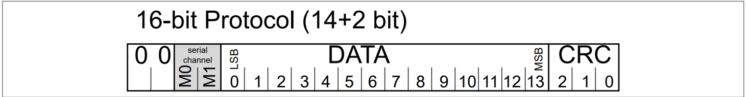
图 10 第 4 阶段的 16 位协议（21 位报文）
