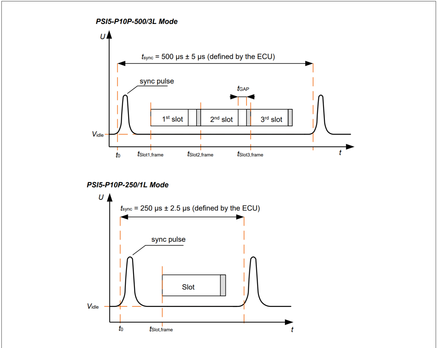
图 3 同步模式下的时序
