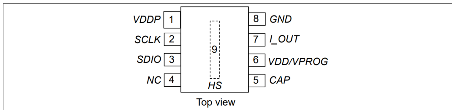
图 1 引脚配置 (PG-DFN-8-1)
