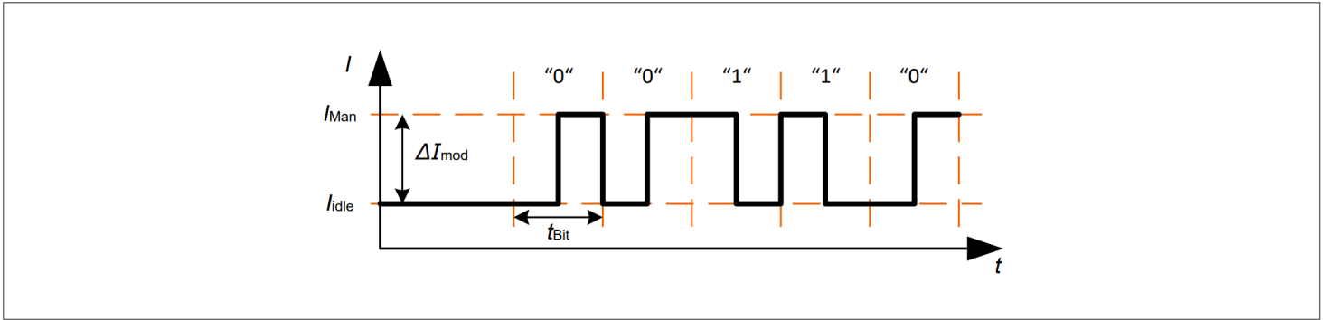
图 2 基于曼彻斯特的电流调制
