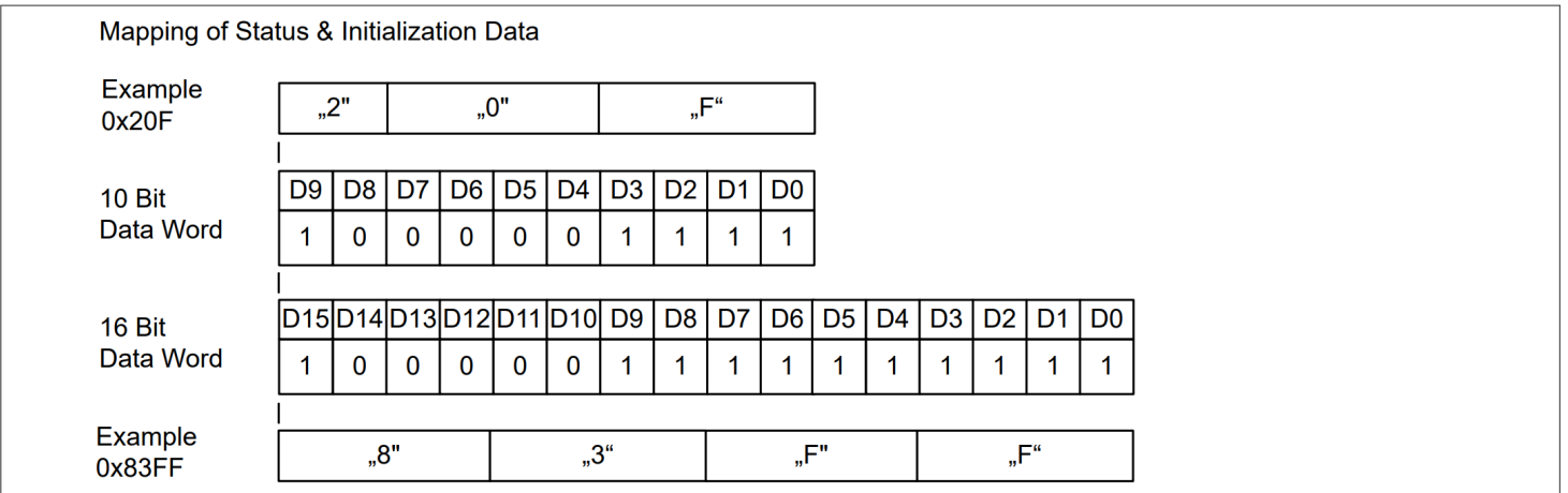
图 13 示例：将状态和初始化数据映射到数据字中
