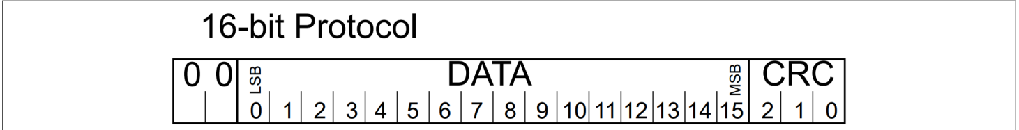
图 12 第 2 和第 3 阶段的 16 位协议 (21 位报文)
