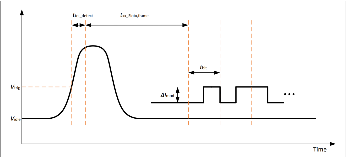
图 4 PS15 插槽时序
