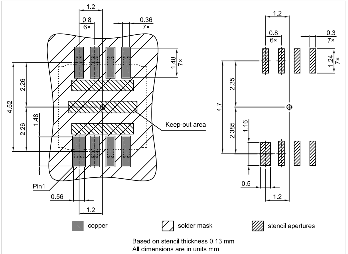
图 22 PG-DFN-8-1 封装尺寸图
