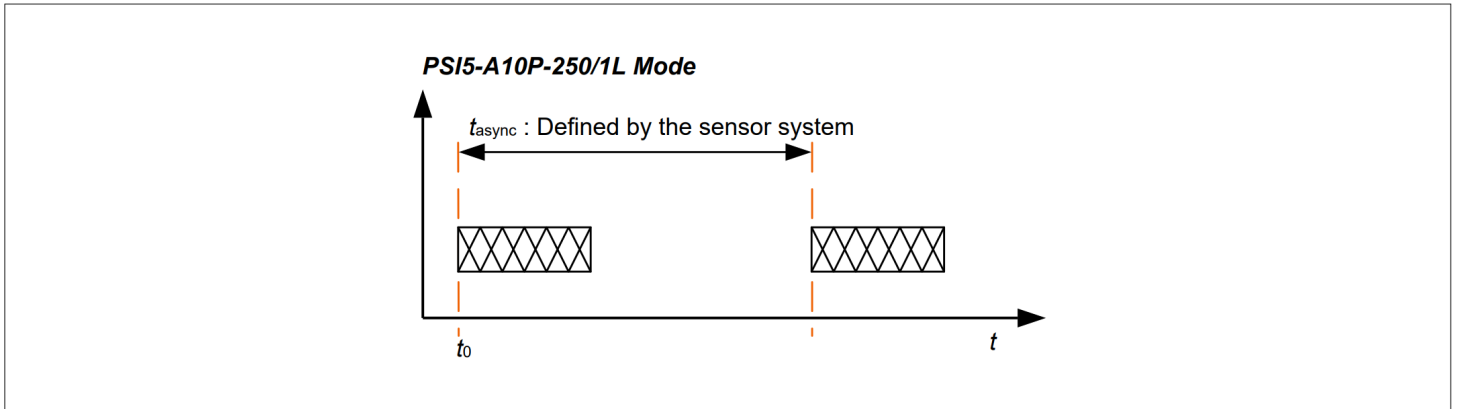
图 7 异步模式下的时序
