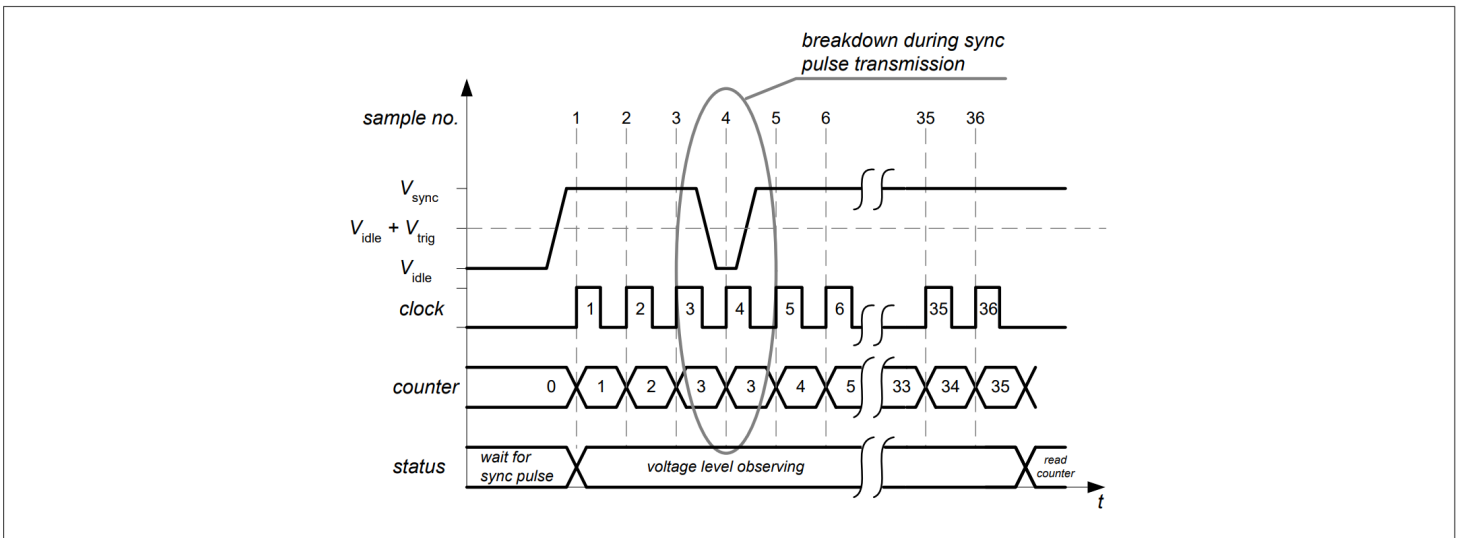
图 5 同步脉冲计数器功能
