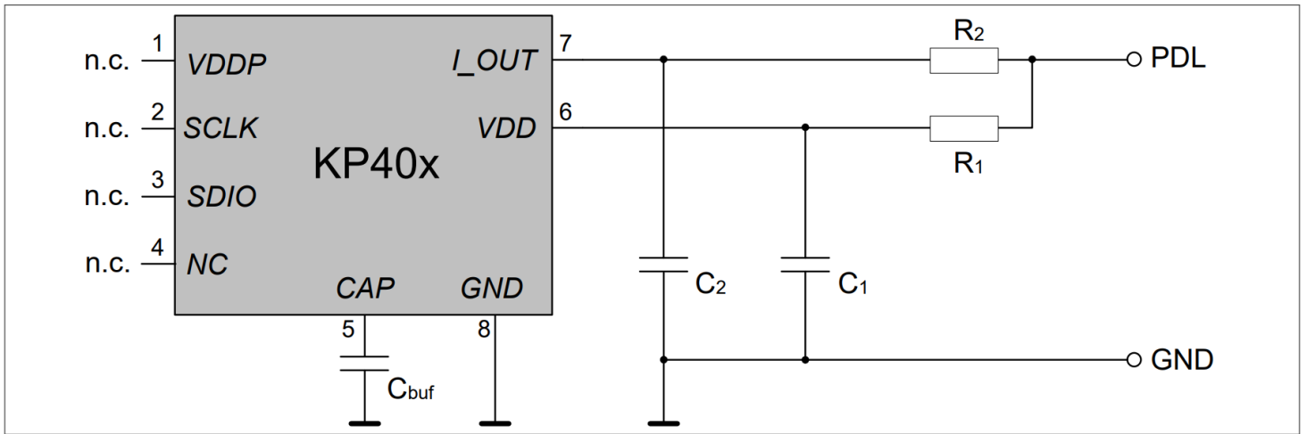
图 20 应用图示例
