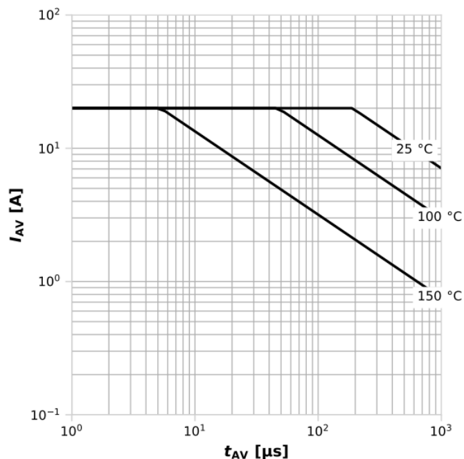
图 13: 典型雪崩特性
