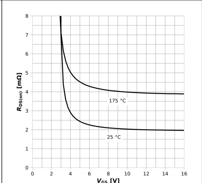
图 8：典型漏源导通电阻
