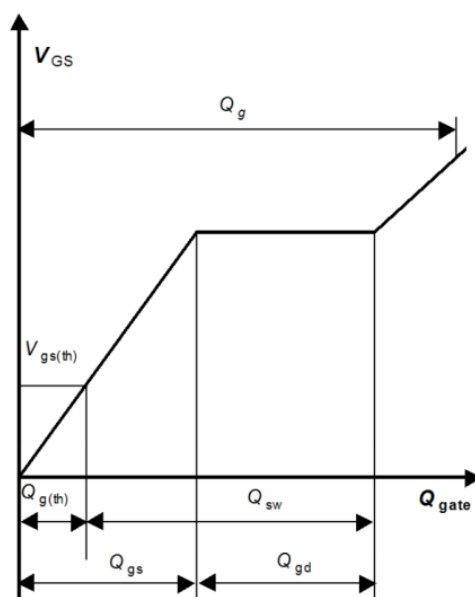
栅极充电波形
