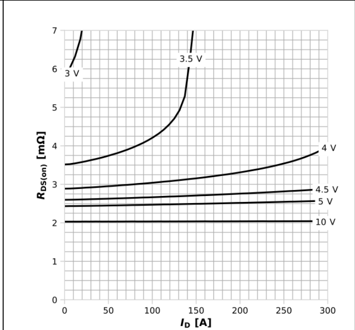
图 6：典型漏源导通电阻
