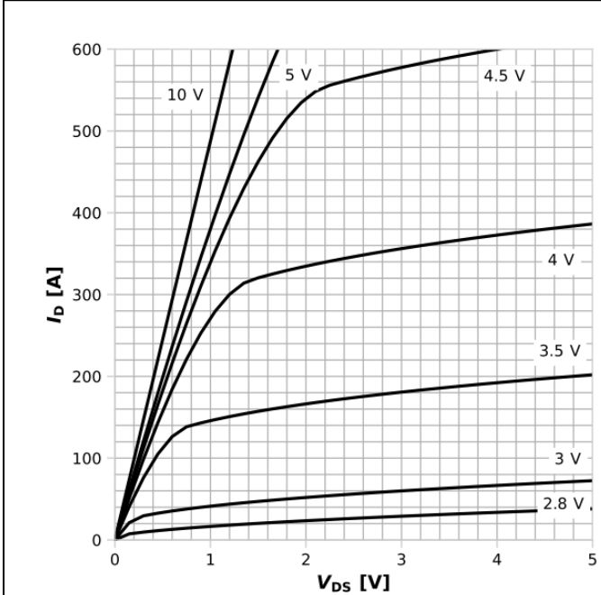
图 5：典型输出特征
