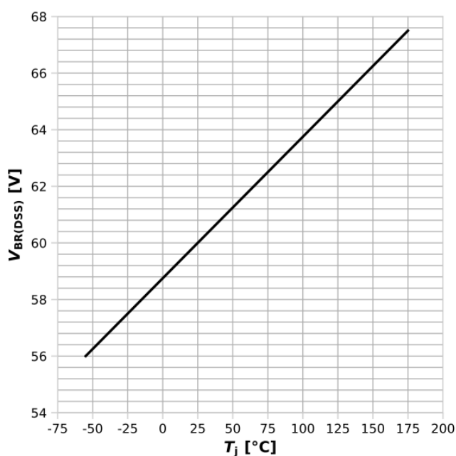
图 15: 最小漏源击穿电压
