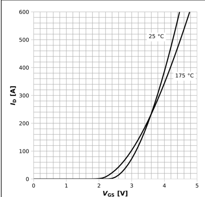
图 7：典型转移特性
