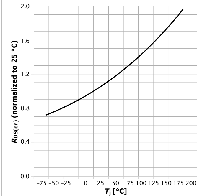
图 9: 典型漏源导通电阻
