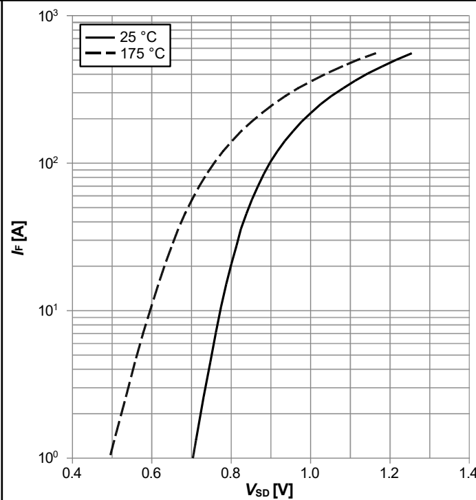
图 12: 典型反向二极管的正向特性
