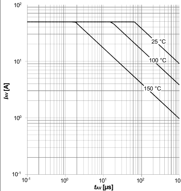
图 13: 雪崩特性
