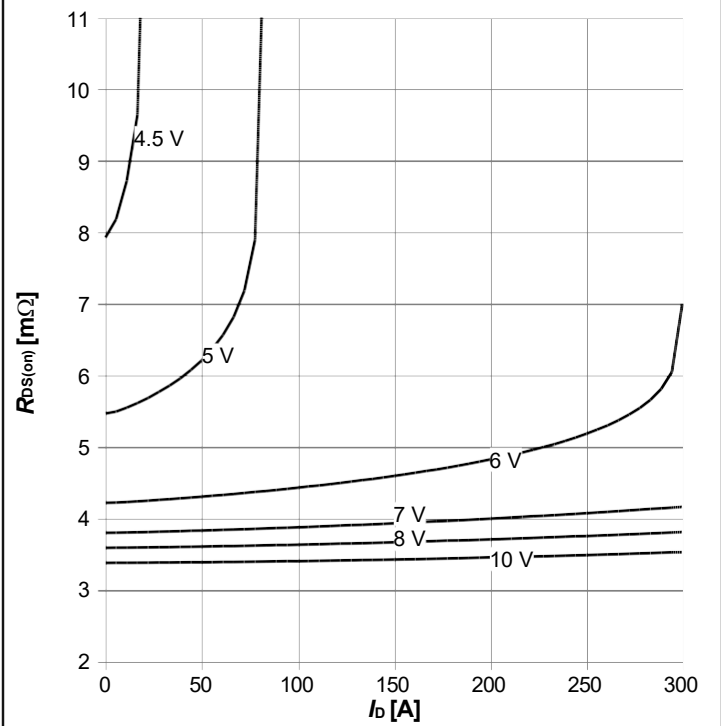
图 6: 典型漏源导通电阻抗
