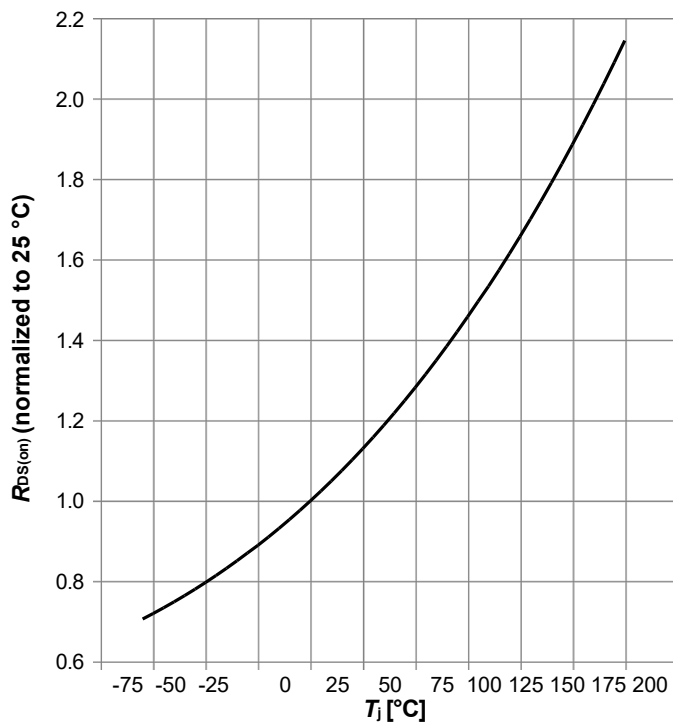
图 9: 归一化漏源导通电阻
