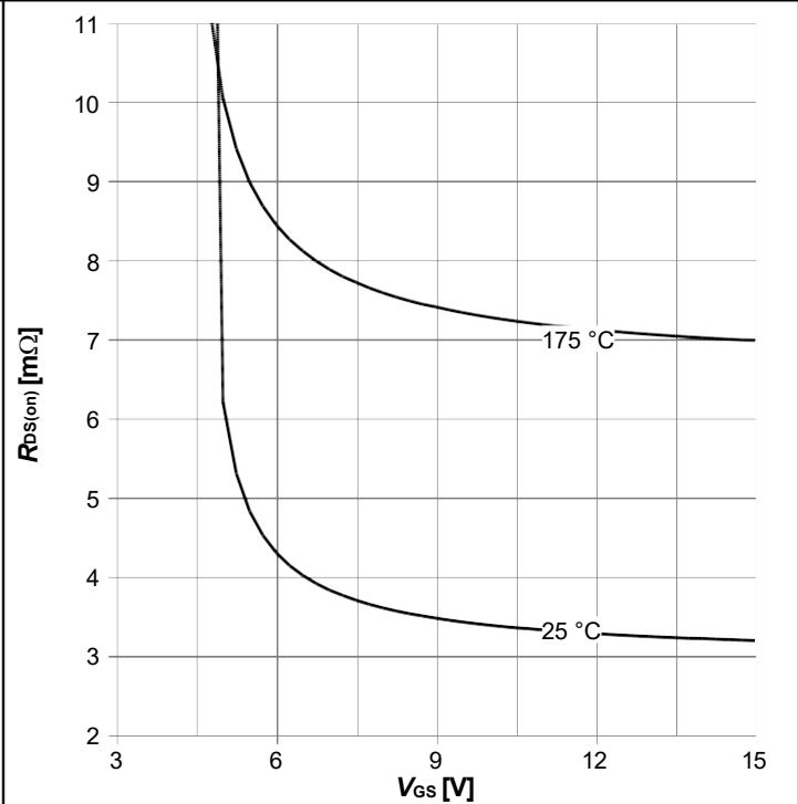
图 8: 典型漏源导通电阻抗
