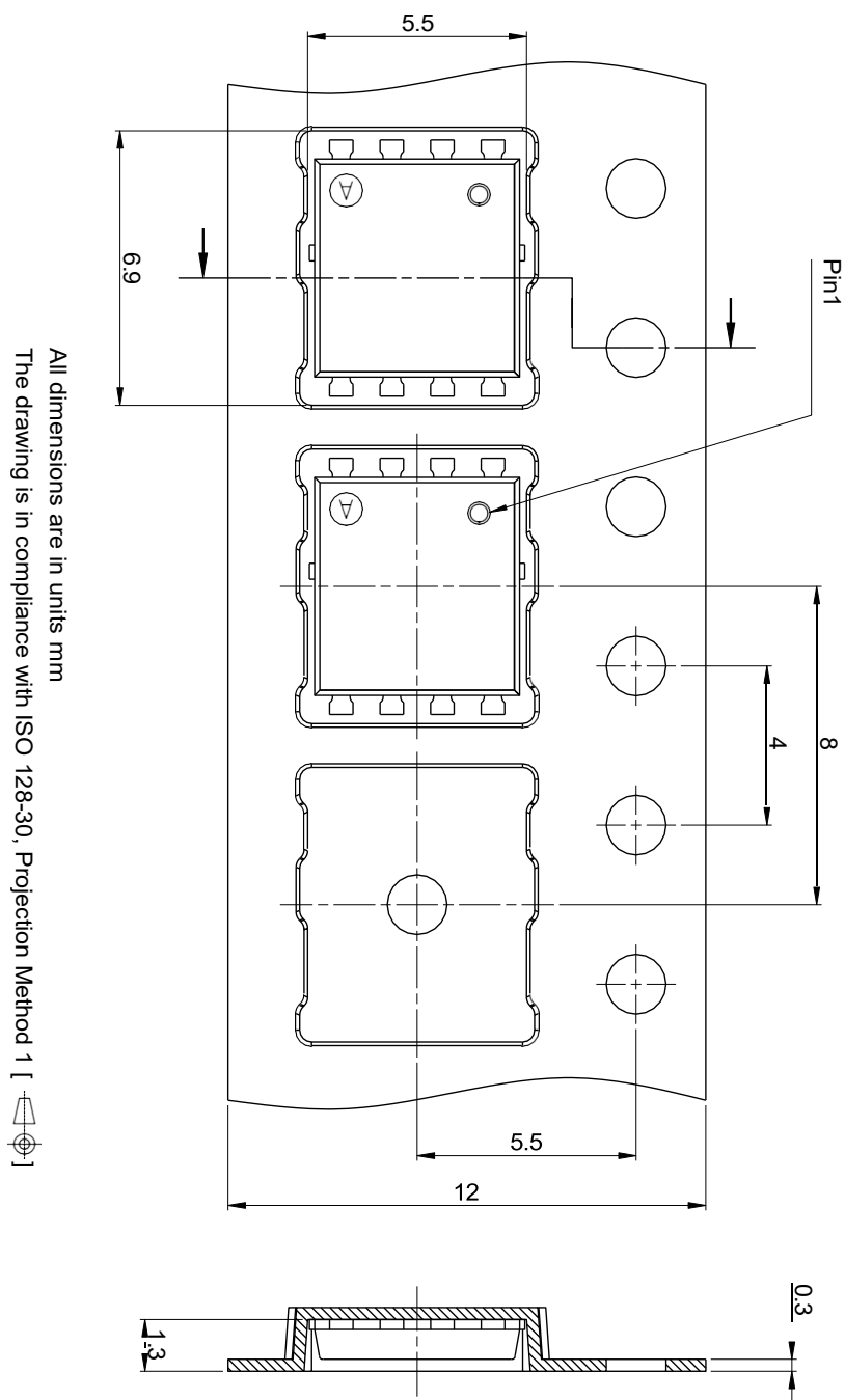
图 3 PG-TDSON-8 外形图，尺寸单位为毫米
