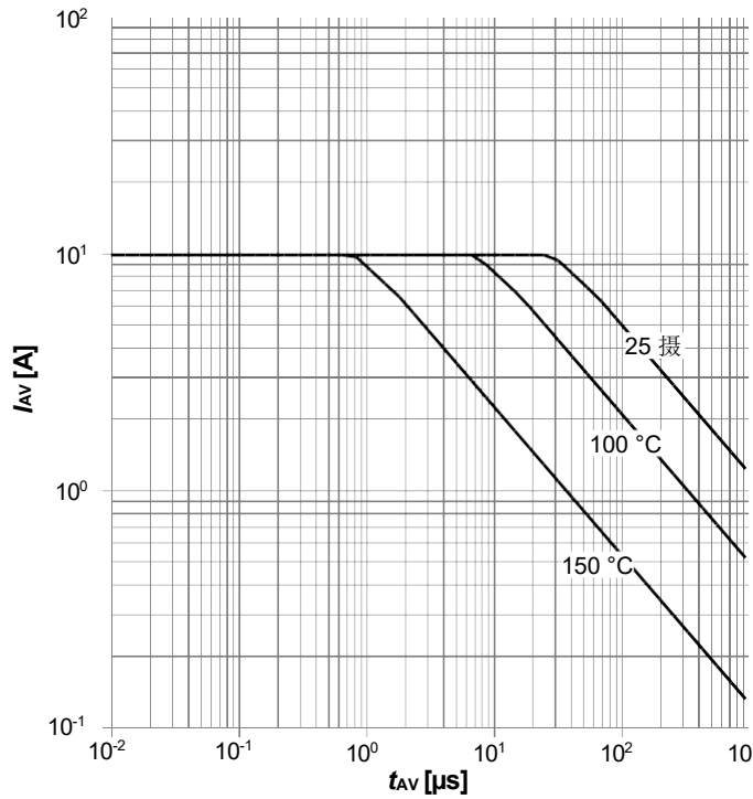
图 13: 雪崩特性
