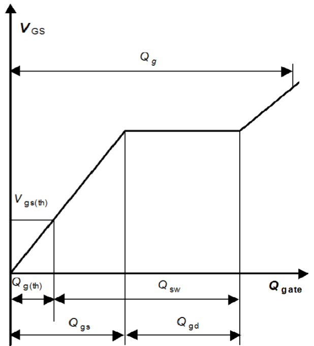
图 栅极充电波形
