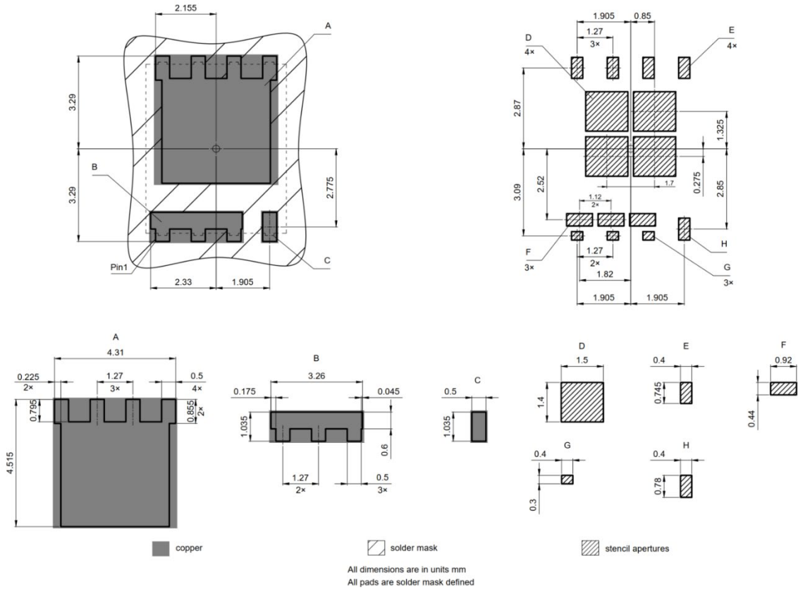
图 2 PG-TDSON-8 外形图，尺寸单位为毫米
