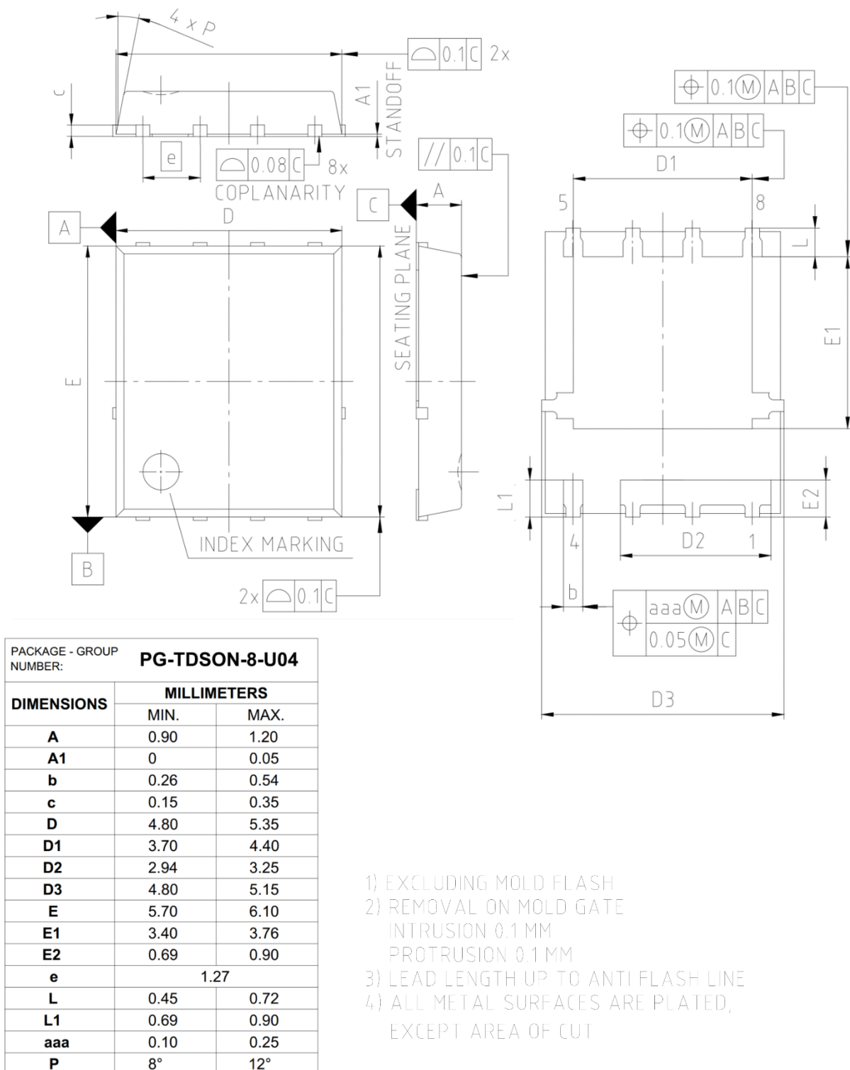
图 1 PG-TDSON-8 外形图，尺寸单位为毫米
