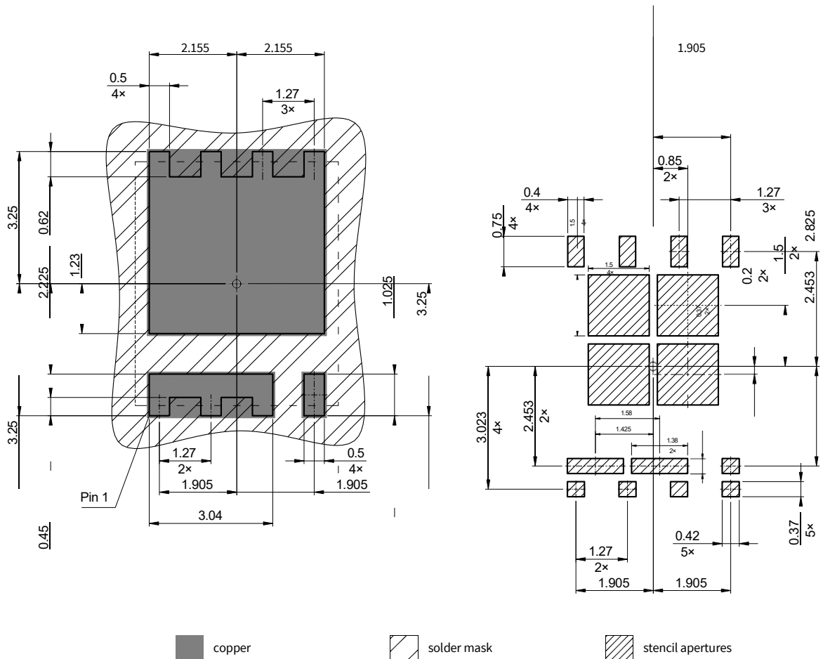
图 2 PG-TDSON-8 封装图, 尺寸单位为毫米
