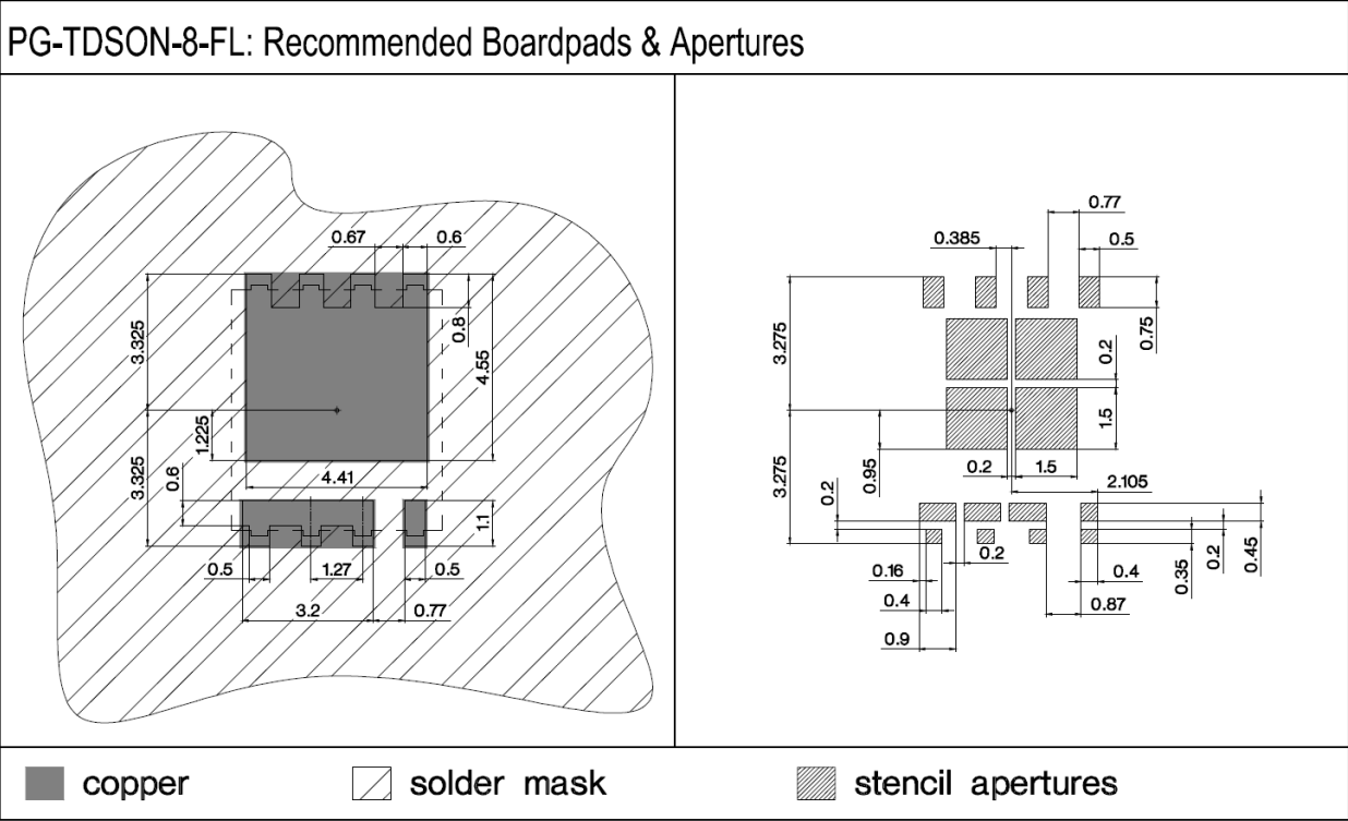
图 2 外形板焊盘 (TDSON-8 FL)
