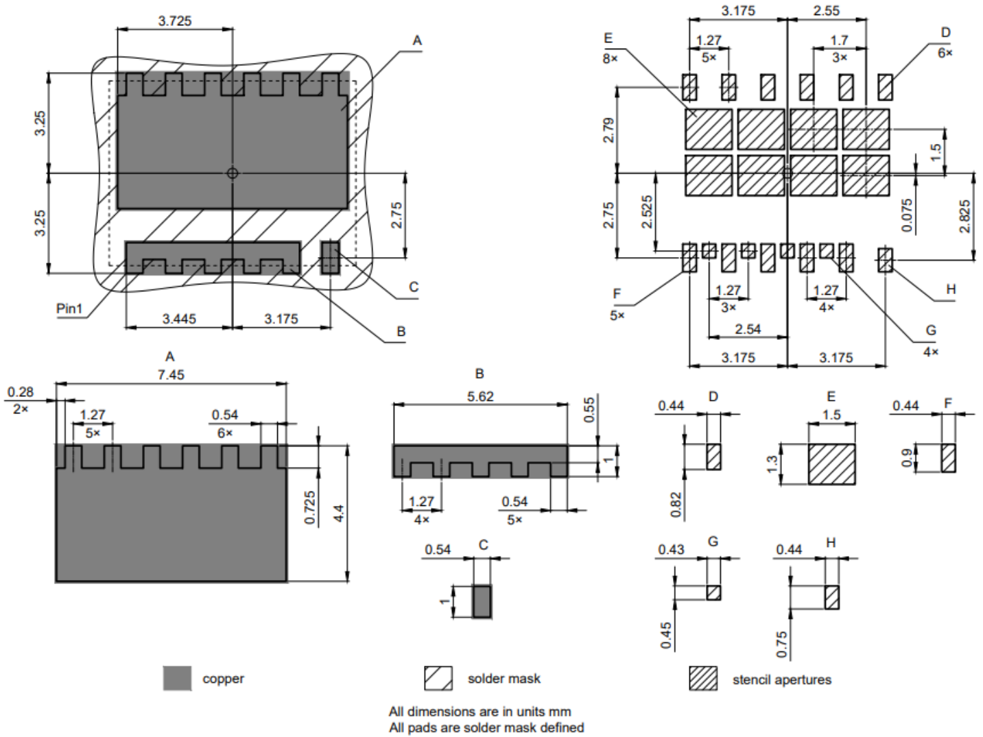
图 2 外形板焊盘 (PG-TSON-12), 尺寸单位为毫米
