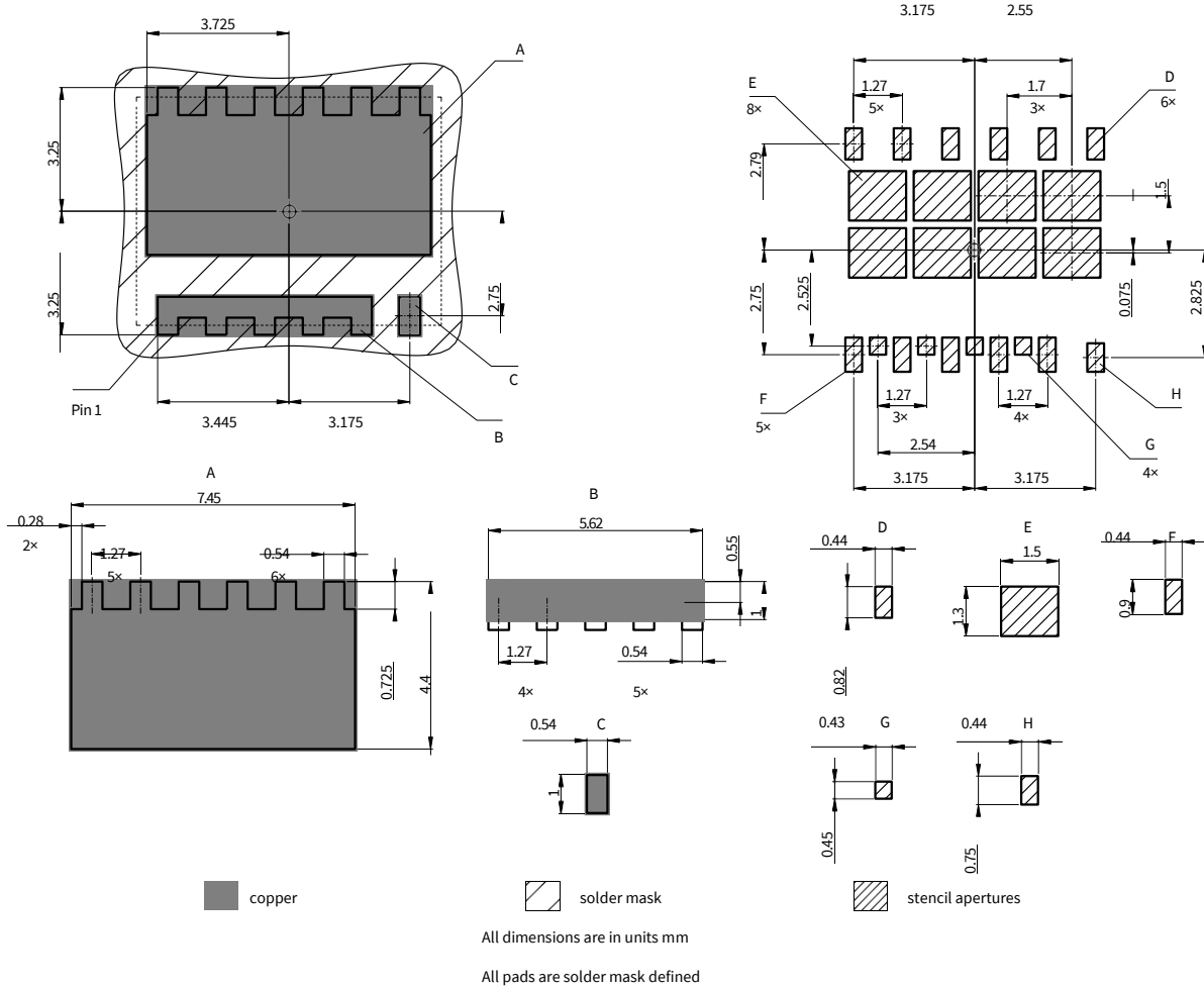
图 2 外形板焊盘 (PG-TSON-12), 尺寸单位为毫米
