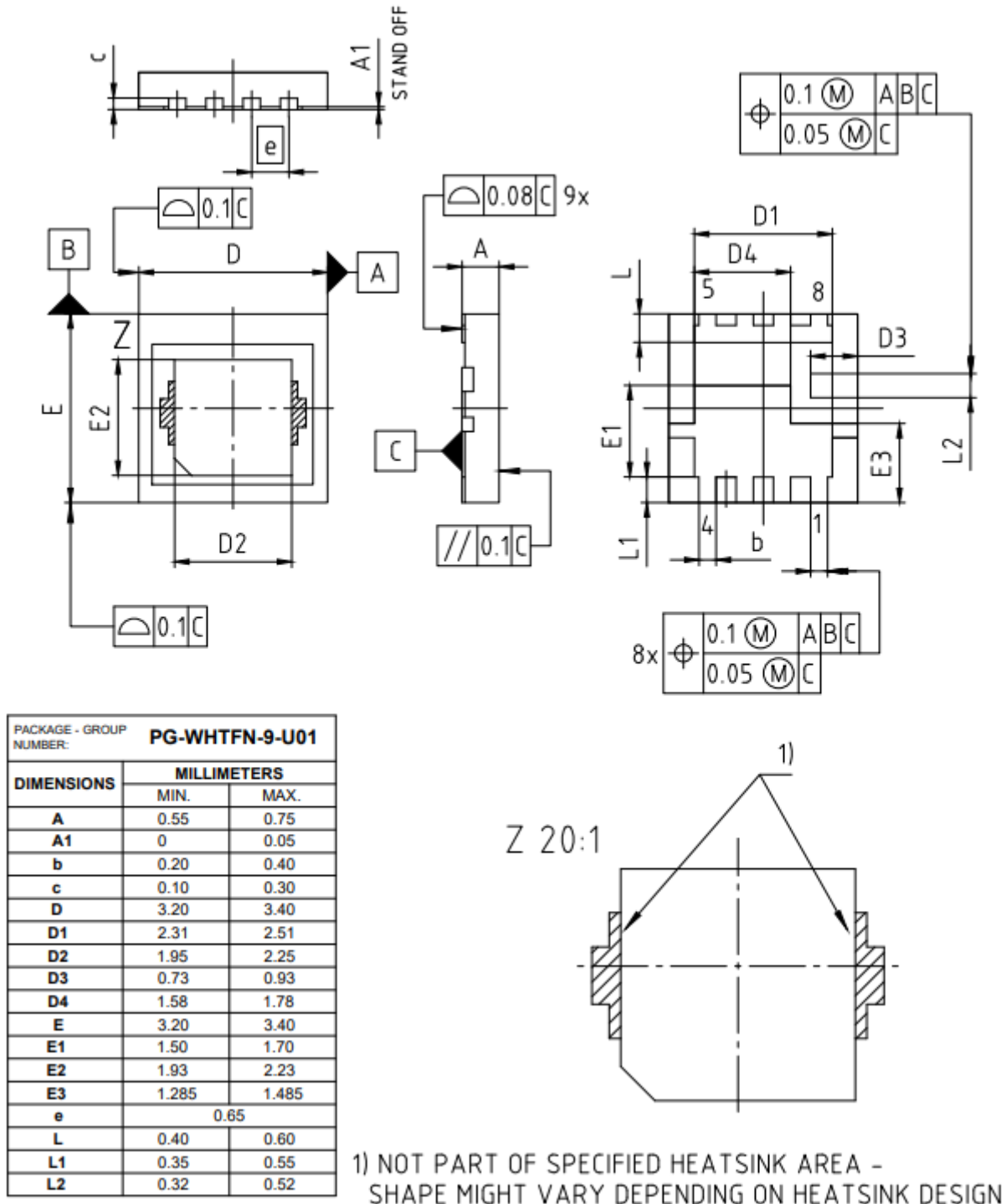
图 1 PG-WHTFN-9 外形图，尺寸单位为毫米
