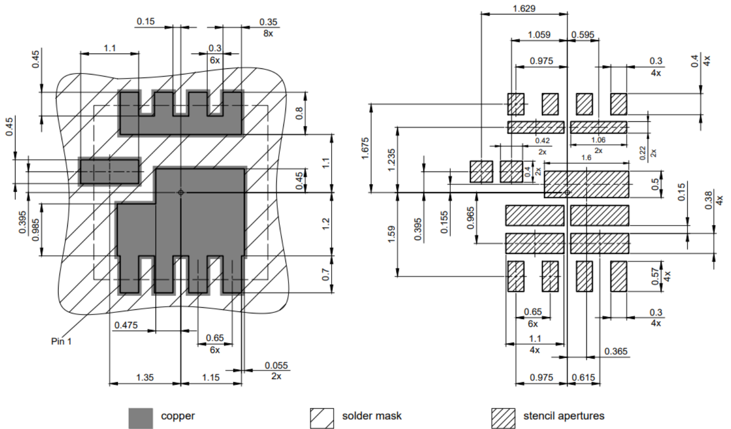
图 2 PG- WHTFN- 9封装图，尺寸单位为毫米
