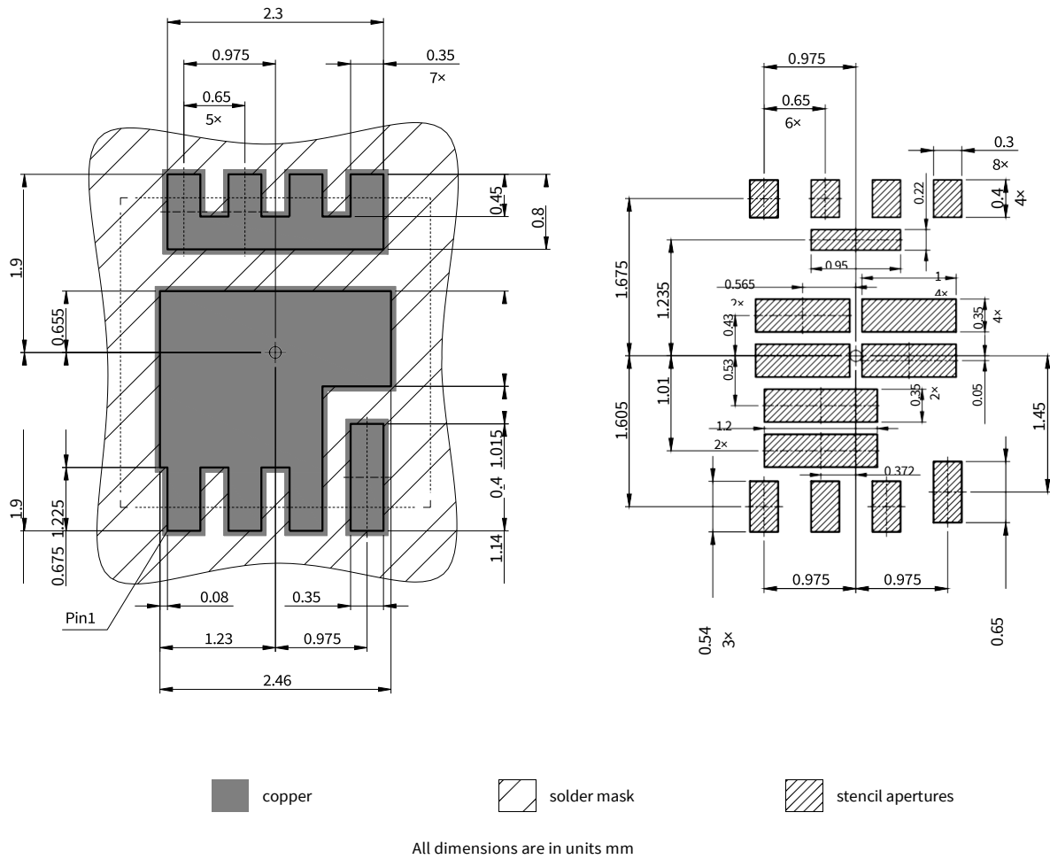
图 2 外形图 (PG-WHSON-8-1)，尺寸单位为毫米
