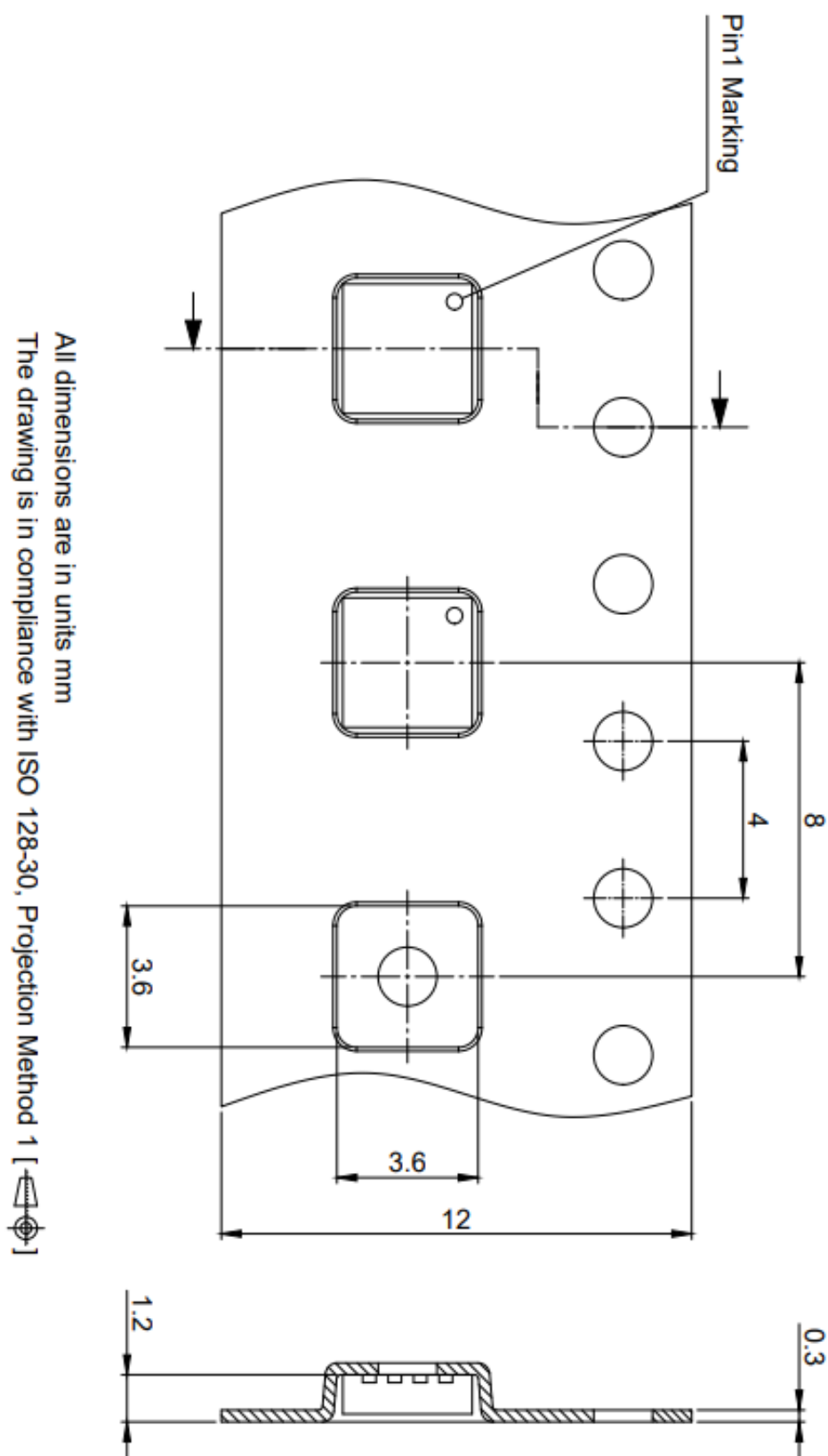
图 3 外形胶带 (PG-WHTFN-9-1), 尺寸单位为毫米
