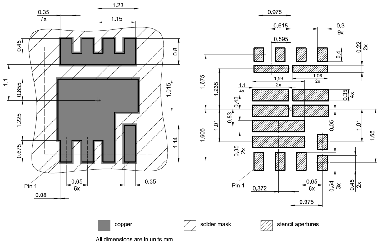
图 2 外形板焊盘 (PG-TSON-8-4)
