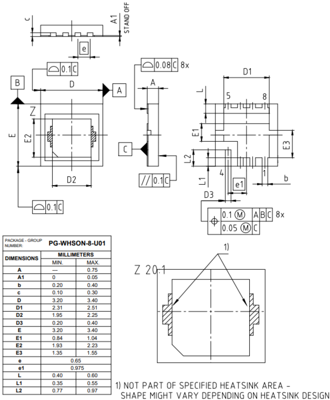
图 1 PG-WHSON-8 外形图，尺寸单位为毫米
